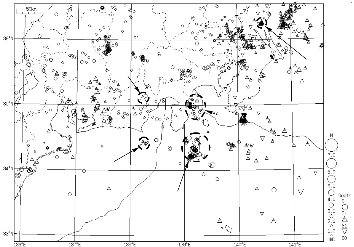
図1 震央分布図
