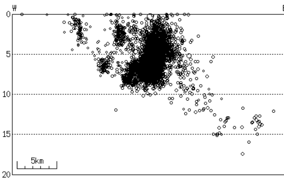
図 3 東西断面図
