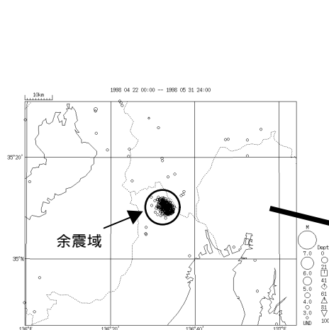
図 3 震央分布図
