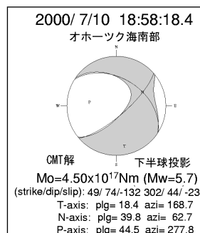
図3-1 発震機構
