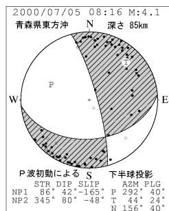
図 4－1 発震機構
