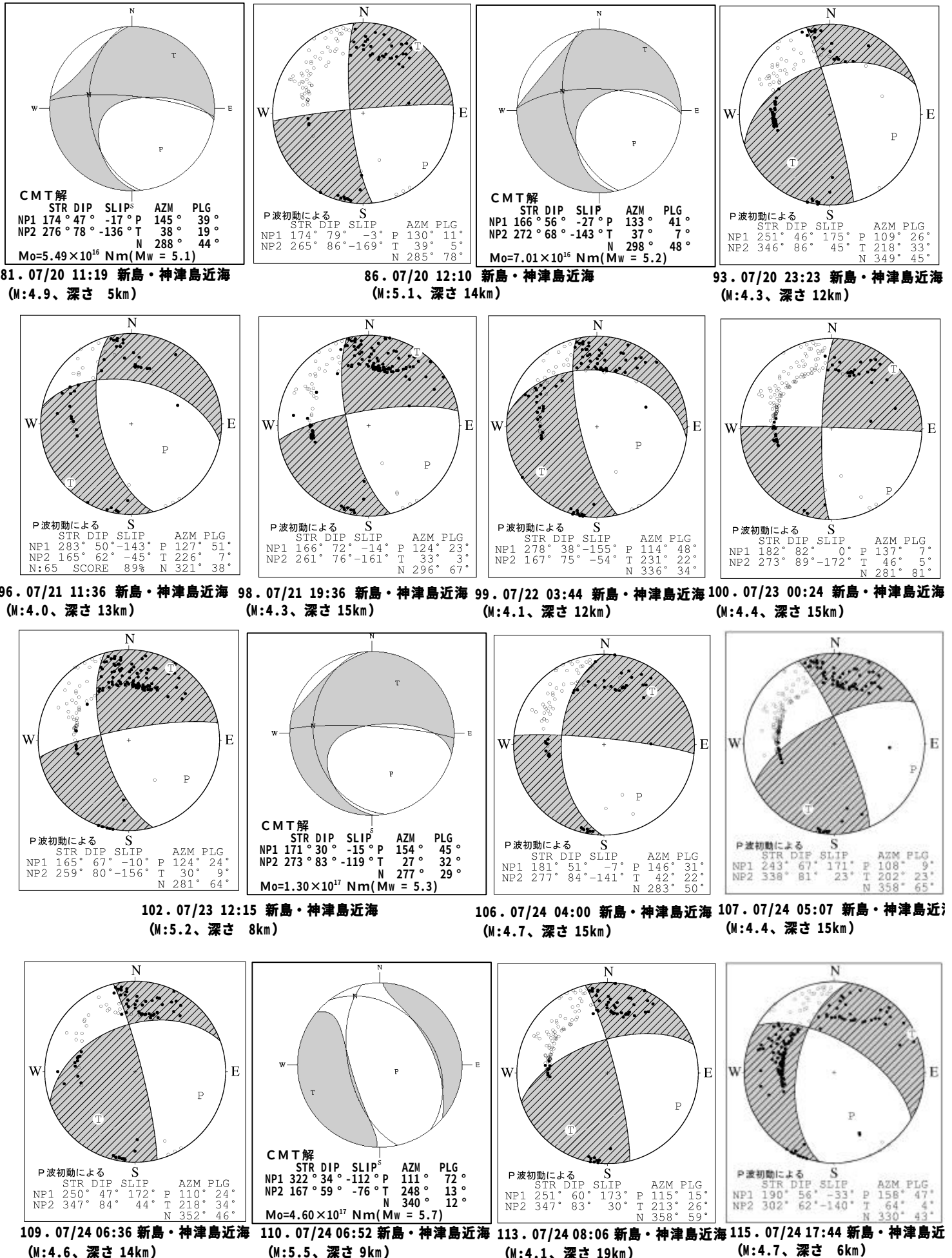
図 3 - 2 - 4 発震機構 <図の数字は、表 1 の番号に対応する>
