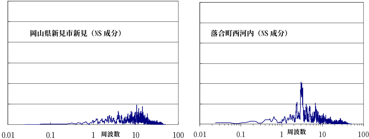
図 1－3 鳥取県西部地震の周波数解析（内陸部） 縦軸の 1 マスは、図 1－2－3 と同じである。
