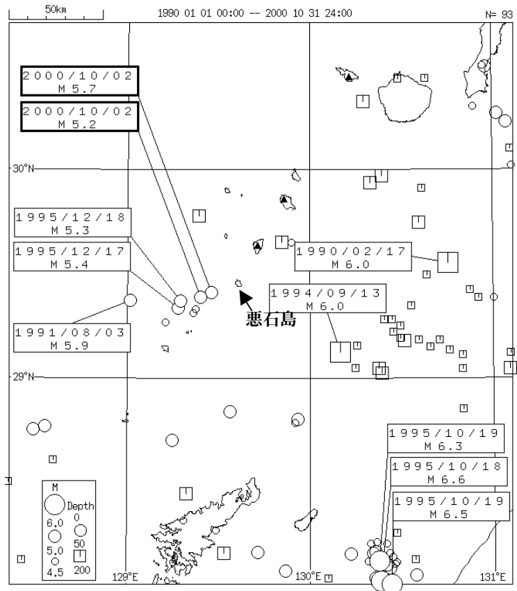
図1 今回の地震と最近の地震活動（M≥4.5）
