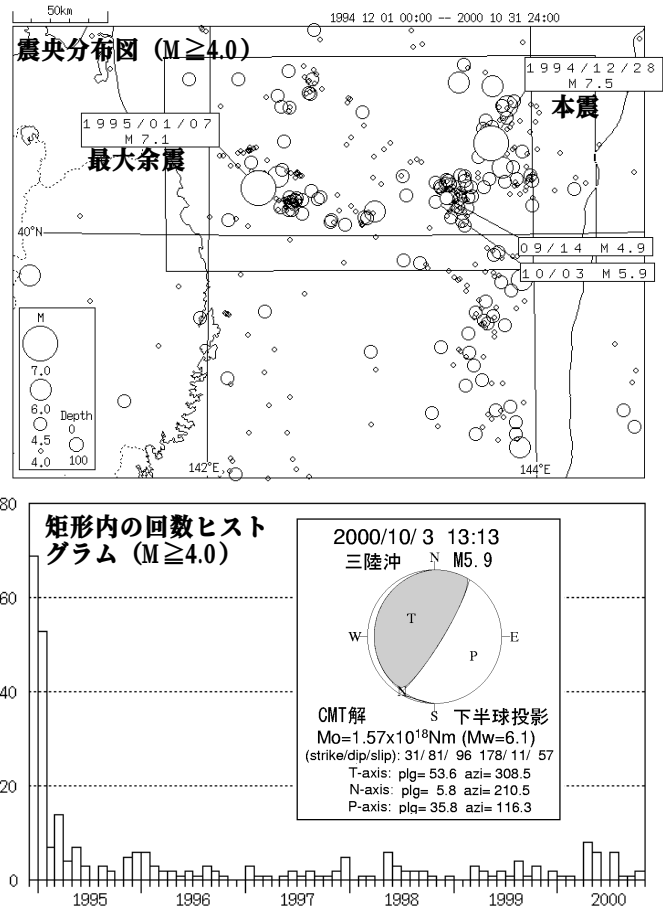
図4-1 三陸沖の地震活動 表示期間：1994年12月～2000年10月
