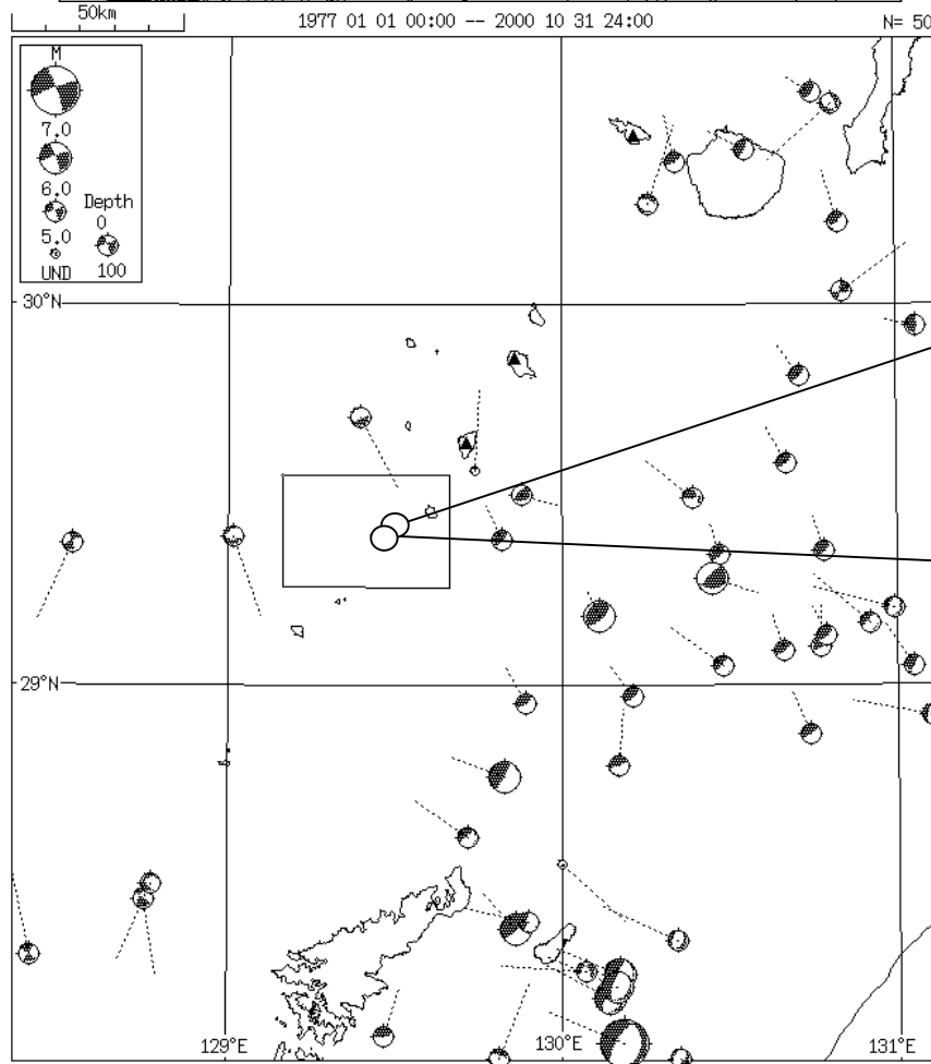
図4 過去の地震のCMT解（ハーバード大学による）と今回の地震のCMT解（気象庁）
