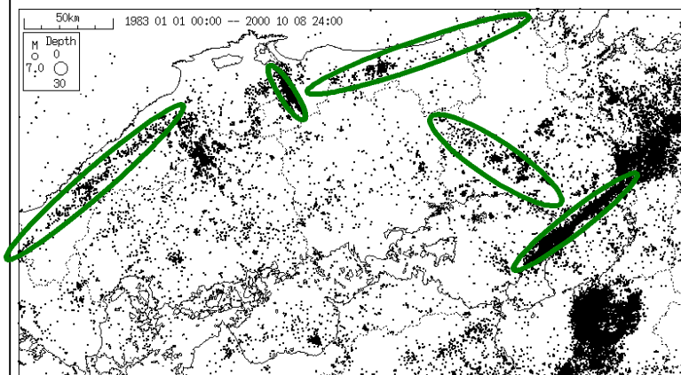
図3 中国地方の震央分布
