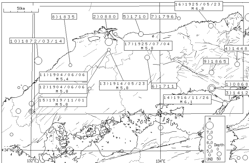
図3-1-1 過去の被害地震 （～1925年）
