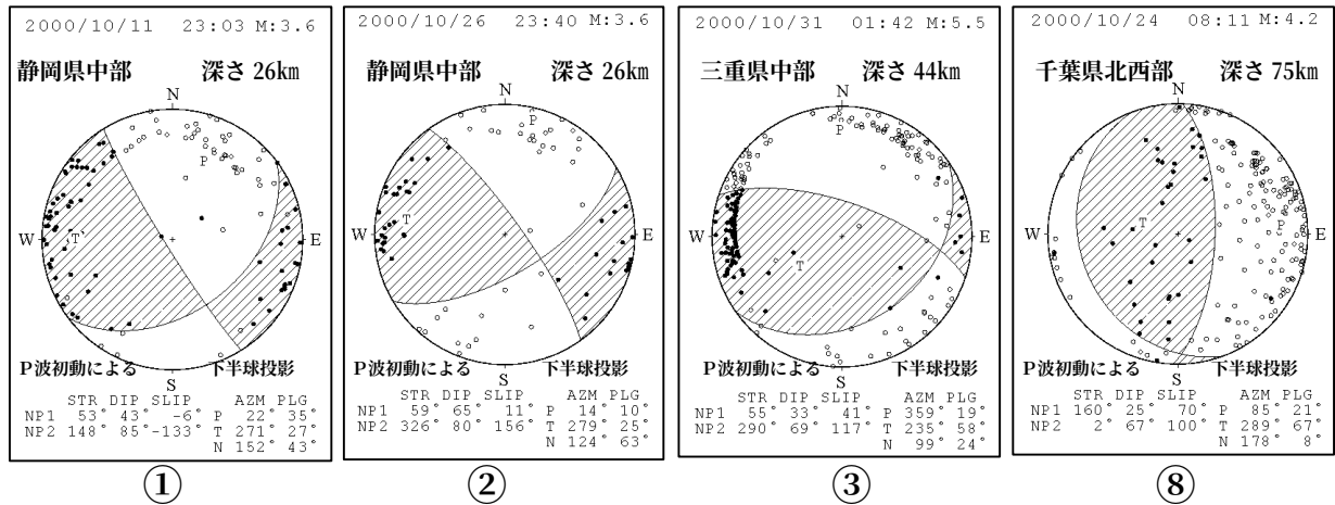
図3 主なP波初動による発震機構＜図中の数字は、本文中の番号に対応する＞
