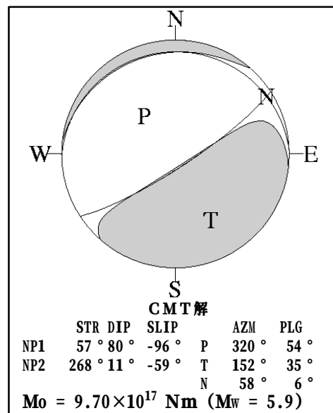
3. 10/02 16:44 奄美大島近海 (M:5.7、深さ 30km) 北北西—南南東方向に張力軸を持つ正断層型
