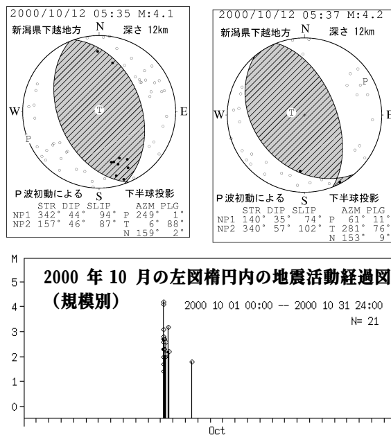
図 5-2 新潟県下越地方の地震活動
