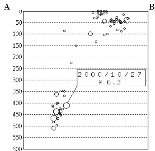
図 5-4 父島近海の地震活動
