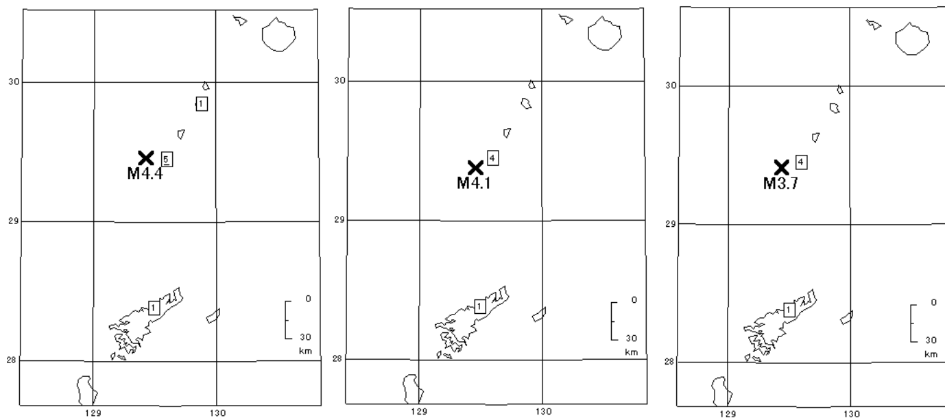
4. 10/02 17:04 奄美大島近海 (M:4.4、深さ 25km)
