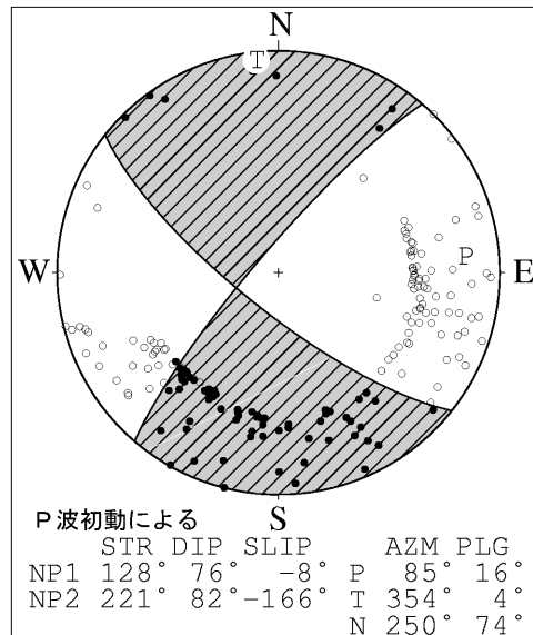
6. 10/06 13:30 鳥取県西部 (M:7.3、深さ 11km) 東西方向に圧力軸を持つ横ずれ断層型
