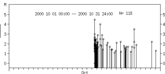
図 5-3 栃木県北部の地震活動
