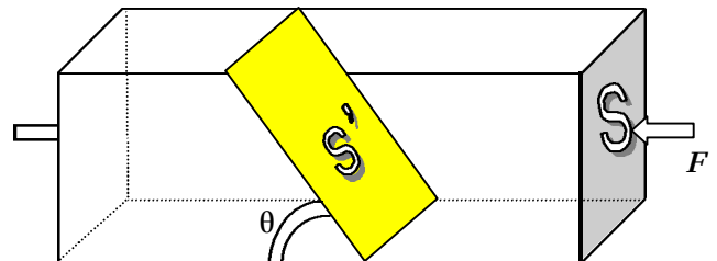
図2 岩石破壊実験(上)と破壊面に掛かる力の模式図(下)
