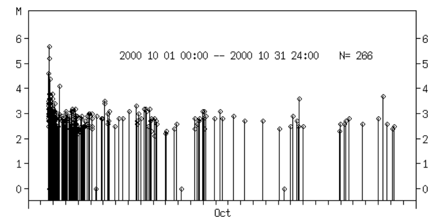
図3 今回の地震活動（上）及び1995年の活動（下）の地震活動経過図（規模別）
