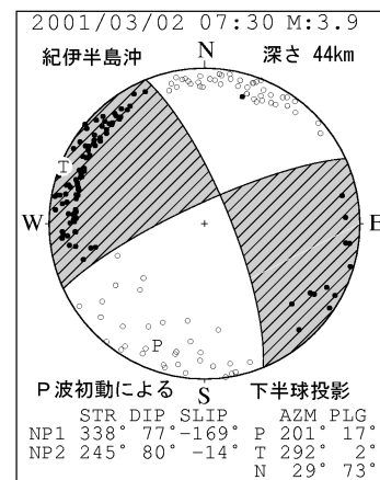
図 6 - 1 紀伊半島沖の地震の発震機構
