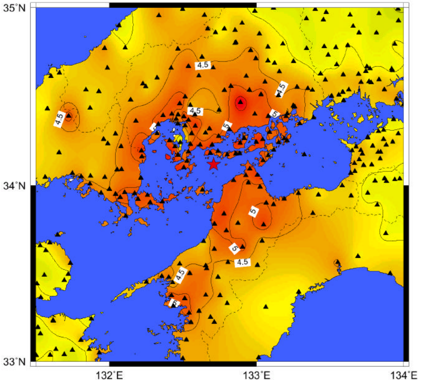
図 1 芸予地震の等計測震度分布
