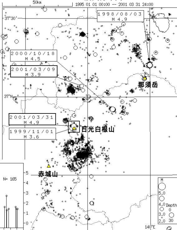
図 5 - 3 栃木県北部の地震活動
