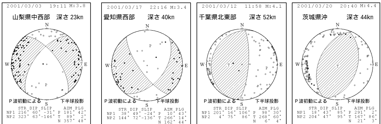
図3 主なP波初動による発震機構＜図中の数字は、本文中の番号に対応する＞
