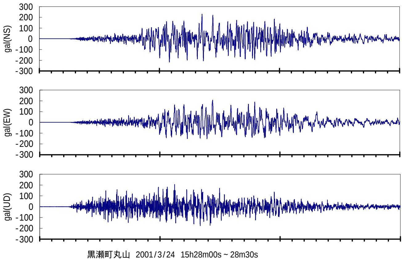
付図 各地の加速度記録（ 2 ）
