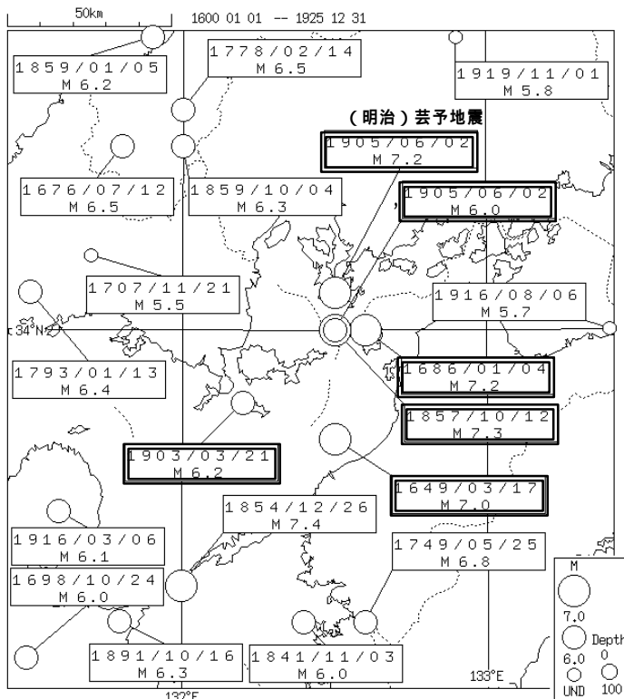
図 3 - 1 - 1 過去の被害地震（1600～1925 年）
