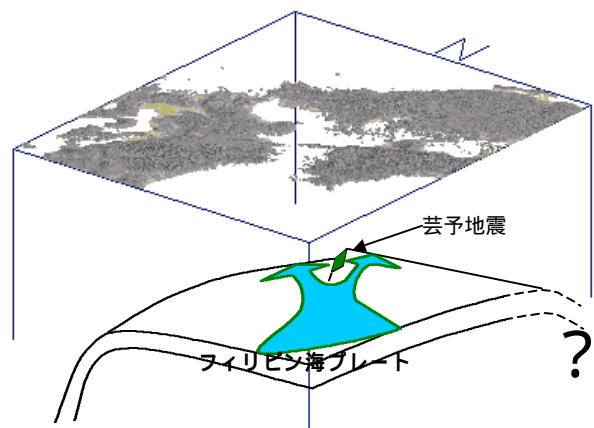
図2 フィリピン海プレートの沈みこみと芸予地震の模式図
