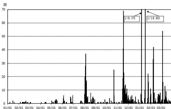
図 2 樽前山 日別地震回数 (2000 年 1 月～2001 年 3 月)
