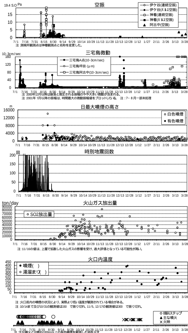
図 7 三宅島火山活動経過図（2000 年 7 月～2001 年 3 月）
