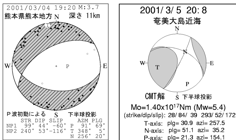
図 7 - 1 発震機構
