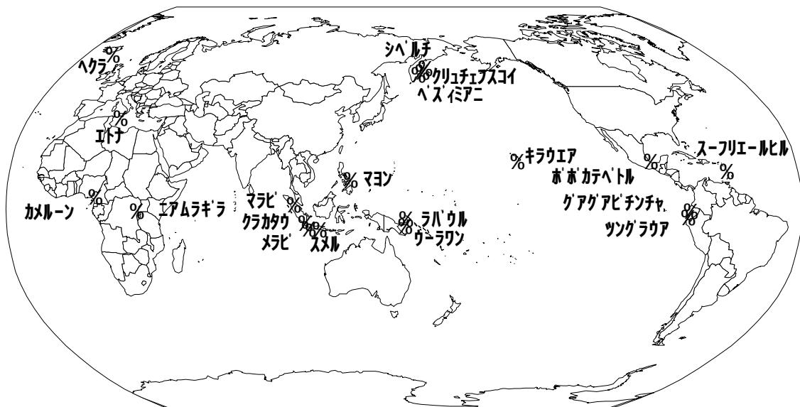
図 1 2000 年（平成 12 年）の海外の主な噴火火山
