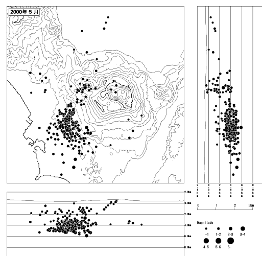
図 7 -a 震源分布図
