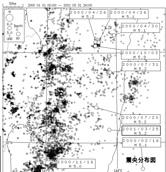
図 4 - 2 三陸沖の地震活動及び発震機構
