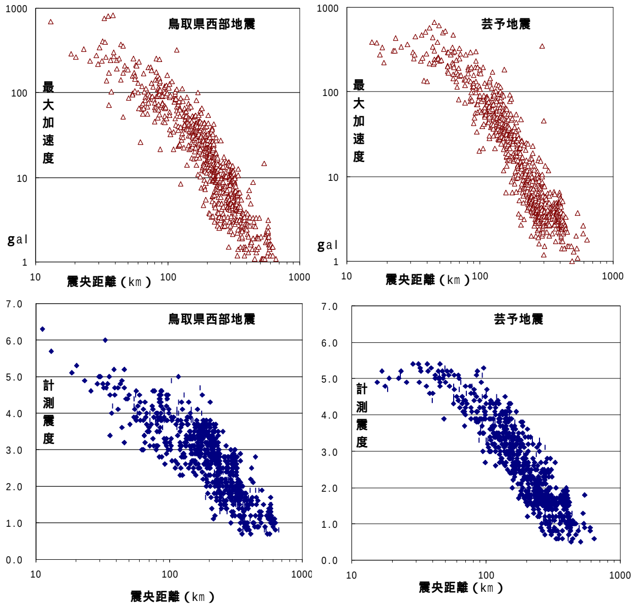
図 1 - 2 鳥取県西部地震（左）と芸予地震（右）における最大加速度（3 成分合成値）と震央距離の関係（上）及び計測震度と震央距離（下）の関係
