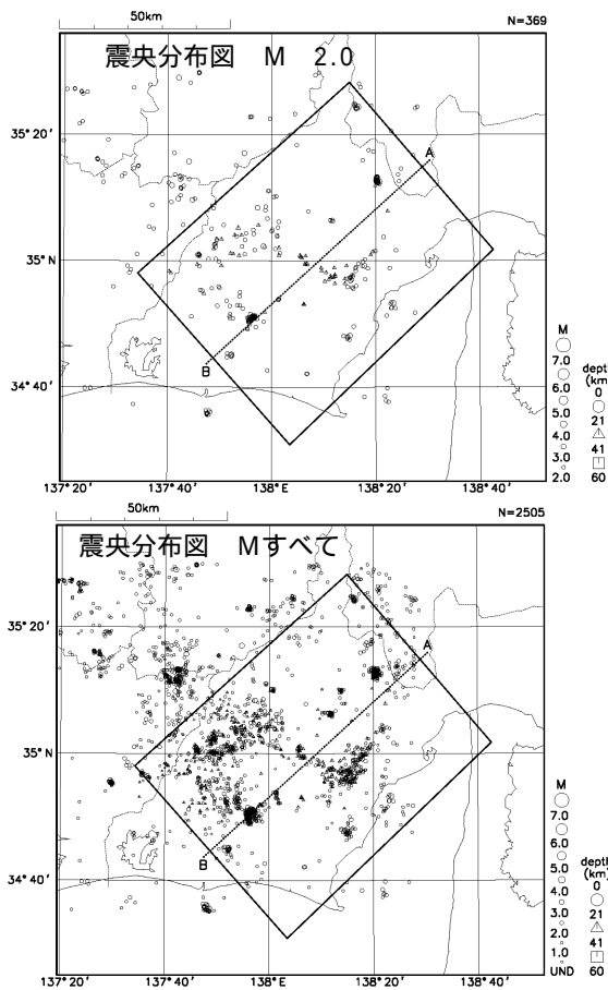
図 4 静岡県中西部（固着域周辺）における地殻内の地震活動（1997 年 1 月～2002 年 2 月）
