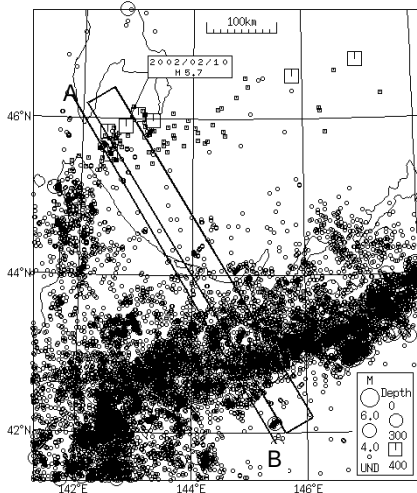
図 3 - 1 宗谷海峡の地震活動
