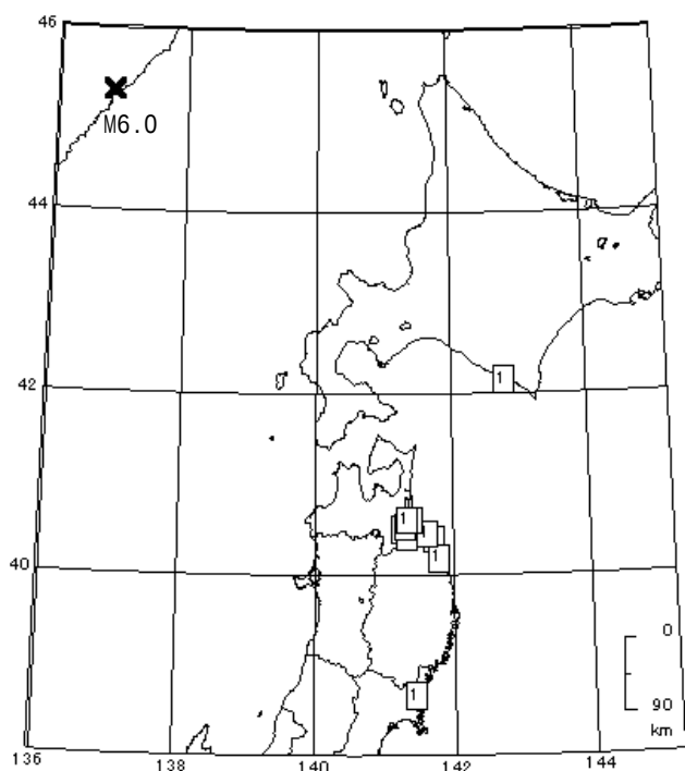
1. 2/2 06:55 クズネ付近 (M6.0、深さ407km)
