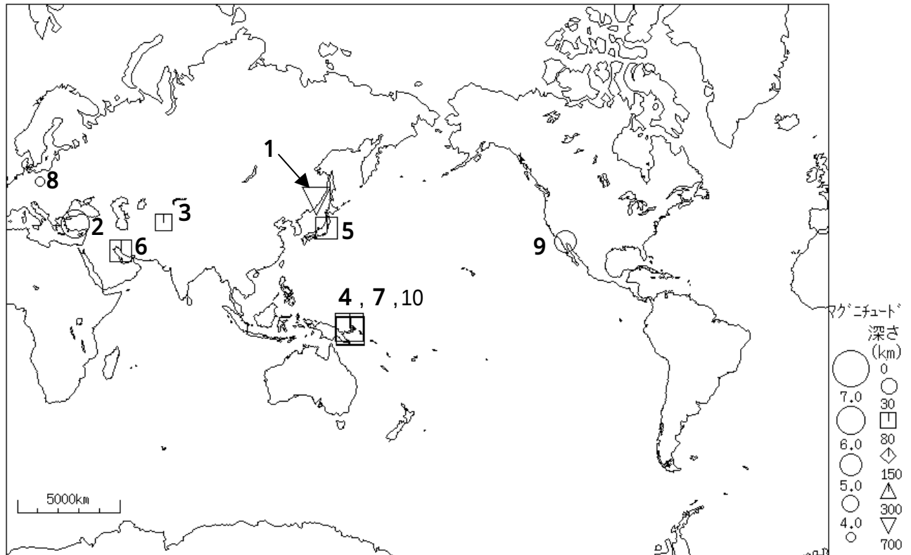
図 1 2002 年 2 月に世界で発生した M6.0 以上または被害を伴った地震の震央分布
