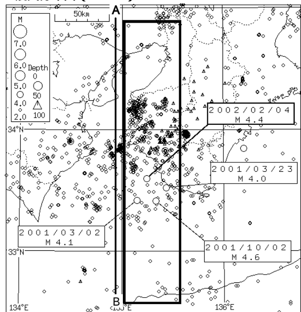
震央分布図 (M 2.0) 2001/1-2002/2
