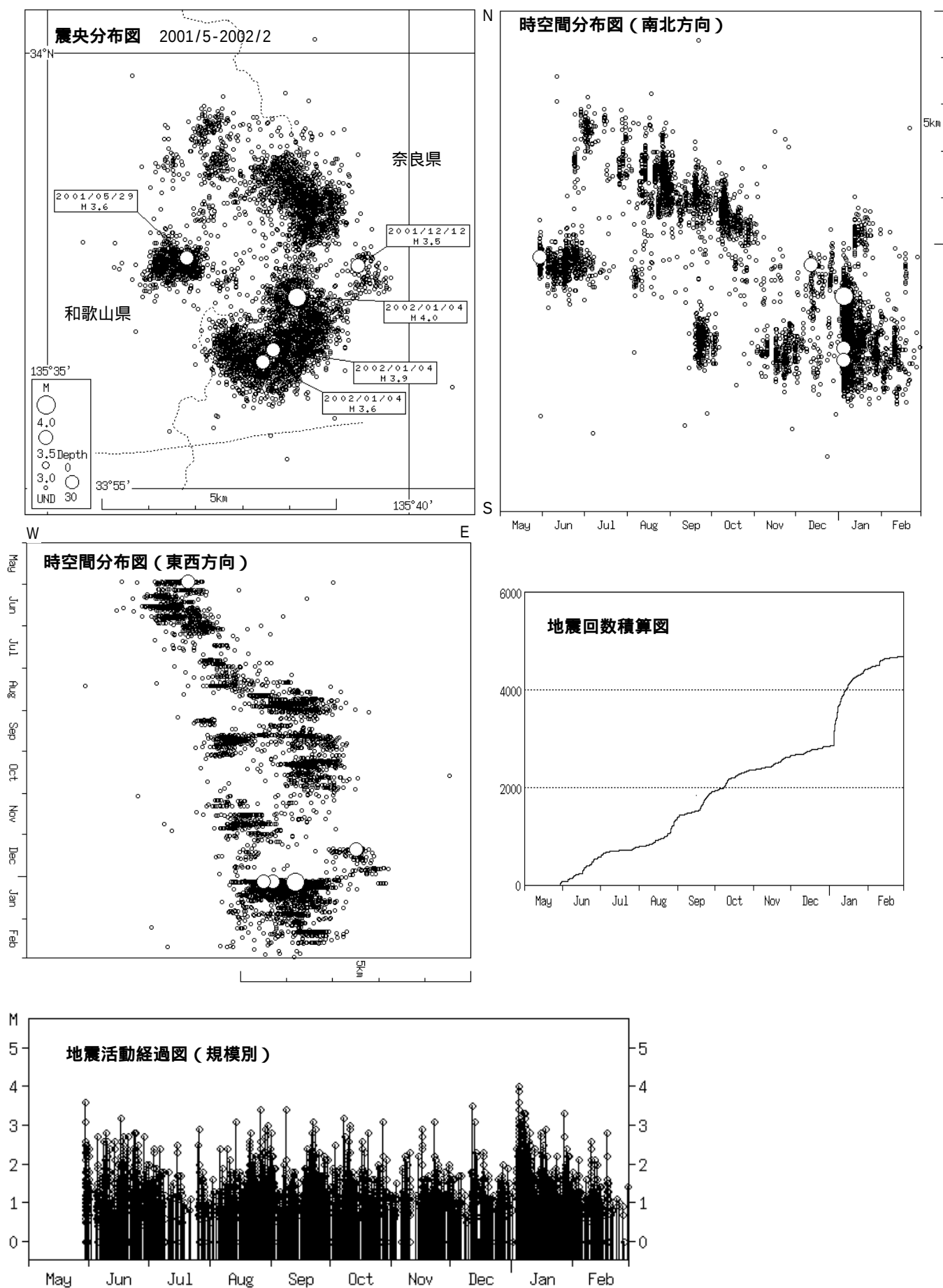
図 6 - 2 和歌山県北部（和歌山・奈良県境付近）の地震活動
