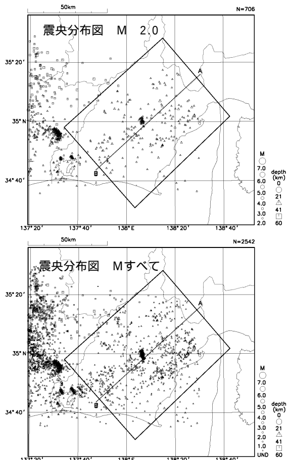
図 5 静岡県中西部（固着域周辺）におけるフィリピン海プレート内の地震活動（1997 年 1 月～2002 年 2 月）
