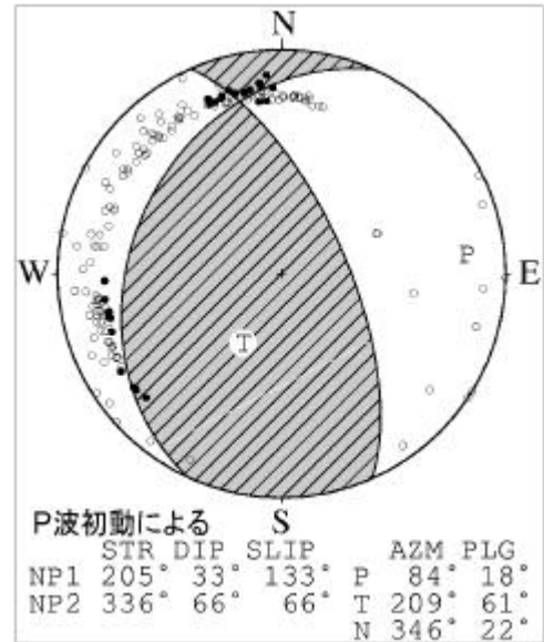
2. 2/11 10:09 茨城県沖 (M5.0、深さ 35km) 東西方向に圧力軸を持つ逆断層型
