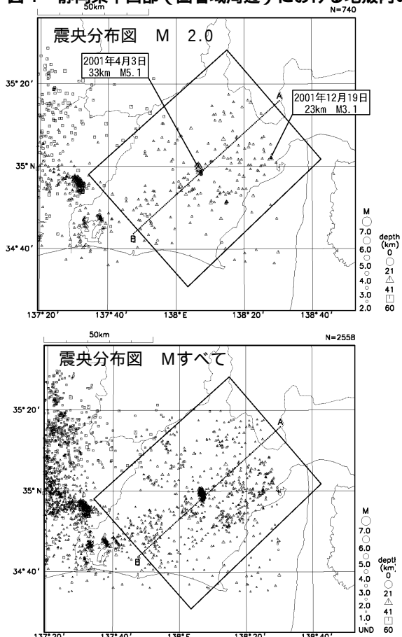
図5 静岡県中西部（固着域周辺）におけるフィリピン海プレート内の地震活動（1997 年 1 月～2002 年 1 月）
