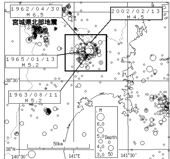
震央分布図(M 3.0) 1950/1-2002/2
