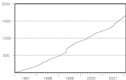
左図矩形内の地震回数積算図 2001 年半ば以降、地震回数はやや多い状態
