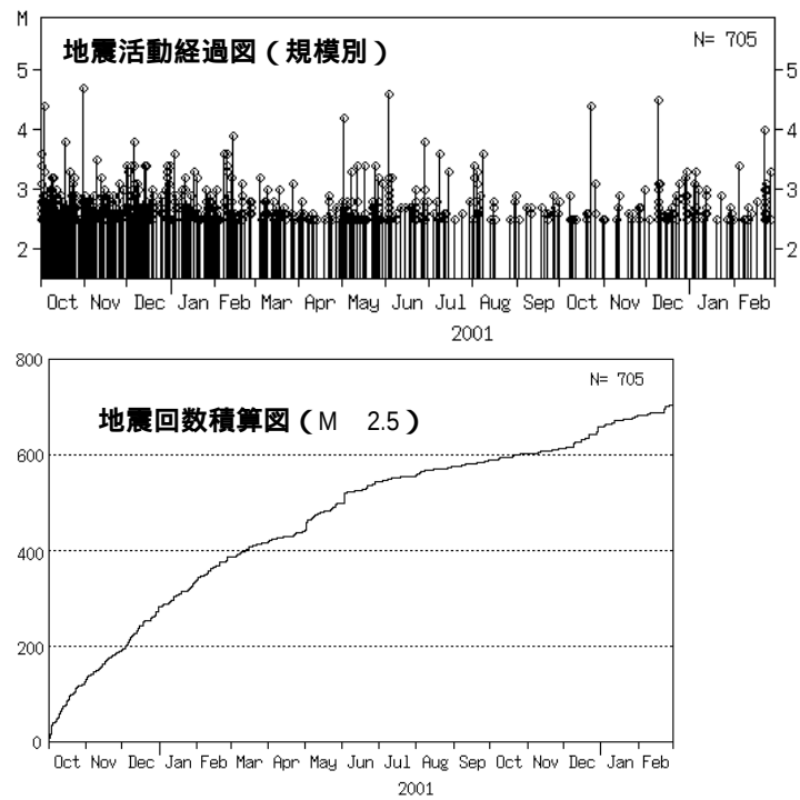
図 5 - 1 三宅島近海～新島・神津島近海の地震活動 (2000 年 10 月～2002 年 2 月)
