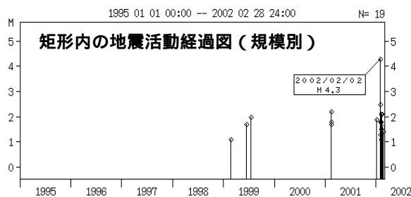
図 5 - 2 新潟県中越地方の地震活動
