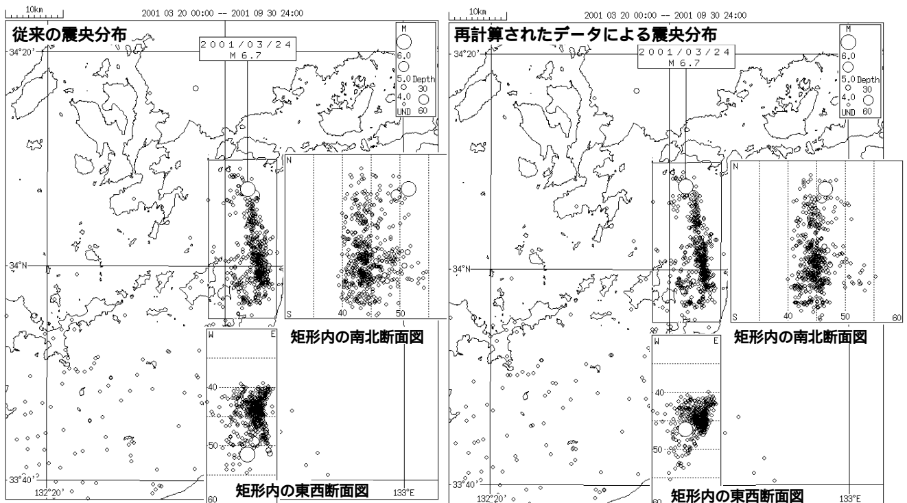
図 2 旧震源と新震源の比較の例（2001 年の芸予地震とその余震活動）表示期間：2001/3/20-2001/9/30
