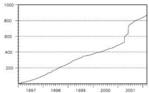
左図矩形内の地震回数積算図 2001 年半ば以降、地震回数は平常の状態
