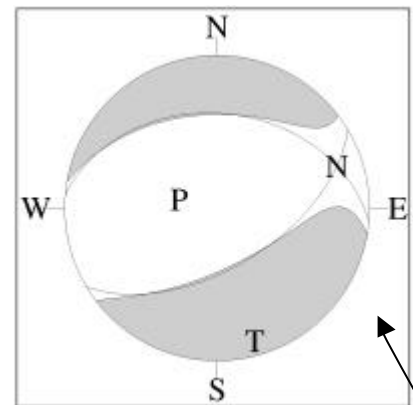
図 2 . 発震機構（ハーバード大学による） 1990 年以降、各発震機構からのびる線は張力軸の方向である。
