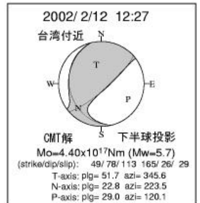
図 8 - 2 台湾付近の地震の CMT 解
