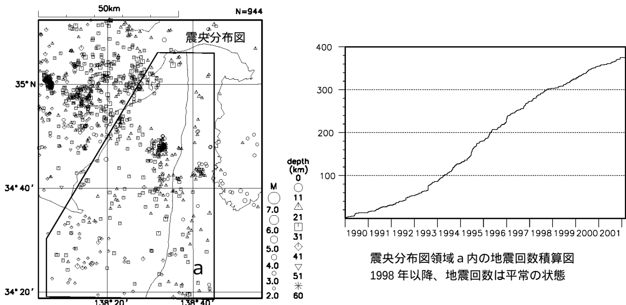
図 3 駿河湾の地震活動（1990 年 1 月～2002 年 2 月、M2.0 以上）
