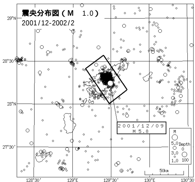
図 7 - 1 奄美大島近海の地震（余震）活動
