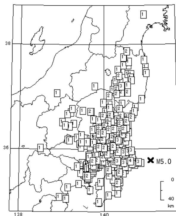
2. 2/11 10:09 茨城県沖 (M5.0、深さ35km)
