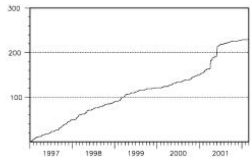
左図矩形内の地震回数積算図 2001 年半ば以降、地震回数はやや少ない状態
