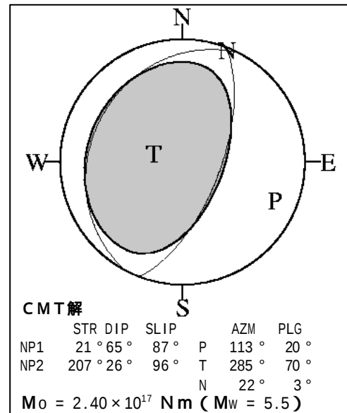
3. 2/12 22:44 茨城県沖 (M5.5、深さ 48km) 西北西 - 東南東方向に圧力軸を持つ逆断層型
