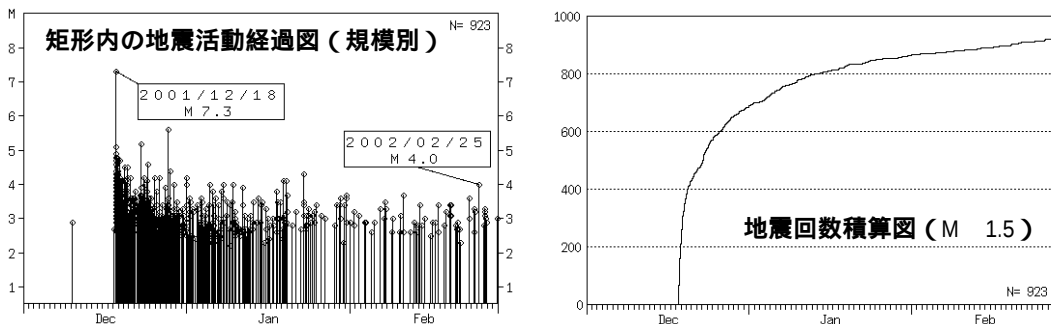
図 8 - 1 与那国島近海の地震活動
