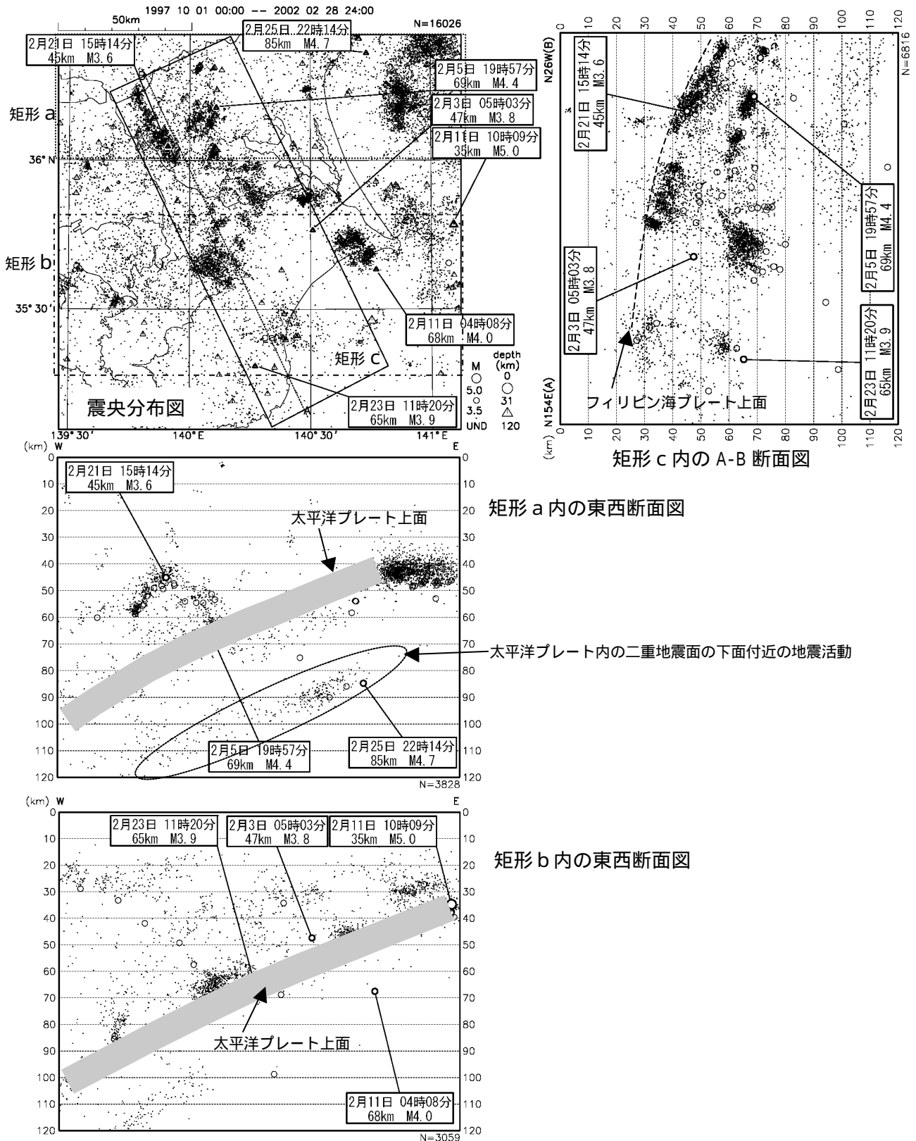
図7 南関東地域の地震活動 表示期間：1997年10月1日～2002年2月28日
