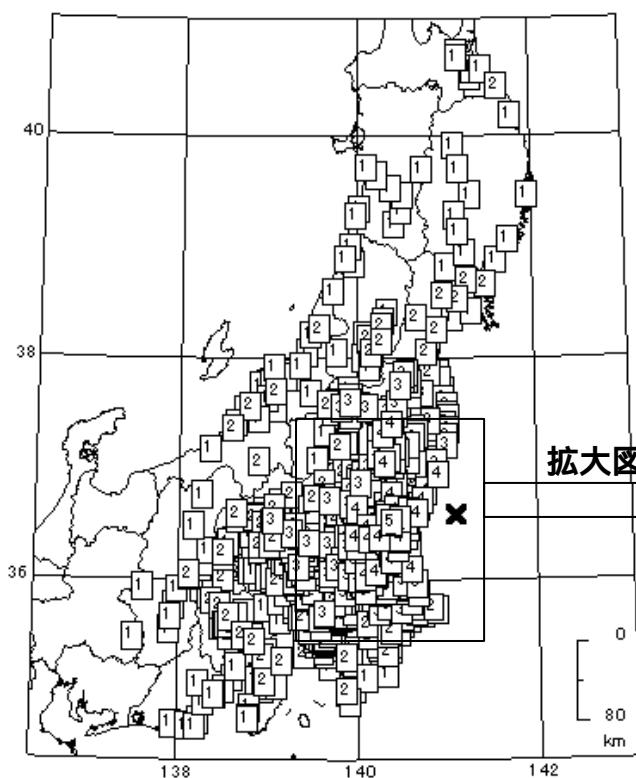
3. 2/12 22:44 茨城県沖 (M5.5、深さ48km)
