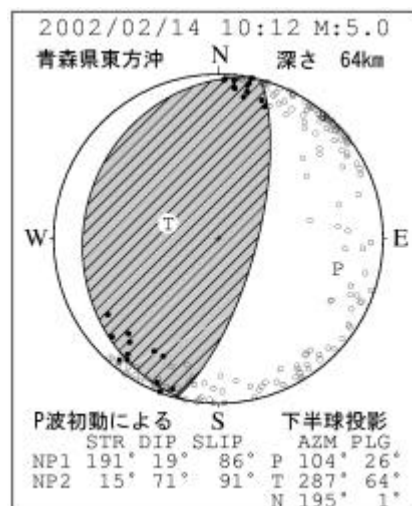
図 4 - 2 青森県東方沖の地震活動
