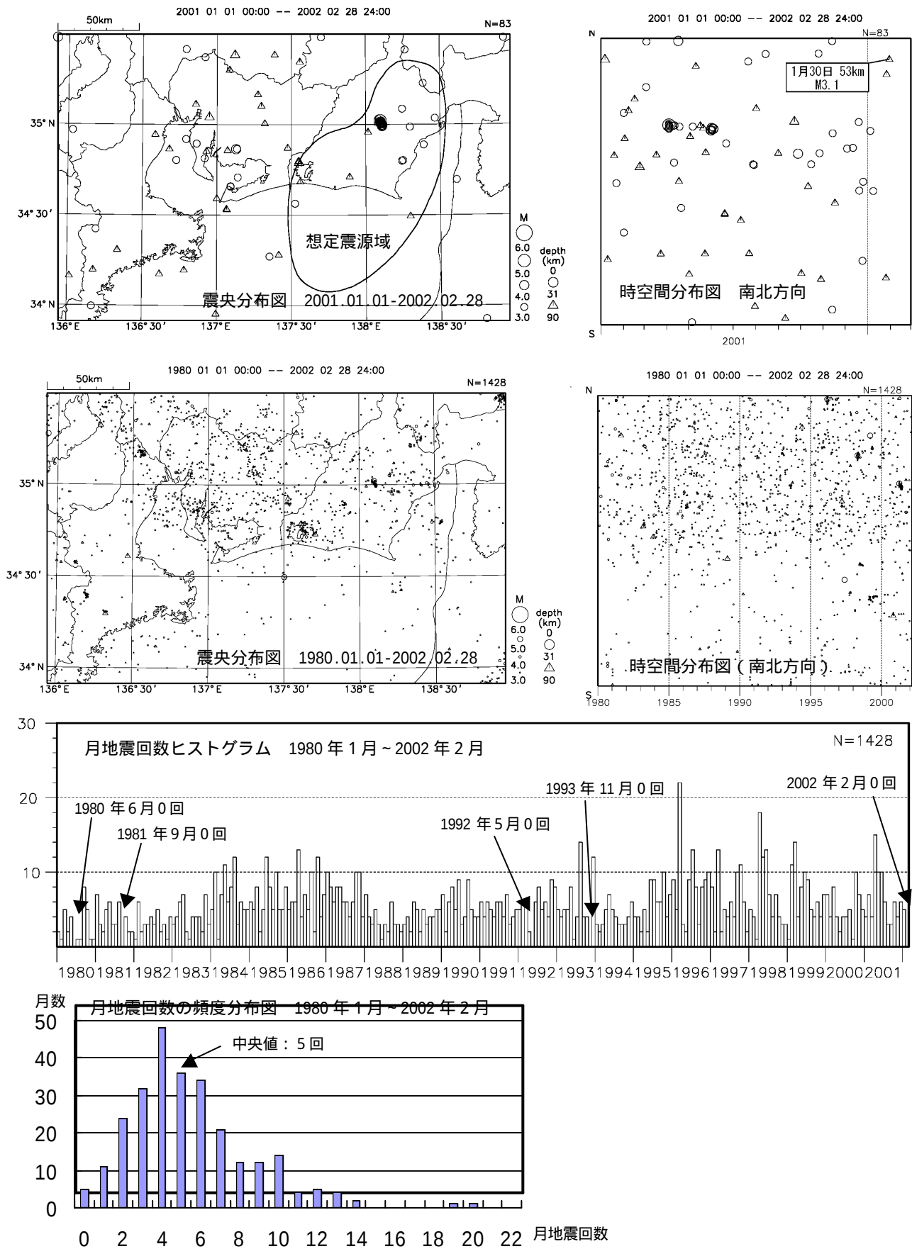
図6 東海地域の地震活動 M 3.0
