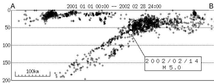
左上図矩形内の断面図
