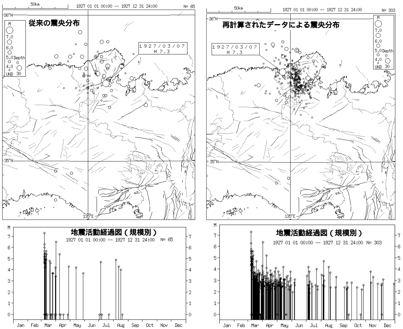
図 1 旧震源と新震源の比較の例（1927 年の北丹後地震とその余震活動）表示期間：1927/1/1-1927/12/31
