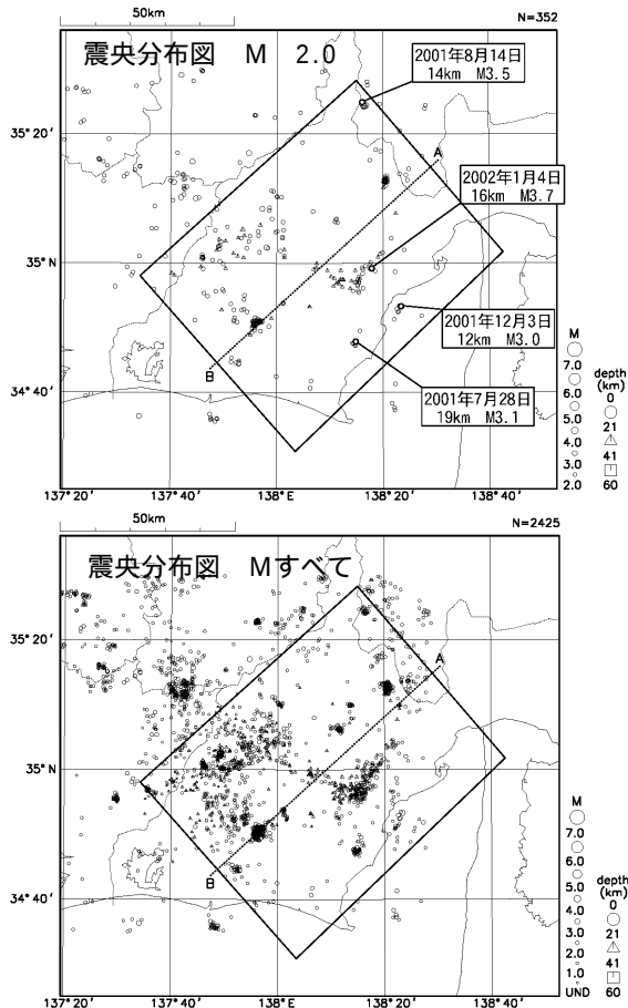
図4 静岡県中西部（固着域周辺）における地殻内の地震活動（1997 年 1 月～2002 年 1 月）
