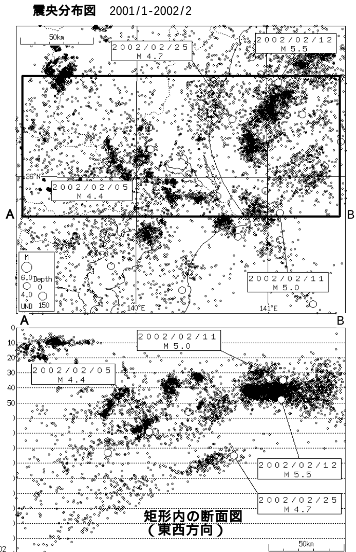
図 5 - 3 茨城県南部、茨城県沖、鹿島灘の地震活動
