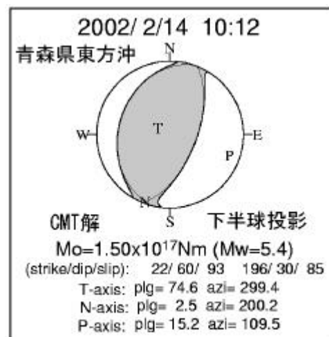
図 4 - 2 青森県東方沖の地震活動
