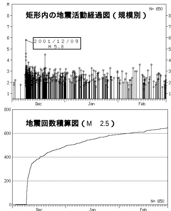
図 7 - 1 奄美大島近海の地震（余震）活動
