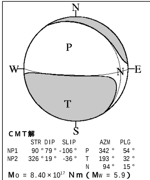
1. 2/2 06:55 蔵利列島付近 (M6.0、深さ 407km) プレートの沈み込む方向（北北西）に圧力軸を持つ
