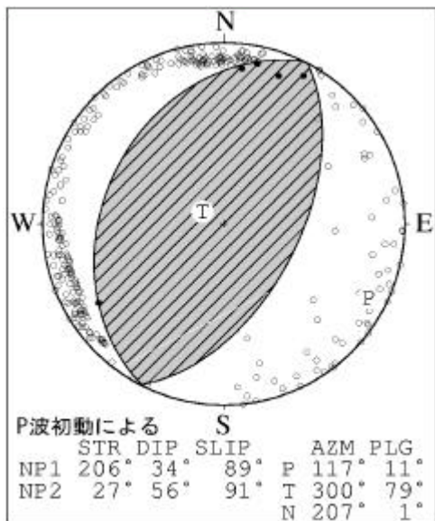
3. 2/12 22:44 茨城県沖 (M5.5、深さ 48km) 西北西 - 東南東方向に圧力軸を持つ逆断層型
