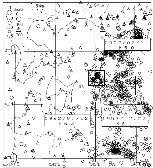
震央分布図 (M 4.5) 1950/1～2002/2
