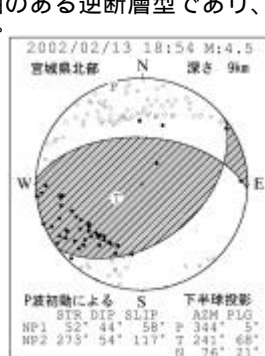
図 4 - 1 宮城県北部の地震活動
