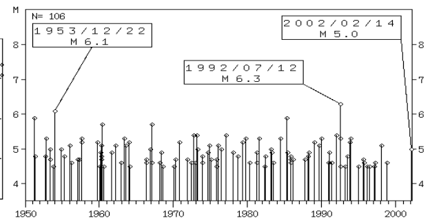
右上図矩形内の地震活動経過図(規模別)
