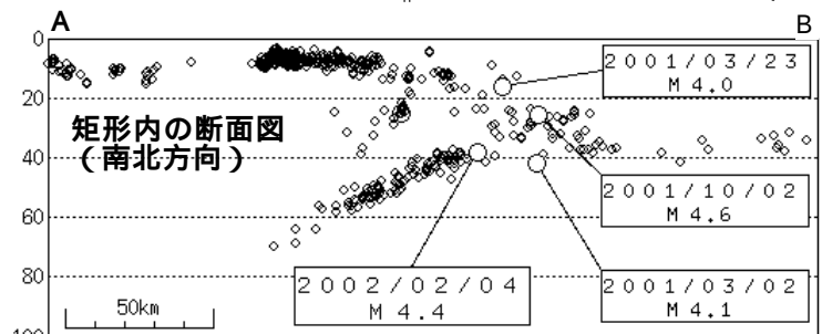
図 6 - 1 紀伊水道の地震活動
