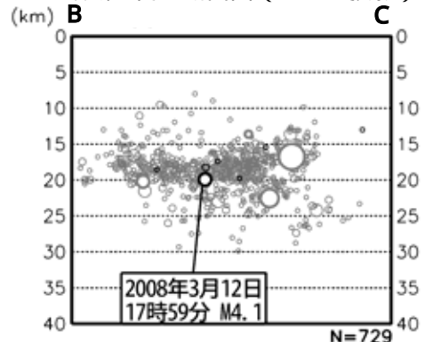
領域 a 内の断面図（B - C 投影）
