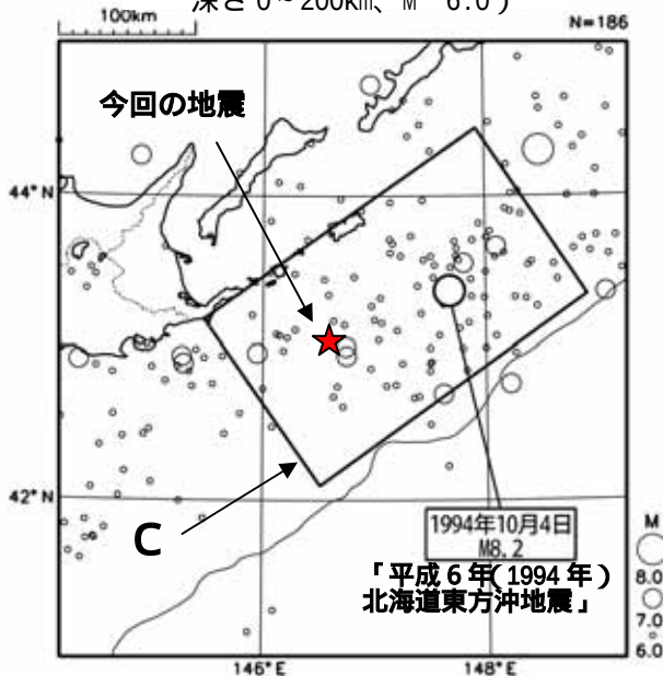
震央分布図 （1923 年 8 月 1 日～2008 年 3 月 31 日 深さ 0～200km、M 6.0）
