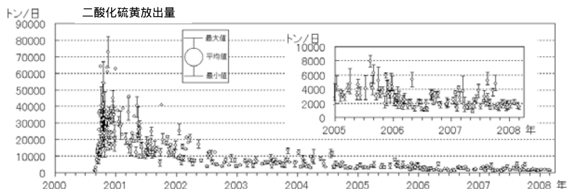
図2 三宅島 二酸化硫黄の放出量の推移（2000年1月～2008年3月）
