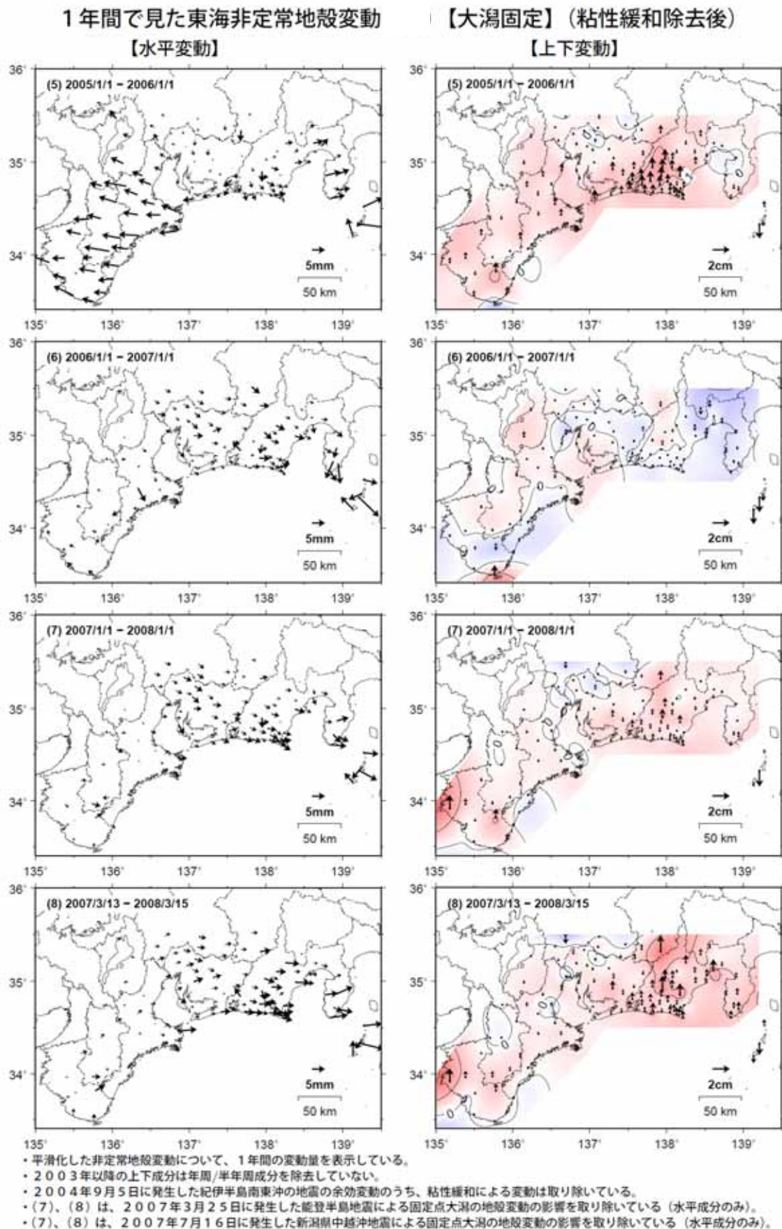
図 9 国土地理院の GPS 観測結果による 1 年間で見た東海非定常地殻変動
