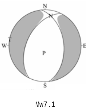
今回の地震の発震機構 （Global CMT 解）
