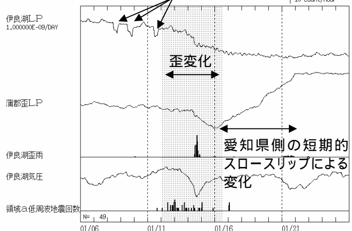
伊良湖の歪変化（2006年1月6日～1月25日）
