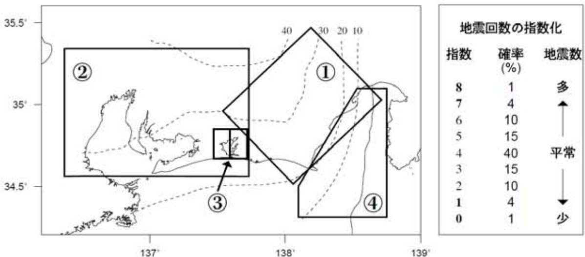
図 4 東海地域の地震活動指数
