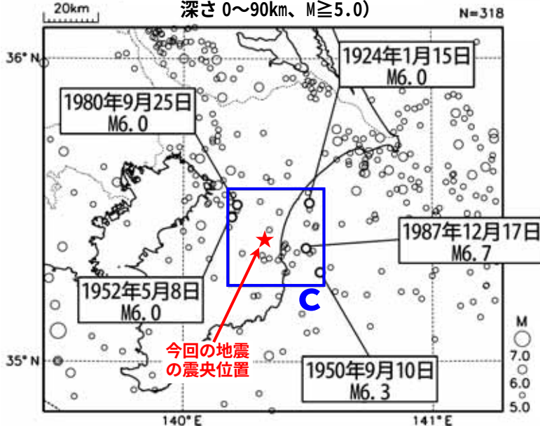
震央分布図（1923 年 8 月 1 日～2008 年 10 月 31 日、 深さ 0～90km、 M \geq 5.0 ）
