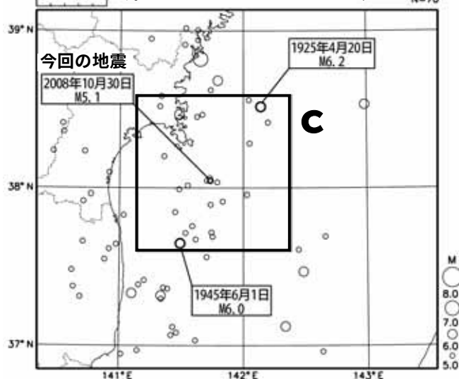
震央分布図 （1923 年 8 月 1 日～2008 年 10 月 31 日 深さ 70 km～150 km M \geq 5.0 ）
