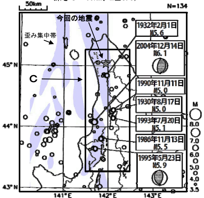
震央分布図 (1923 年 8 月 1 日～2008 年 10 月 31 日 深さ 0～60km、 M \geq 3.5 )
