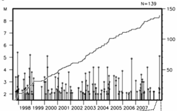
領域 b 内の M-T 図と回数積算図
