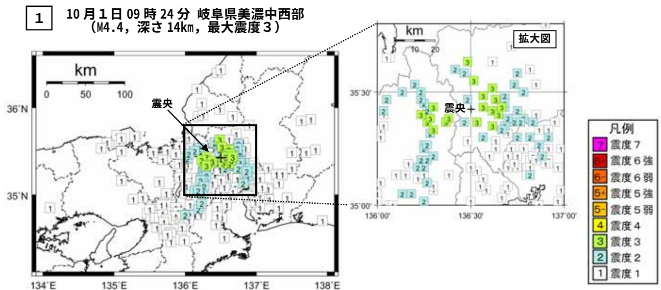
図 2 震度分布図（各図の左上の数字は表 1，図 1 の番号に対応する。+印は震央を示す。）
