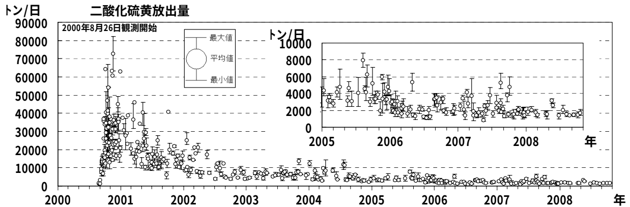
図4 三宅島 二酸化硫黄の放出量 8) の推移（2000年8月～2008年10月）
