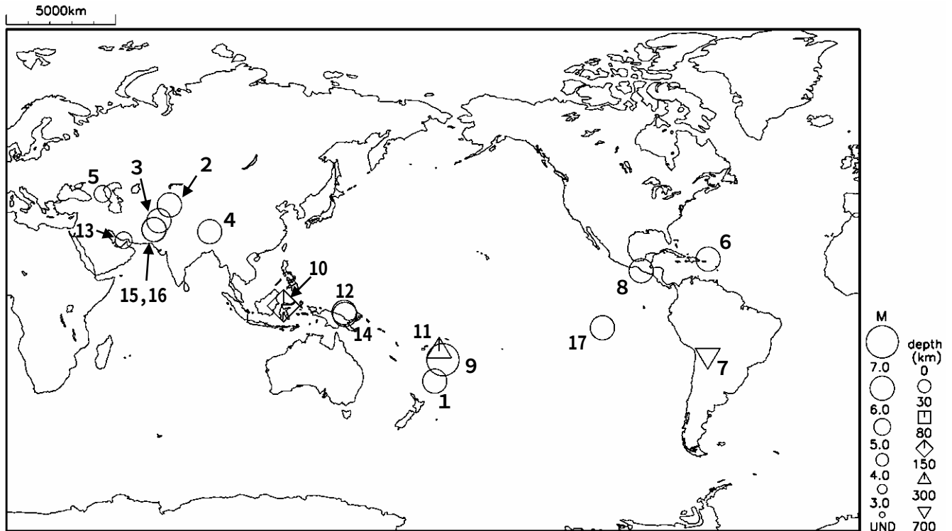
図 1 平成 20 年（2008 年）10 月に世界で発生した M6.0 以上または被害を伴った地震の震央分布
