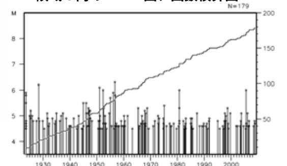
領域 c 内の M-T 図、回数積算図
