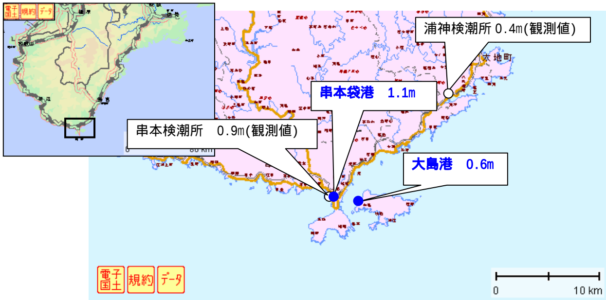
図 3 - 1 4 推定した津波の高さと観測点での津波の高さ（● 推定した地点 ○ 観測点）
