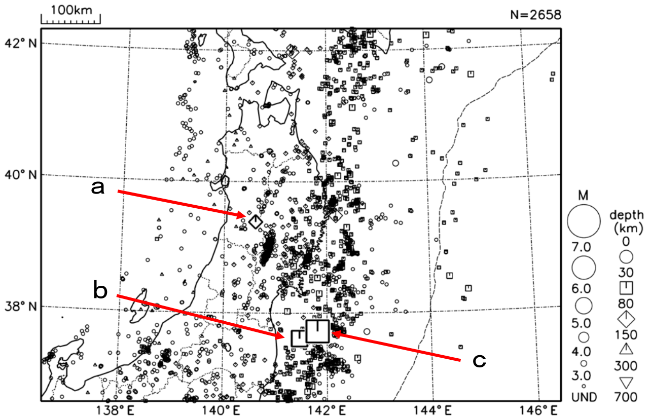
図 4 東北地方の震央分布図（2010 年 3 月 1 日～3 月 31 日）
