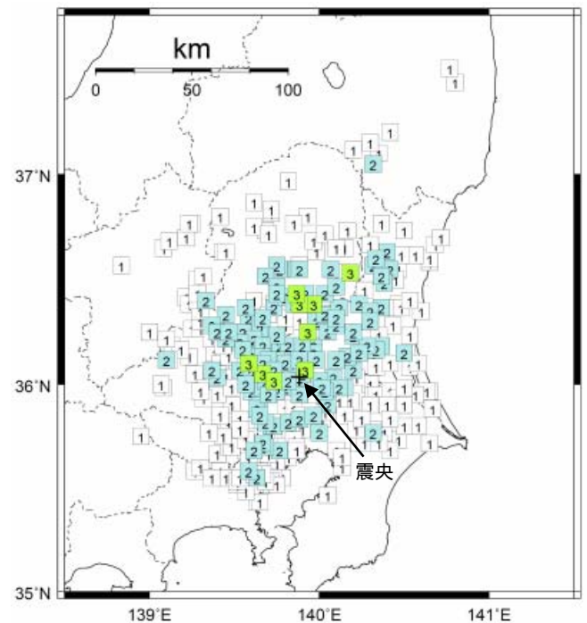
7 3月29日10時29分 茨城県南部 (M4.3、深さ43km、最大震度3)
