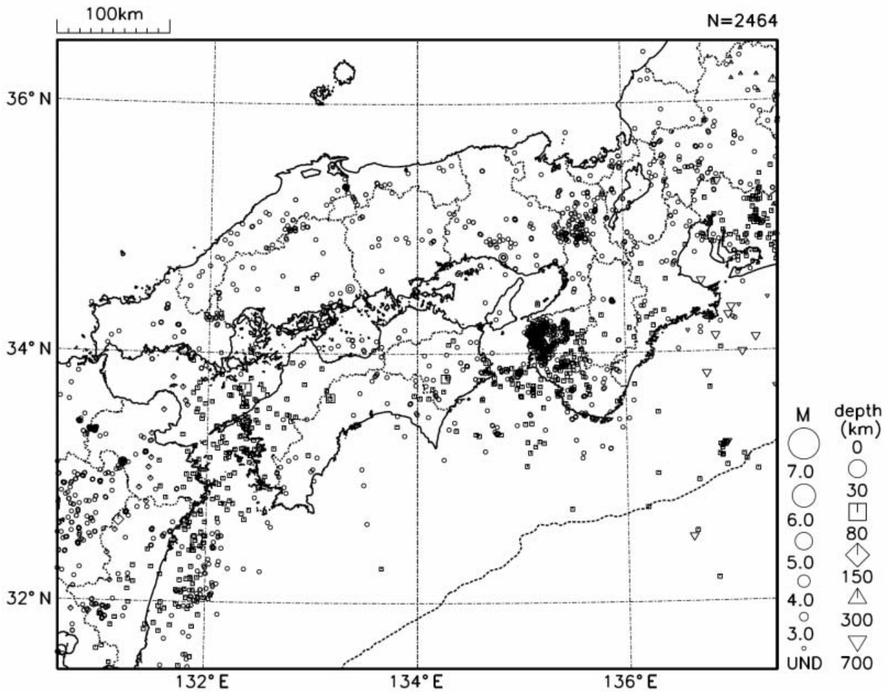
図 6 近畿・中国・四国地方の震央分布図（2010 年 3 月 1 日～3 月 31 日）
