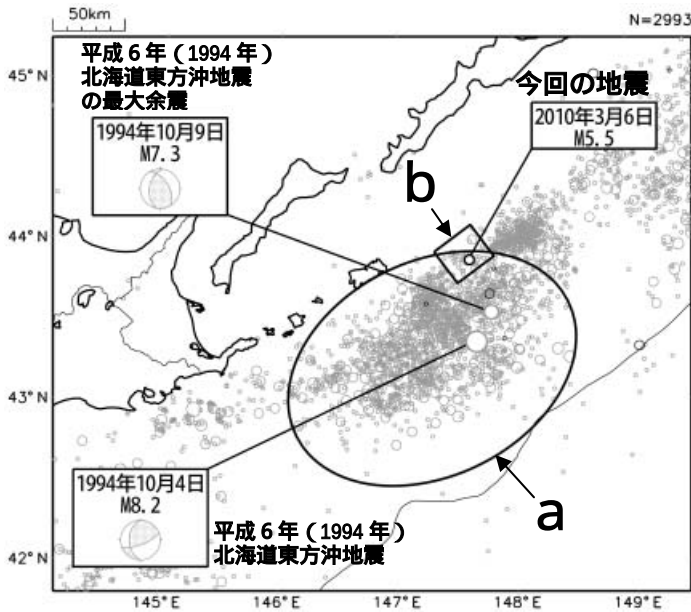
震央分布図 (1994 年 10 月 1 日～2010 年 3 月 31 日、 深さ 0～60km、M 4.0) 2010 年 3 月以降の地震を濃く表示
