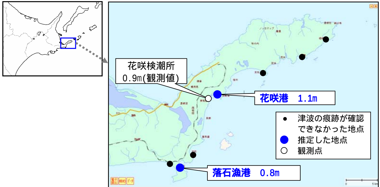
図 3 - 1 0 推定した津波の高さと観測点での津波の高さ
