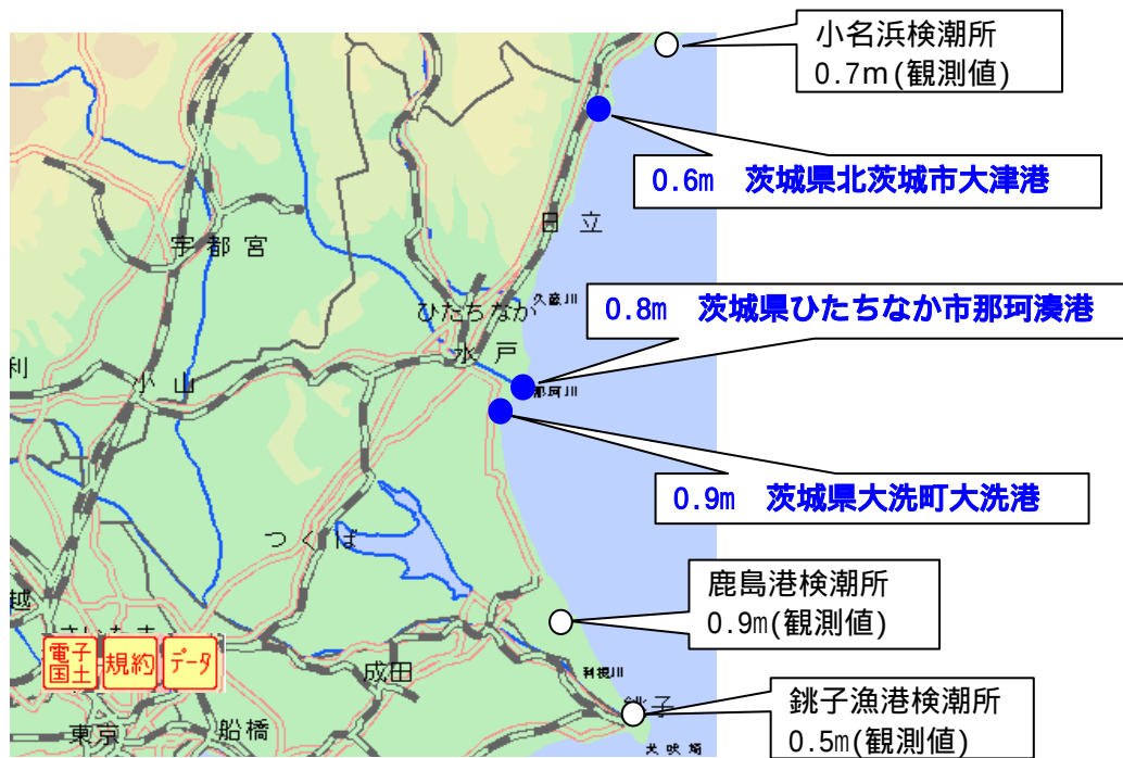
図 3 - 1 2 推定した津波の高さと観測点での津波の高さ（● 推定した地点 ○ 観測点）
