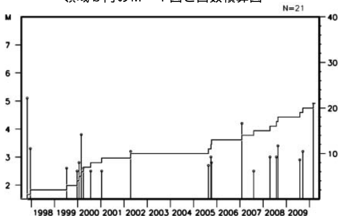
領域 b 内の M - T 図と回数積算図
