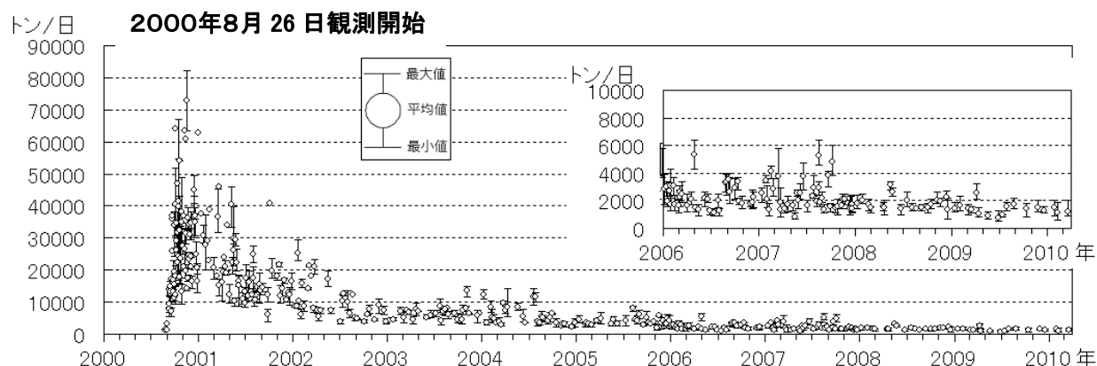
図 3 三宅島 二酸化硫黄の放出量 5) の推移（2000 年 8 月～2010 年 3 月）
