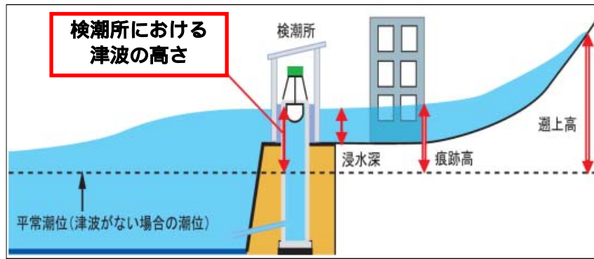
図 3 - 2 検潮所における津波の高さと痕跡高の関係
