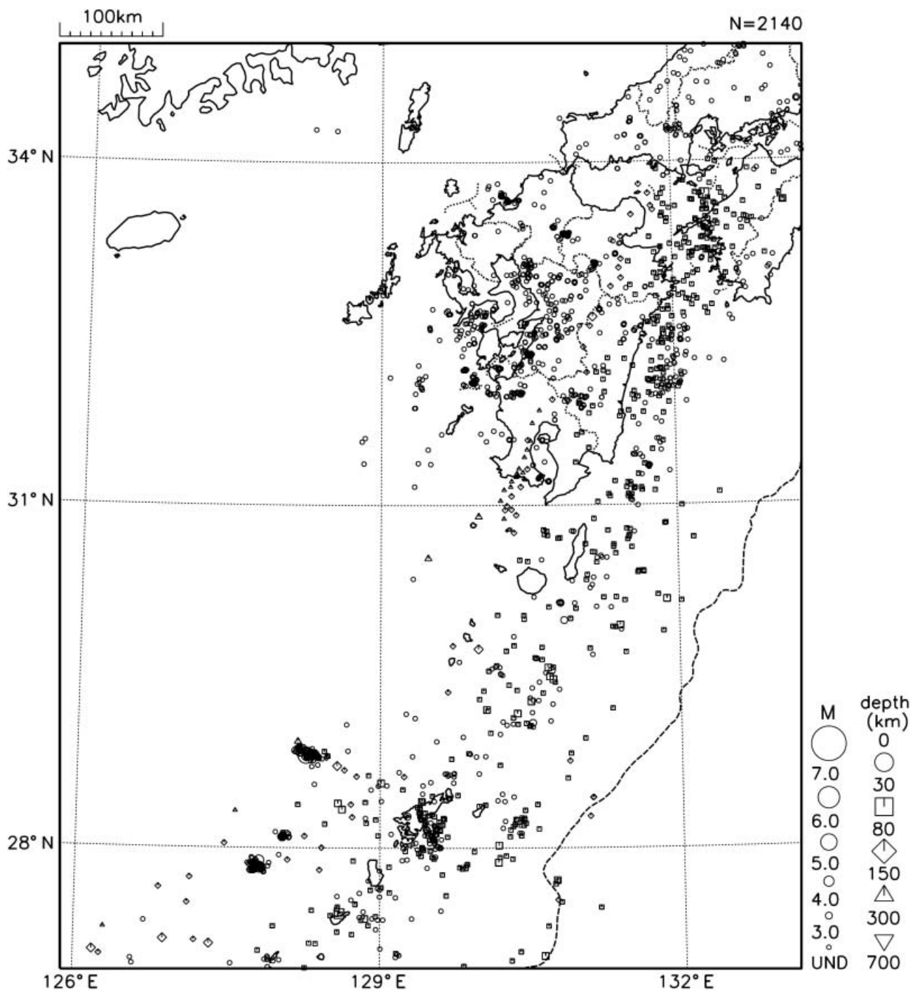
図7 九州地方の震央分布図（2010年3月1日～3月31日）
