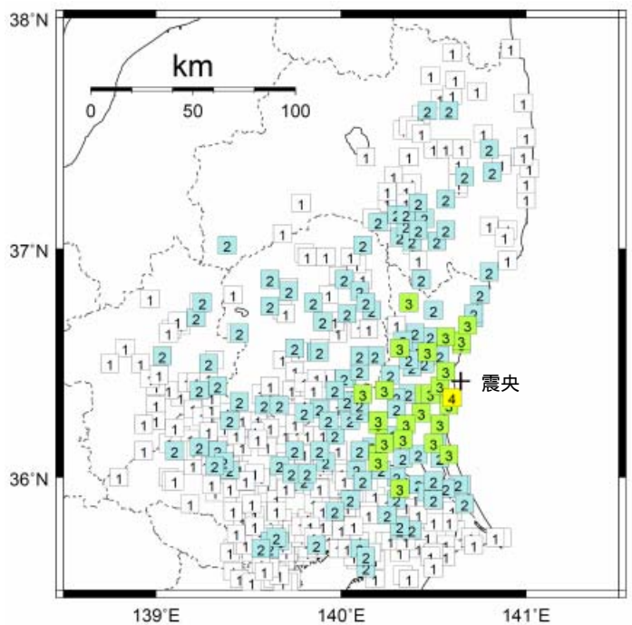
9 3月31日06時18分 茨城県沖 (M4.6、深さ55km、最大震度4)
