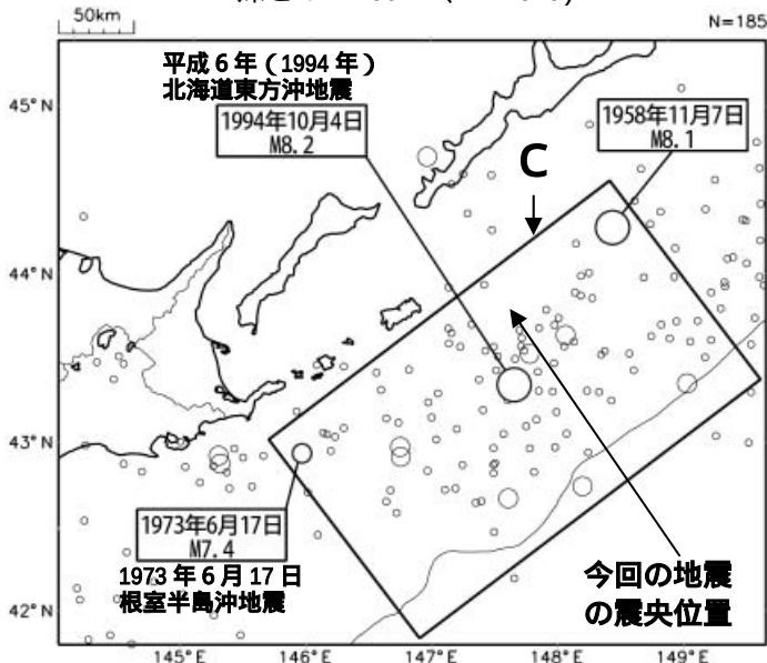
震央分布図 (1923 年 8 月 1 日～2010 年 3 月 31 日、 深さ 0～100km、M 6.0)
