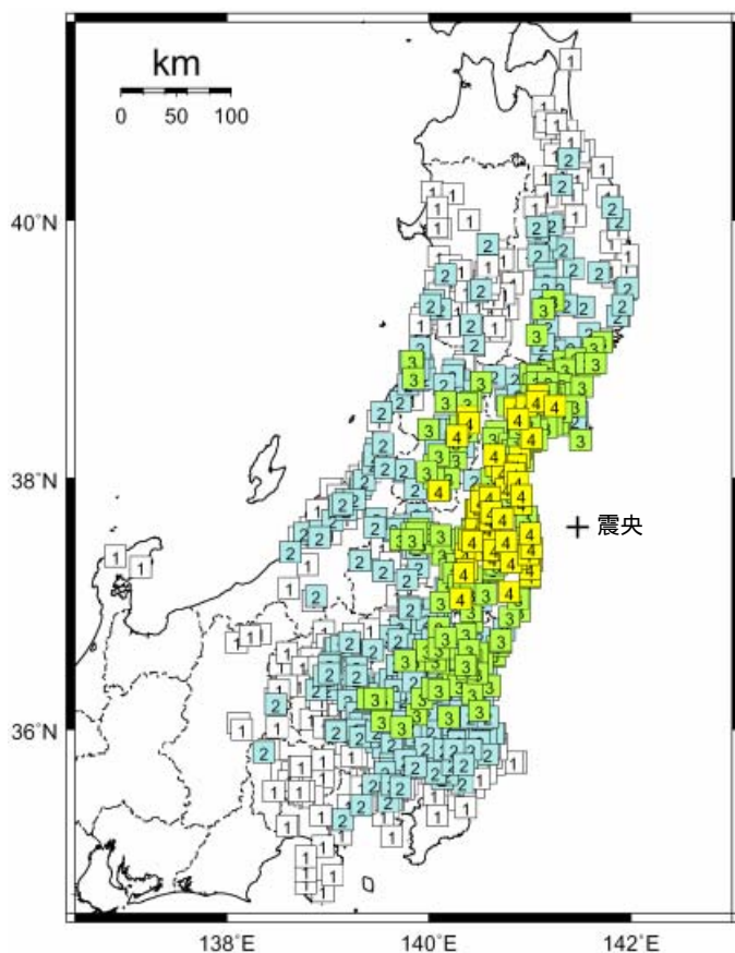
図 2 - 1 震度分布図（各図の左上の数字は表 1，図 1 の番号に対応する。+ 印は震央を示す）
