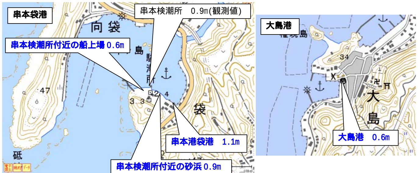
図 3 - 1 4 推定した津波の高さと観測点での津波の高さ（● 推定した地点 ○ 観測点）
