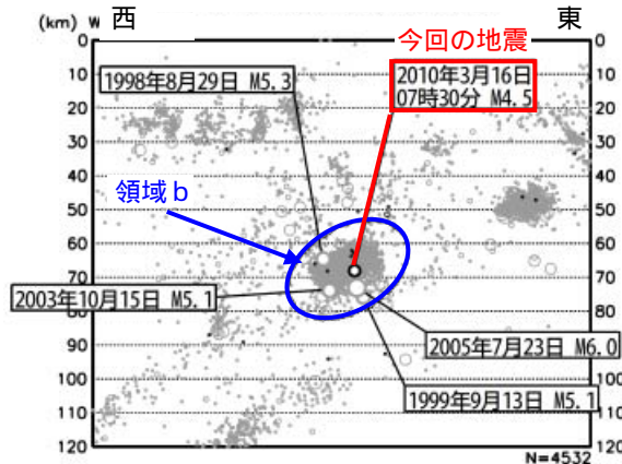
領域 a 内の断面図（東西方向投影）
