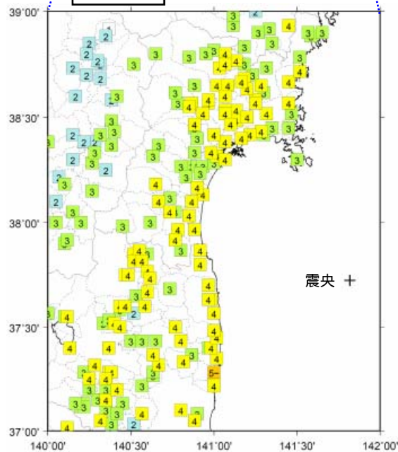
図 2 - 2 震度分布図（各図の左上の数字は表 1，図 1 の番号に対応する。+ 印は震央を示す）
