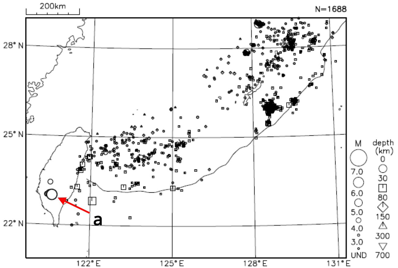
図 8 沖縄地方の震央分布図（2010 年 3 月 1 日～ 3 月 31 日）
