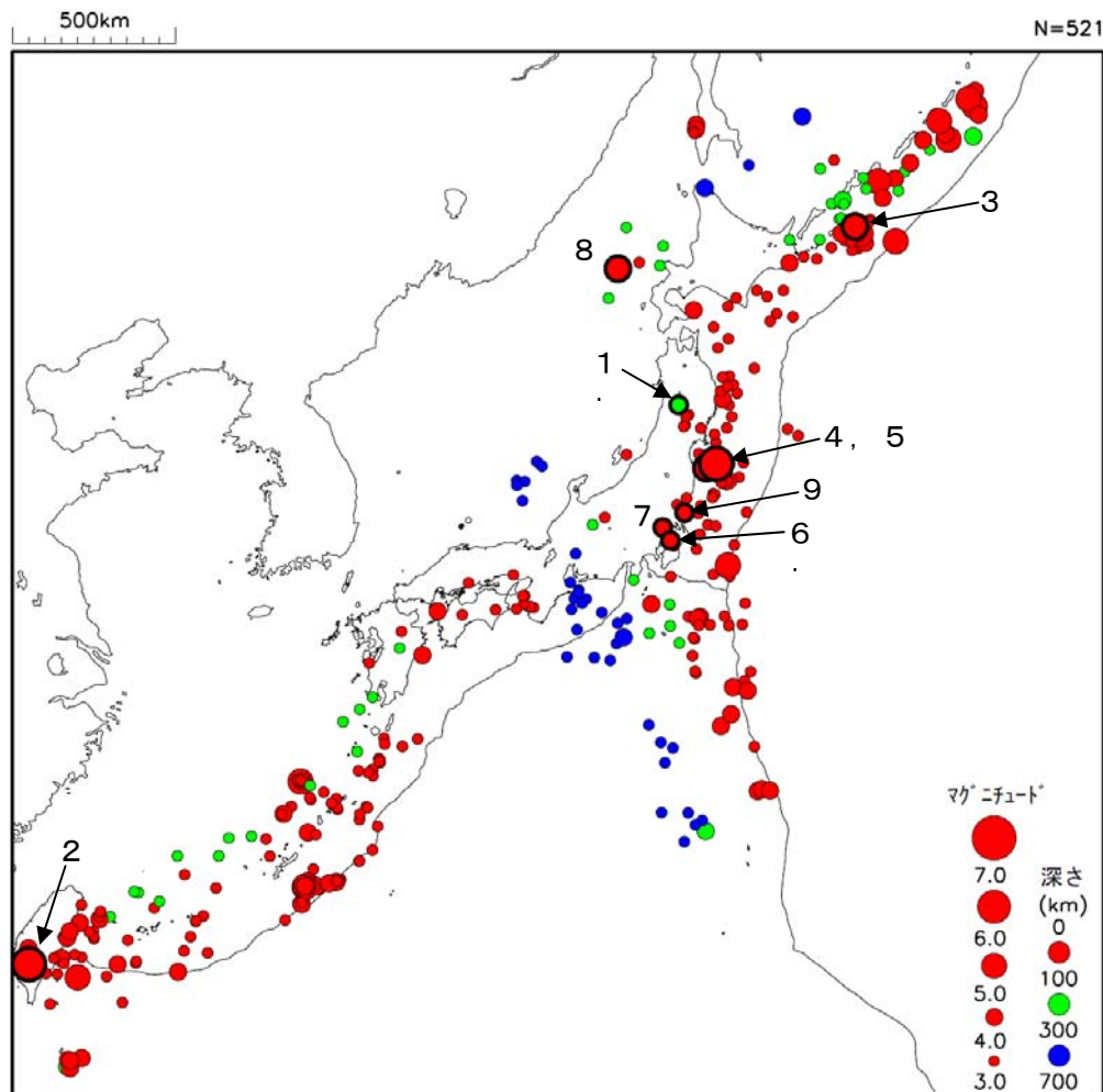
図 1 平成 22 年 3 月に日本及びその周辺で発生した M3.0 以上の地震の震央分布図（図中の数字は表 1 の番号に対応）
