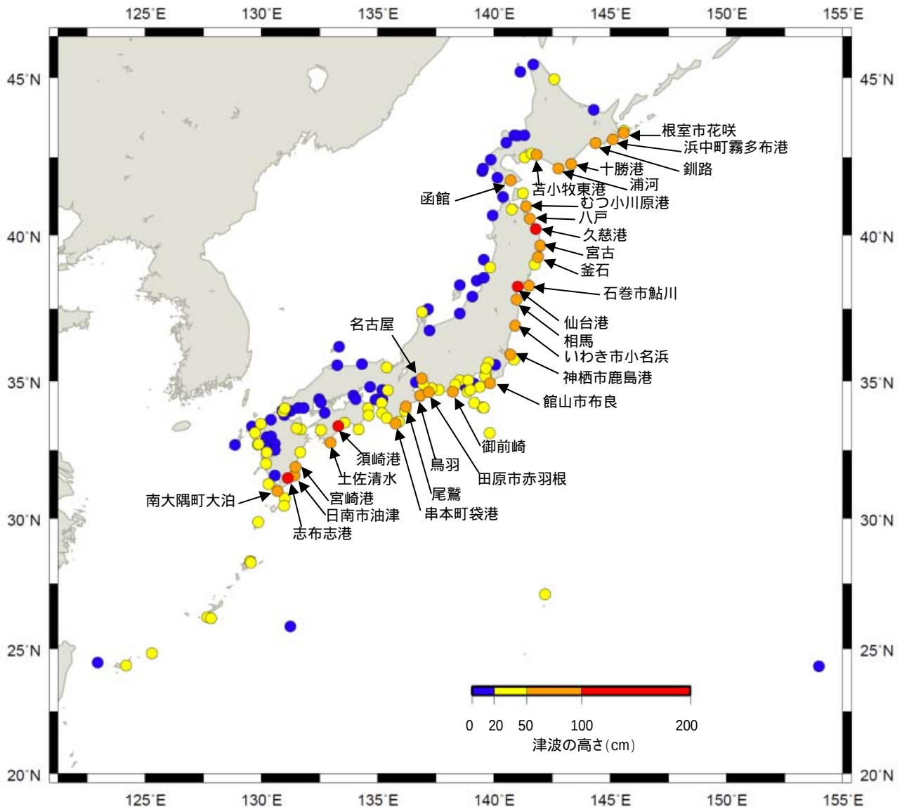
図 2 観測された津波の最大の高さ
