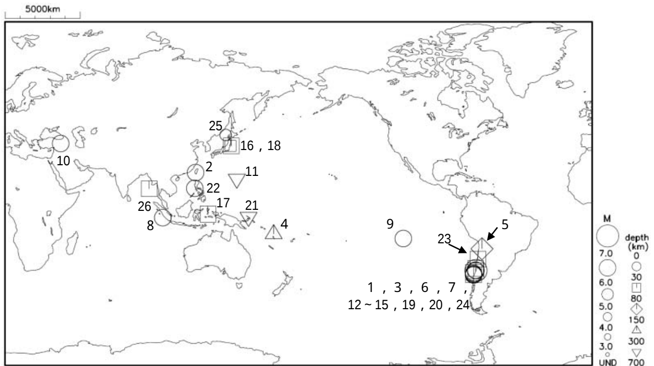
図 1 平成 22 年（2010 年）3 月に世界で発生した M6.0 以上または被害を伴った地震の震央分布
