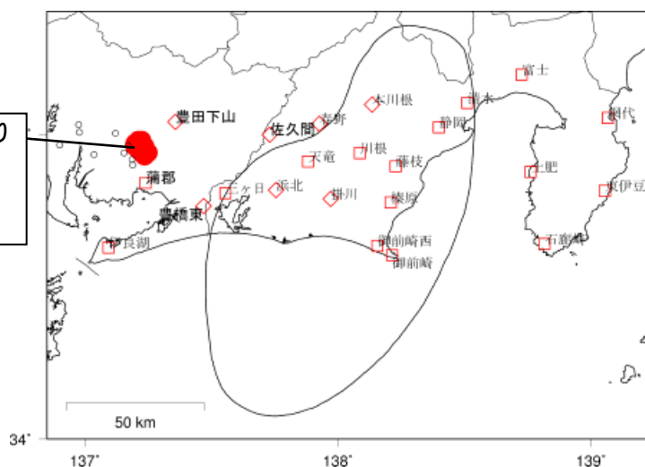
図5 3月10日から11日の歪変化から推定された短期的ゆっくり滑り
