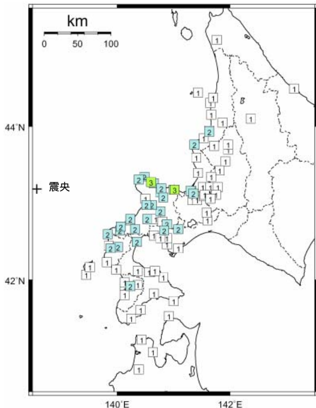
図 2 - 3 震度分布図（各図の左上の数字は表 1，図 1 の番号に対応する。+ 印は震央を示す）
