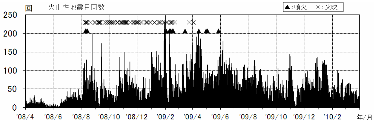
図 2 浅間山 火山性地震の日回数（2008 年 4 月 1 日～2010 年 3 月 31 日）
