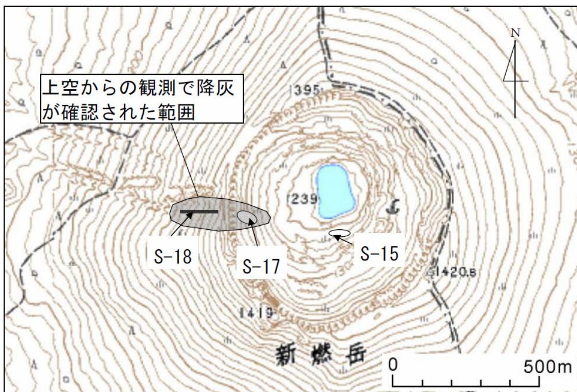
図5 霧島山（新燃岳）30 日に行った上空からの観測で確認された降灰範囲（図中の灰色部分）
