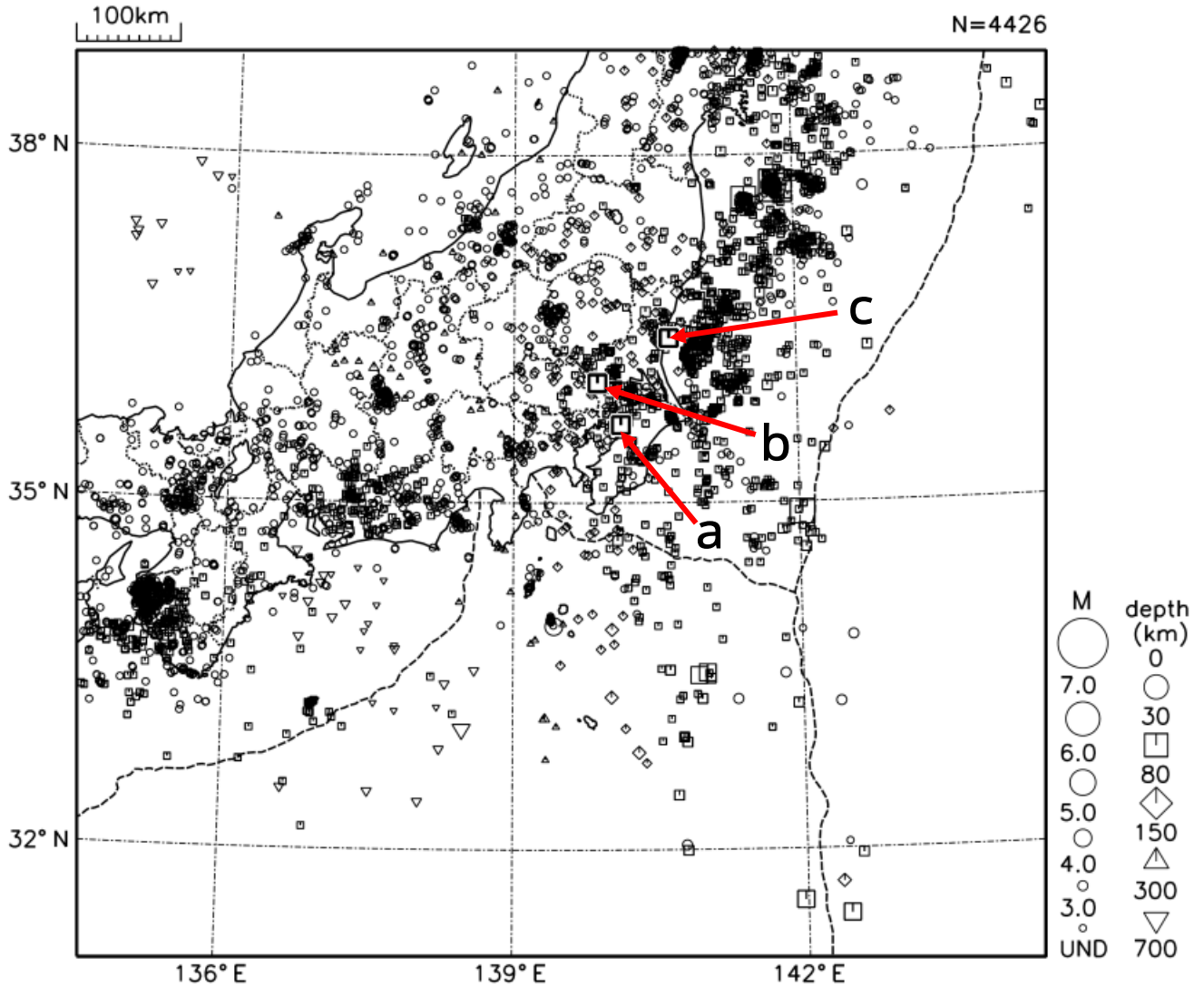
図 5 関東・中部地方の震央分布図（2010 年 3 月 1 日～ 3 月 31 日）
