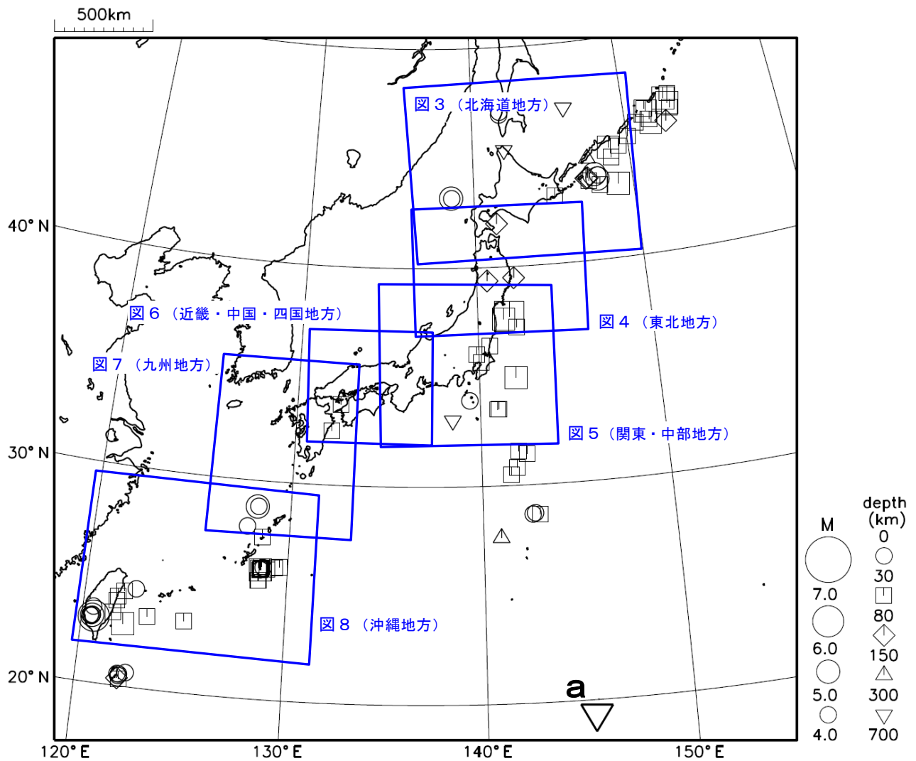
図 9 日本周辺で発生した主な地震の震央分布図（2010 年 3 月 1 日～3 月 31 日、 M \geq 4.0 ）
