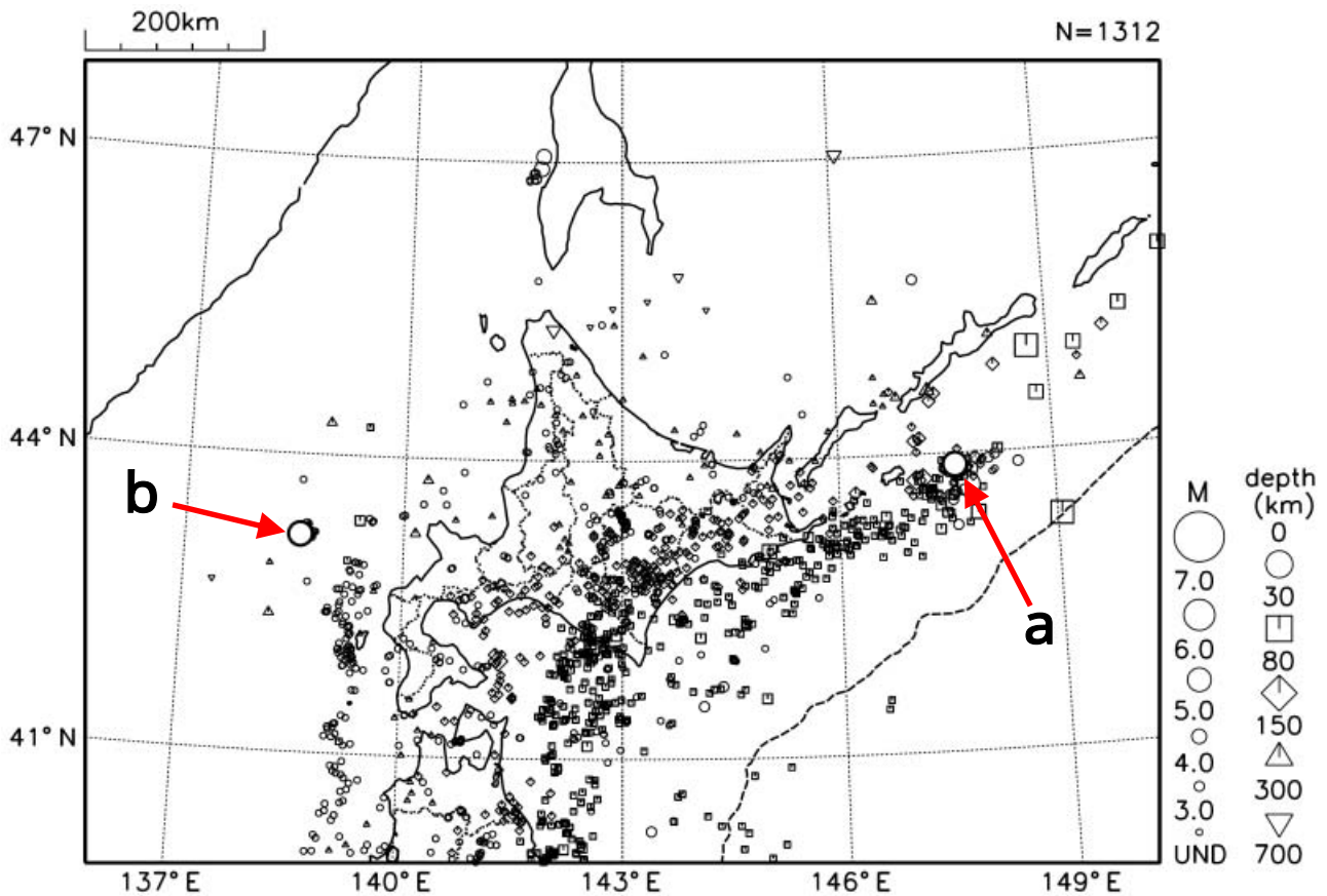
図3 北海道地方の震央分布図（2010年3月1日～3月31日）
