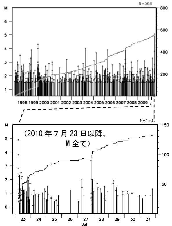
領域 b 内の M-T 図、回数積算図
