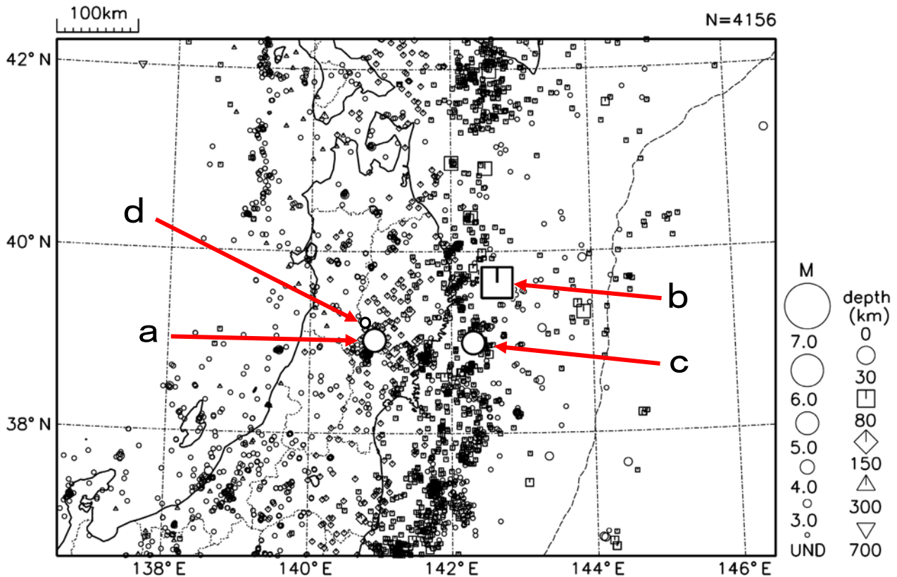
図 4 東北地方の震央分布図（2010 年 7 月 1 日～7 月 31 日）
