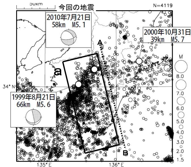
震央分布図 (1997 年 10 月 1 日～2010 年 7 月 31 日、 深さ 20～100km、 M \geq 1.5 )
