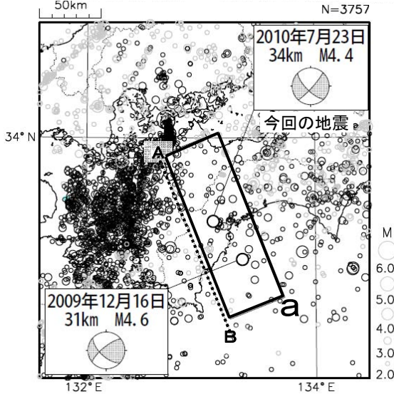
震央分布図 (1997 年 10 月 1 日～2010 年 7 月 31 日、 深さ 0～100km、 M \geq 2.0 ) 20km より深い地震を濃く表示
