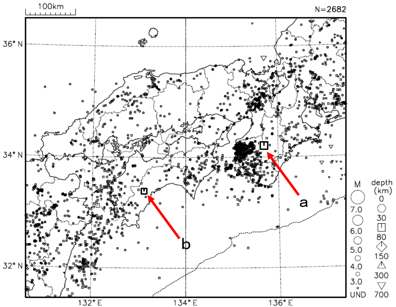
図6 近畿・中国・四国地方の震央分布図（2010年7月1日～7月31日）
