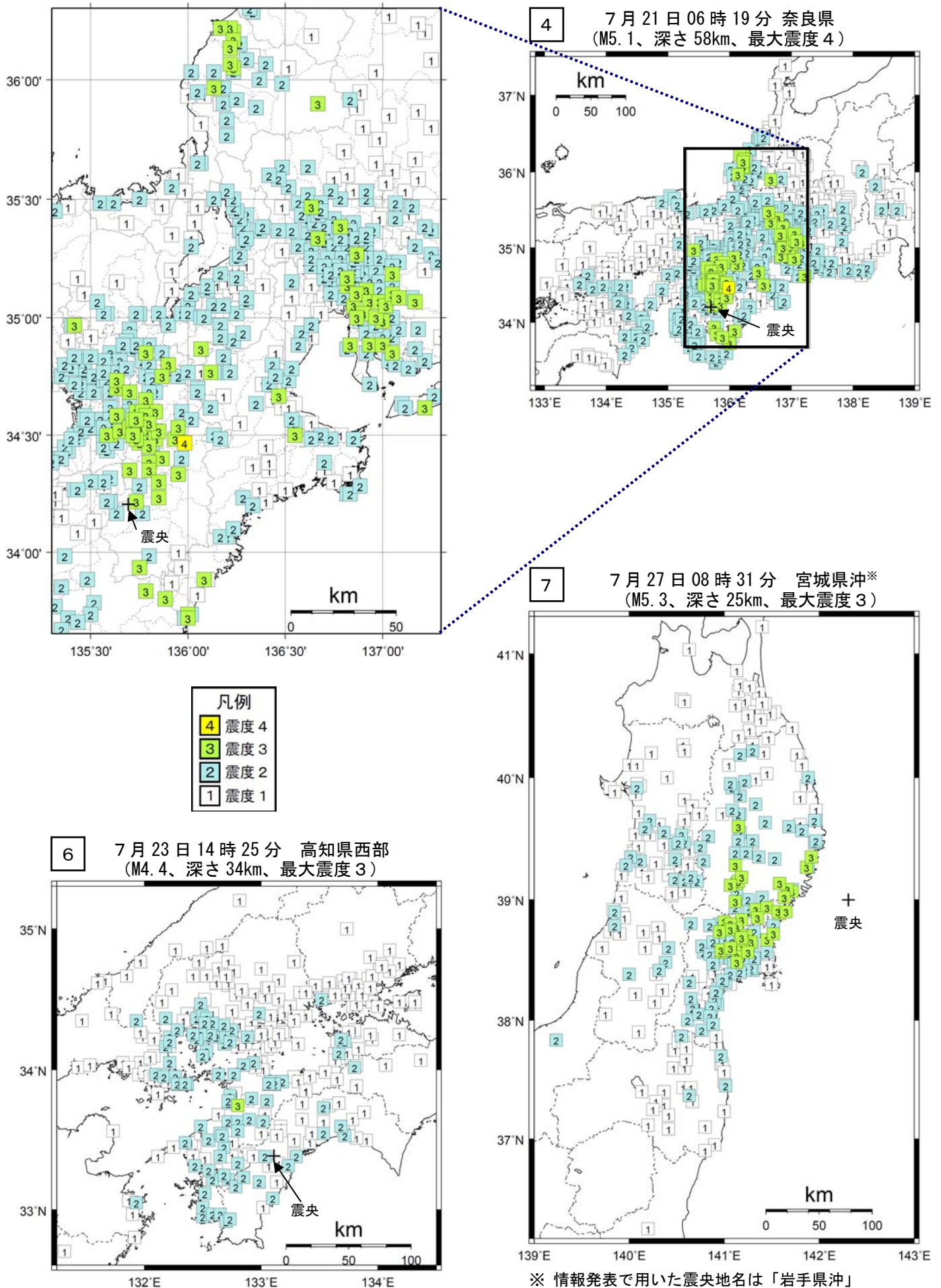
図 2-2 震度分布図（各図の左上の数字は表 1、図 1 の番号に対応する。＋印は震央を示す）
