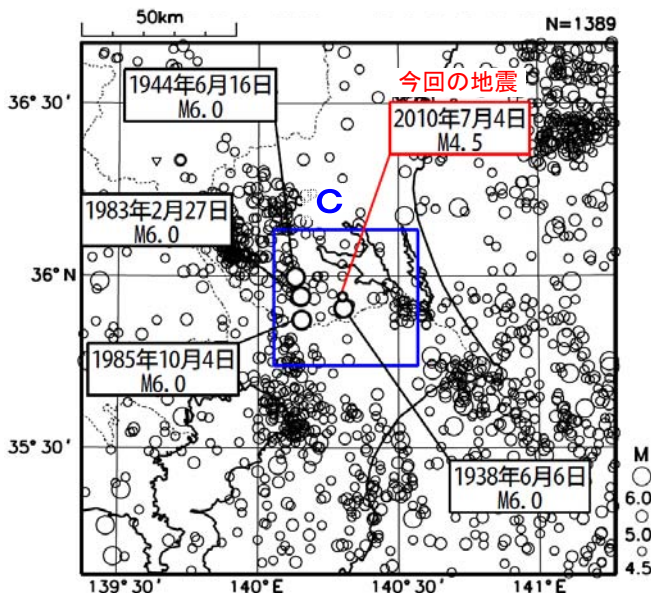
震央分布図 (1923 年 8 月 1 日～2010 年 7 月 31 日、 深さ 0～120km、 M \geq 4.5 )
