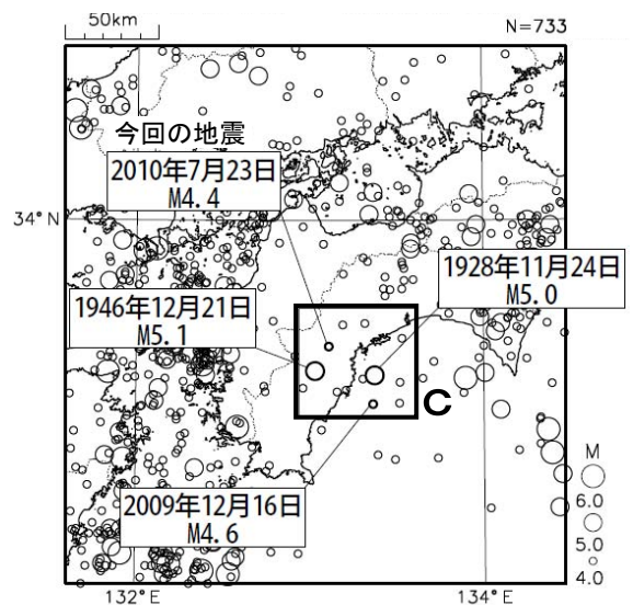
震央分布図 (1923 年 8 月 1 日～2010 年 7 月 31 日、 深さ 0～100km、 M \geq 4.0 )
