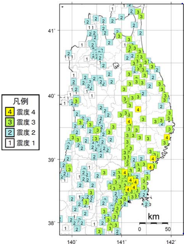
図 2 - 1 震度分布図（各図の左上の数字は表 1，図 1 の番号に対応する。+印は震央を示す）
