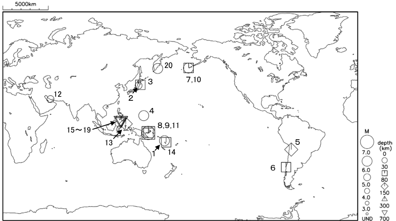
図 1 平成 22 年（2010 年）7 月に世界で発生した M6.0 以上または被害を伴った地震の震央分布
