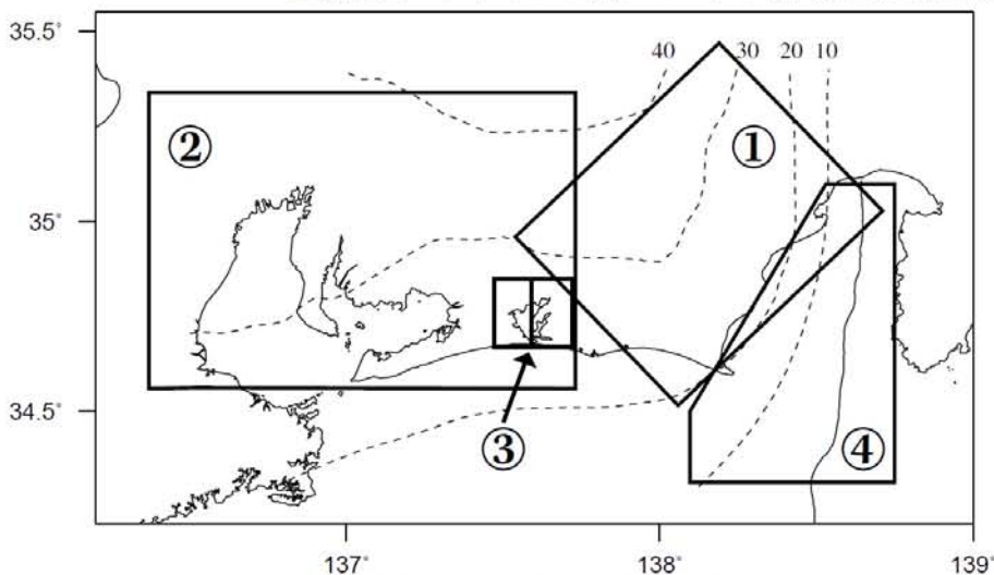
図2 東海地域の地震活動指数
