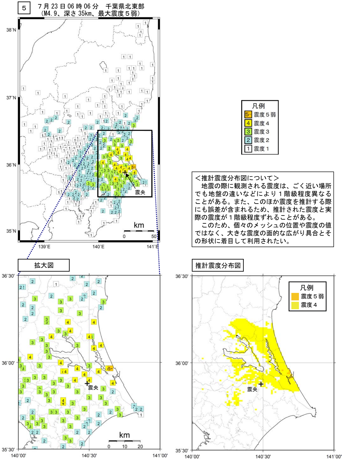
図2-3 震度分布図（各図の左上の数字は表1、図1の番号に対応する。+印は震央を示す）
