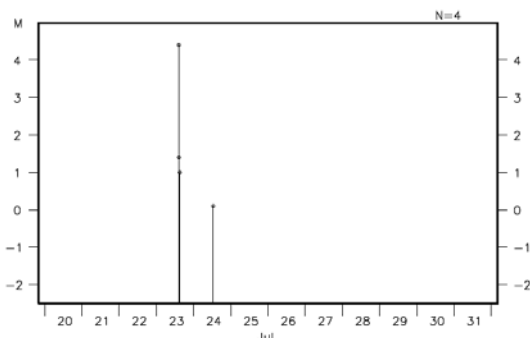
領域 b 内の M-T 図 (2010 年 7 月 20 日～7 月 31 日、M 全て)
