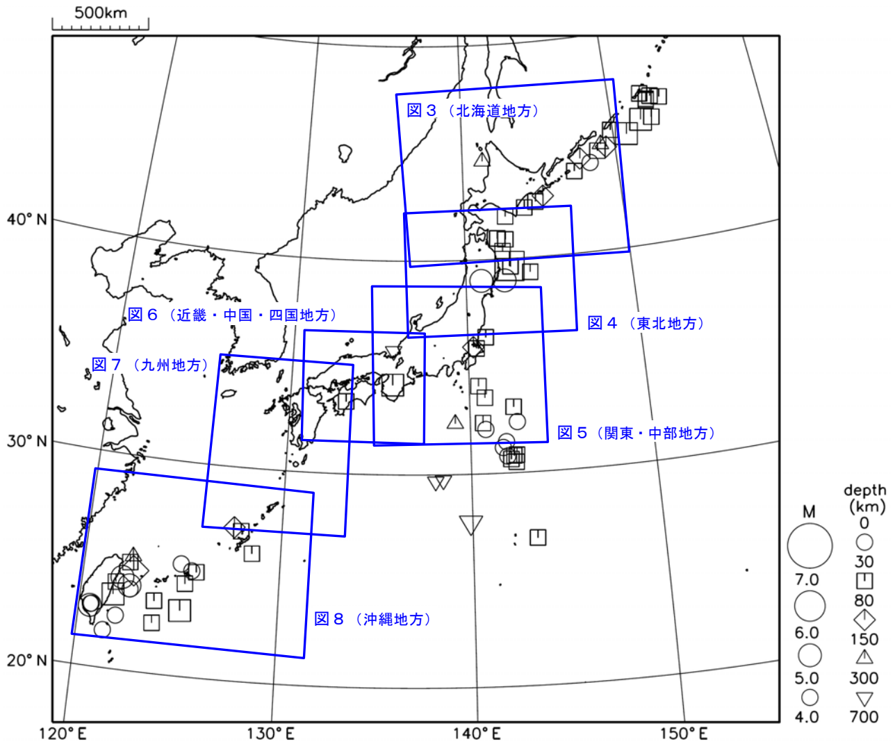
図9 日本周辺で発生した主な地震の震央分布図（2010年7月1日～7月31日、M≥4.0）
