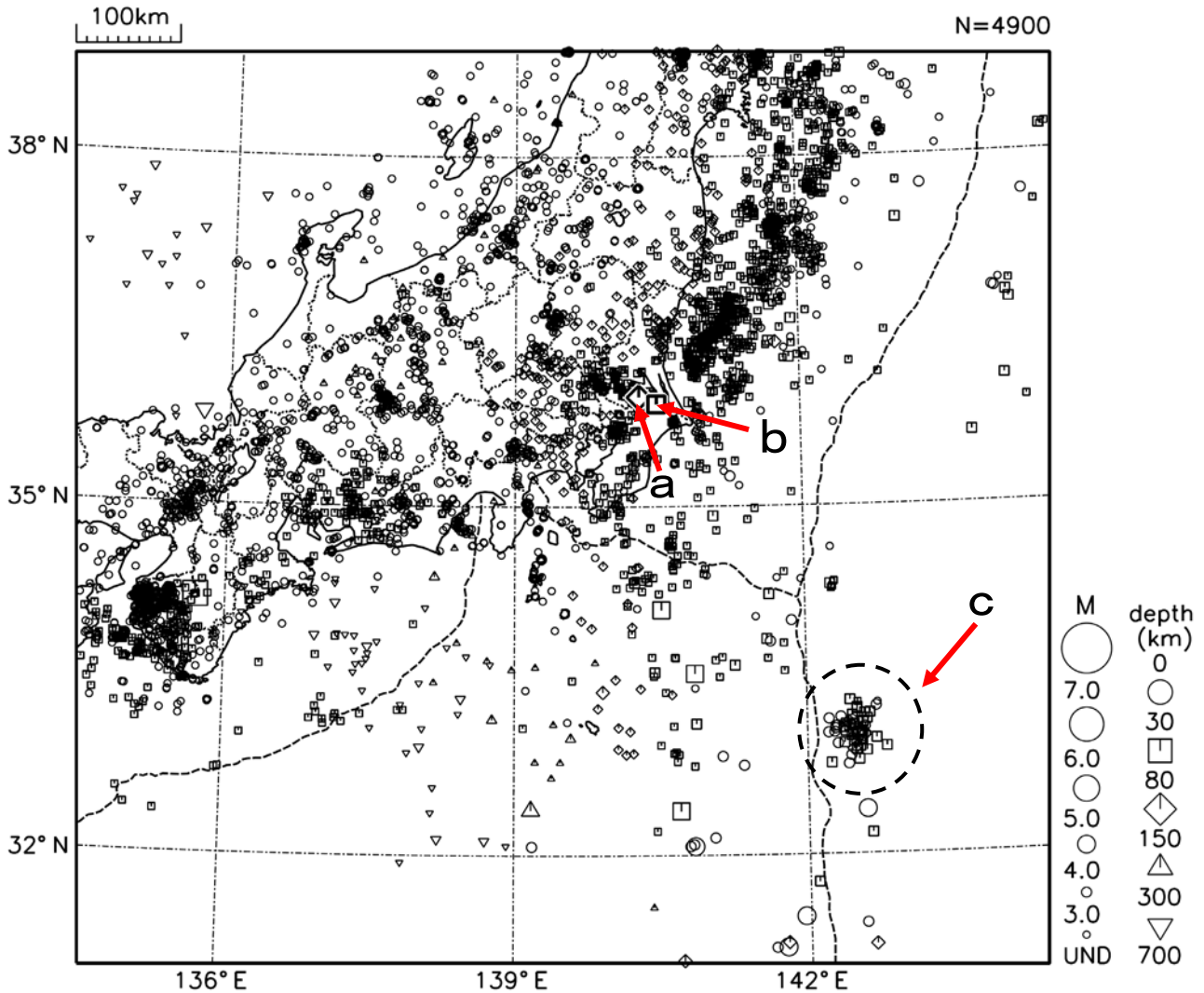
図5 関東・中部地方の震央分布図（2010年7月1日～7月31日）
