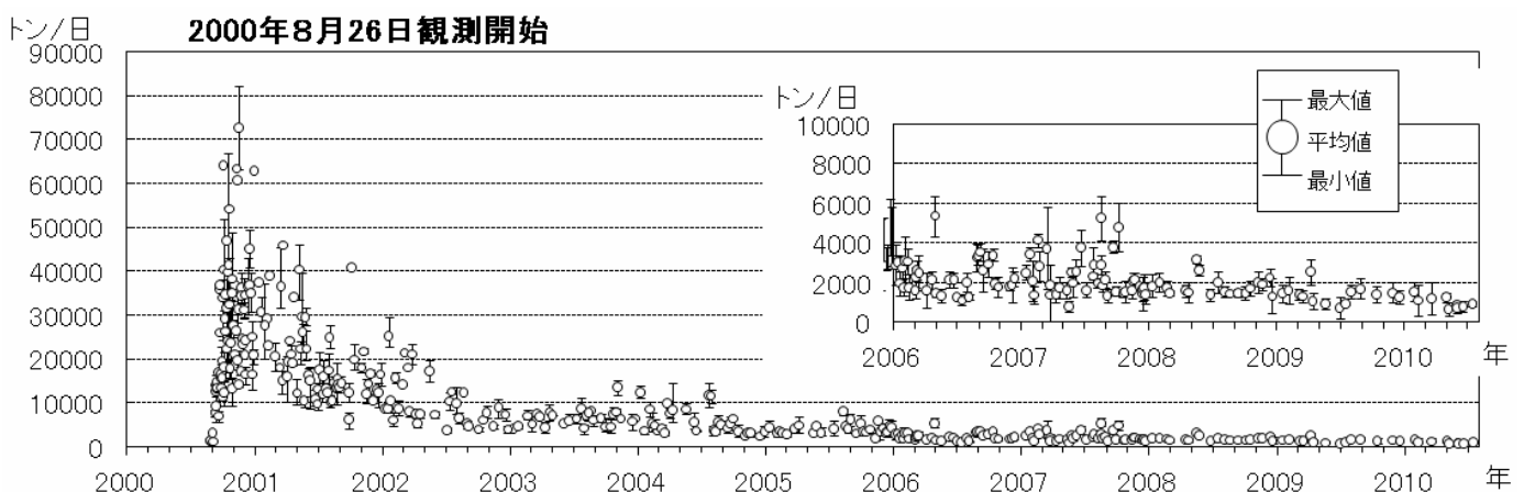
図 2 三宅島 二酸化硫黄の放出量 3) の推移（2000 年 8 月～2010 年 7 月）
