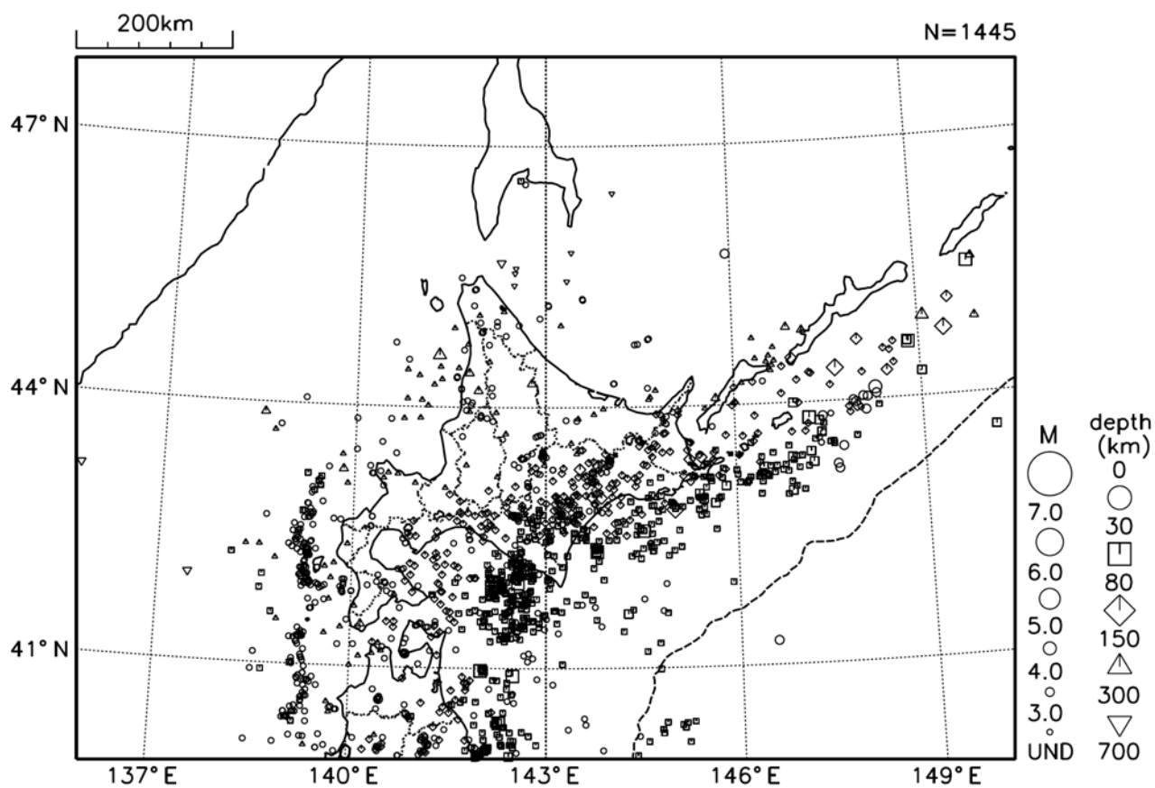
図3 北海道地方の震央分布図（2010年7月1日～7月31日）
