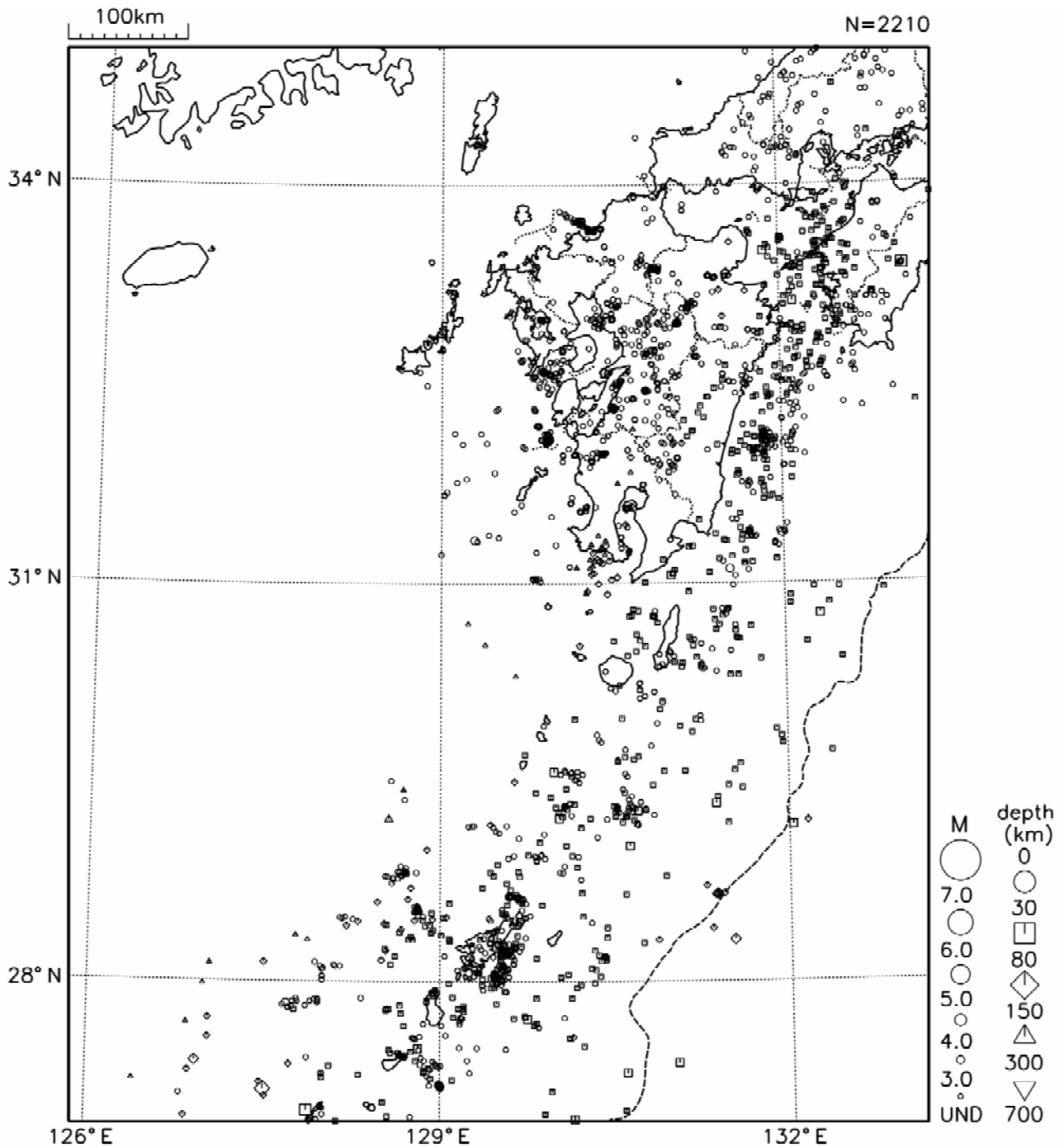
図7 九州地方の震央分布図（2010年7月1日～7月31日）
