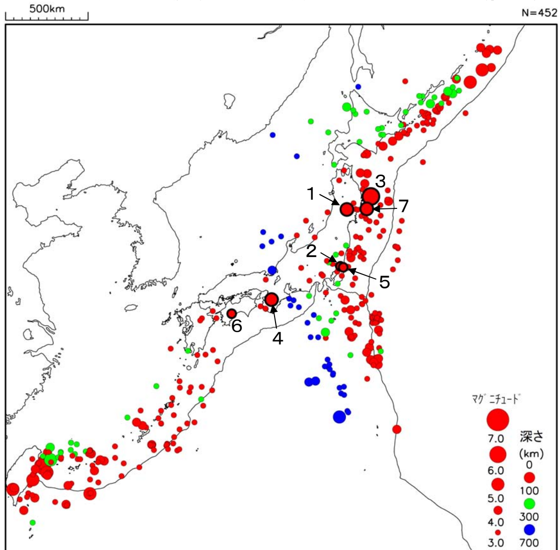
図 1 平成 22 年 7 月に日本及びその周辺で発生した M3.0 以上の地震の震央分布図（図中の数字は表 1 の番号に対応）
