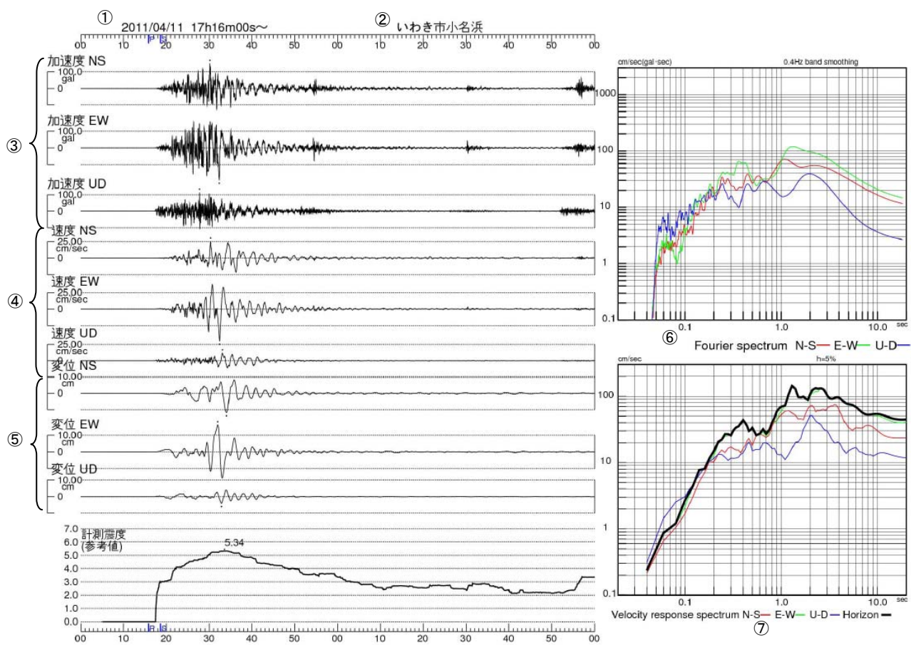
図 3-6 いわき市小名浜で観測した波形、加速度フーリエスペクトル及び速度応答スペクトル
