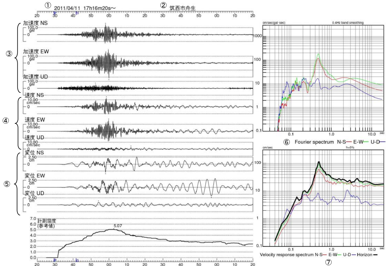
図 3-8 筑西市舟生で観測した波形、加速度フーリエスペクトル及び速度応答スペクトル
