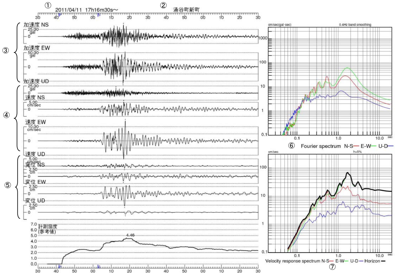
図 3-10 滝谷町新町で観測した波形、加速度フーリエスペクトル及び速度応答スペクトル
