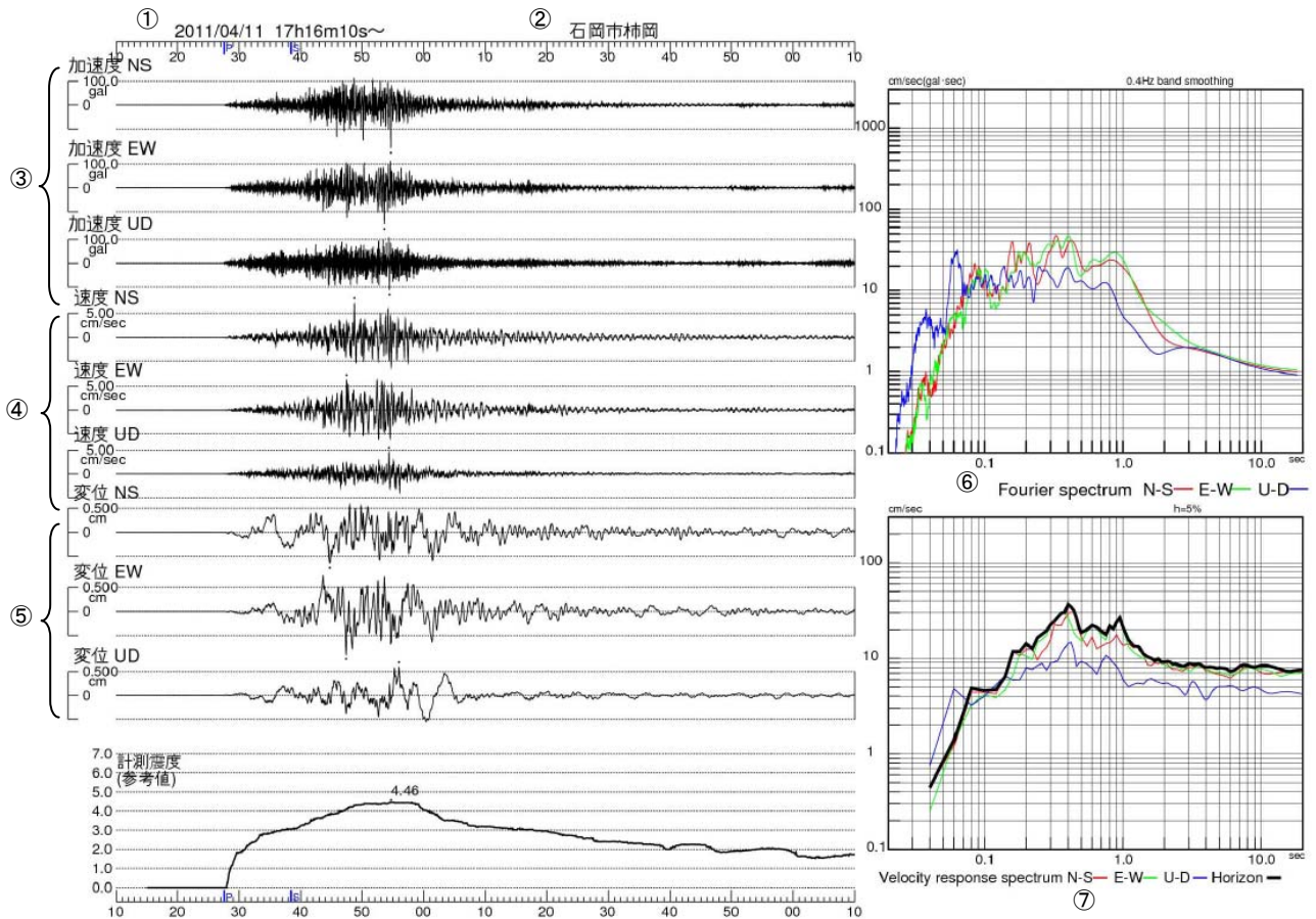
図 3-12 石岡市柿岡で観測した波形、加速度フーリエスペクトル及び速度応答スペクトル
