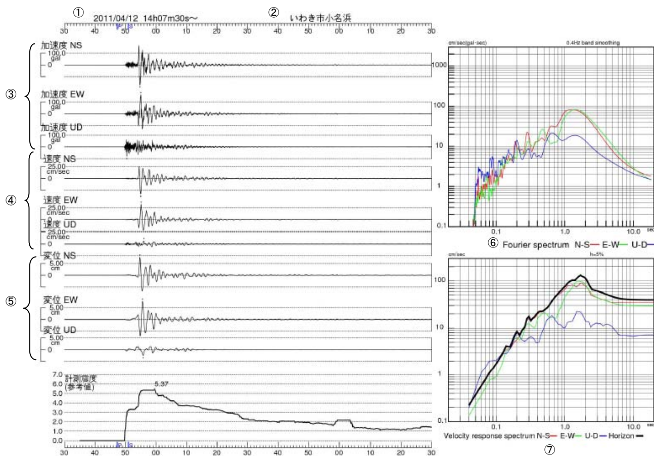
図 3-15 いわき市小名浜で観測した波形、加速度フーリエスペクトル及び速度応答スペクトル
