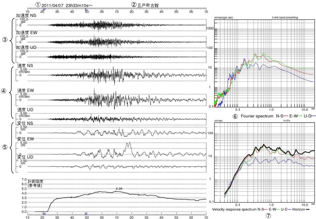
図 2-11 五戸町古館で観測した波形、加速度フーリエスペクトル及び速度応答スペクトル
