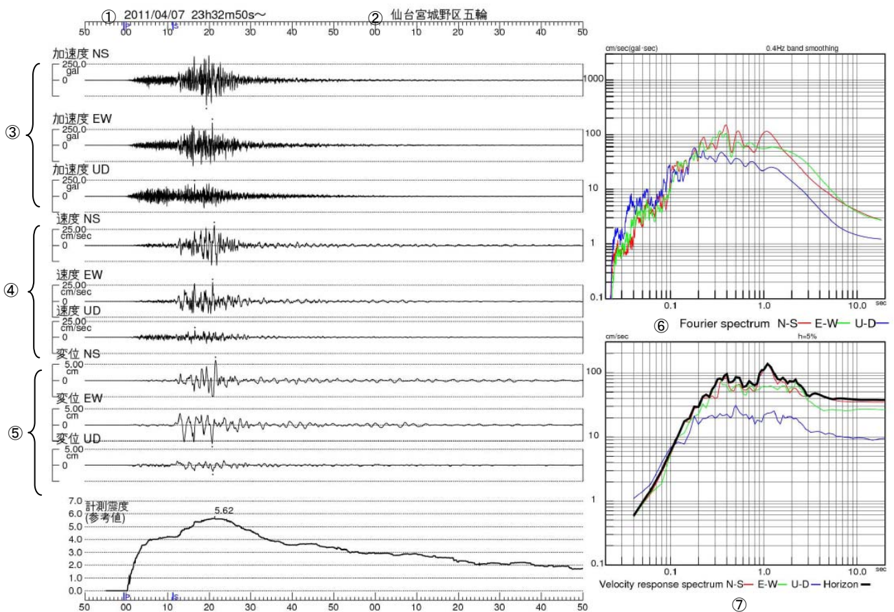
図 2-9 仙台宮城野区五輪で観測した波形、加速度フーリエスペクトル及び速度応答スペクトル
