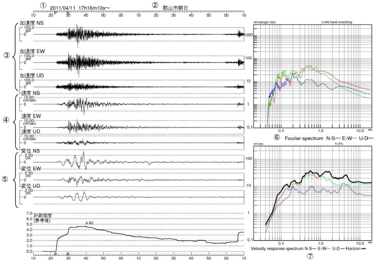
図 3-11 郡山市朝日で観測した波形、加速度フーリエスペクトル及び速度応答スペクトル
