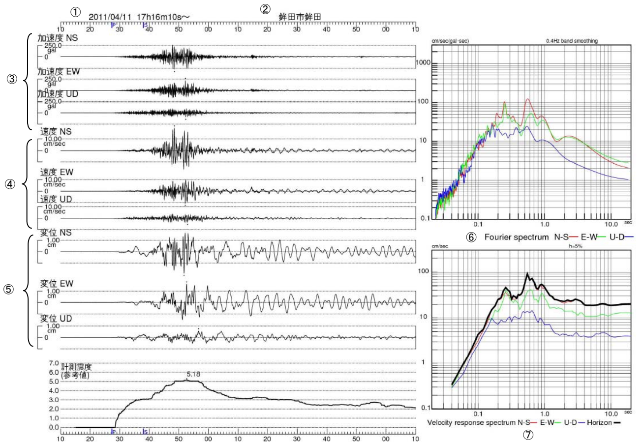
図 3-9 鉾田市鉾田で観測した波形、加速度フーリエスペクトル及び速度応答スペクトル
