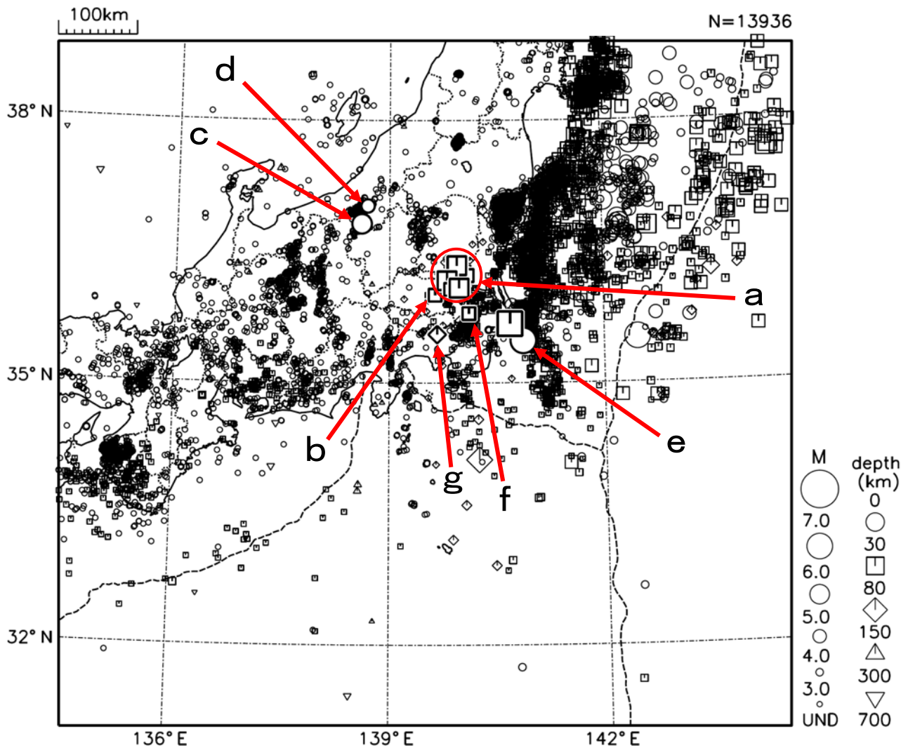
図6 関東・中部地方の震央分布図（2011年4月1日～4月30日） （「平成23年（2011年）東北地方太平洋沖地震」の余震域で発生した地震について 処理の遅れのため掲載されていないものがある）
