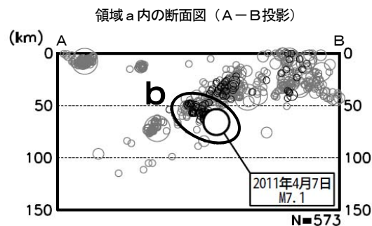
図 2-1-1 震央分布図および領域 a 内の断面図 （1997 年 10 月 1 日～2011 年 4 月 30 日、 M \geq 4.0、深さ 0～150km） 2011 年 4 月以降の地震を濃く表示
