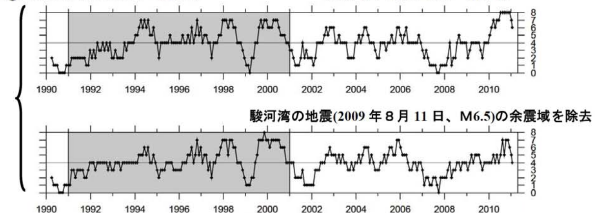
図 3 東海地域の地震活動指数の推移
