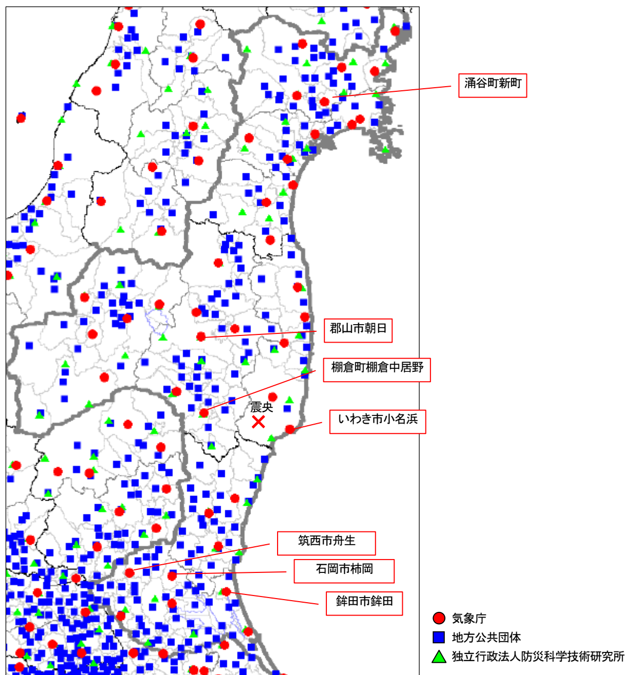
図 3-5 図 3-6～12 で波形等を示している観測点の位置
