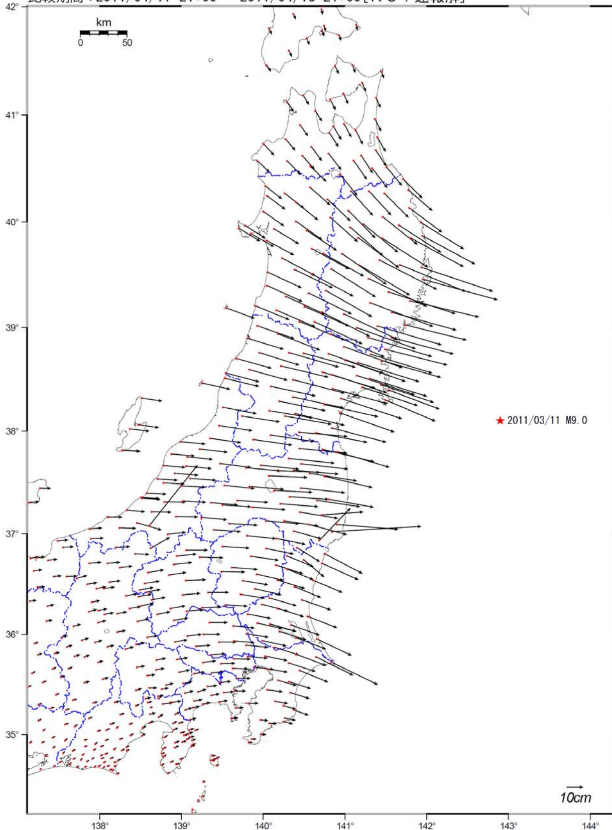
図7 「平成 23 年（2011 年）東北地方太平洋沖地震」後の水平地殻変動（余効変動） 国土地理院資料
