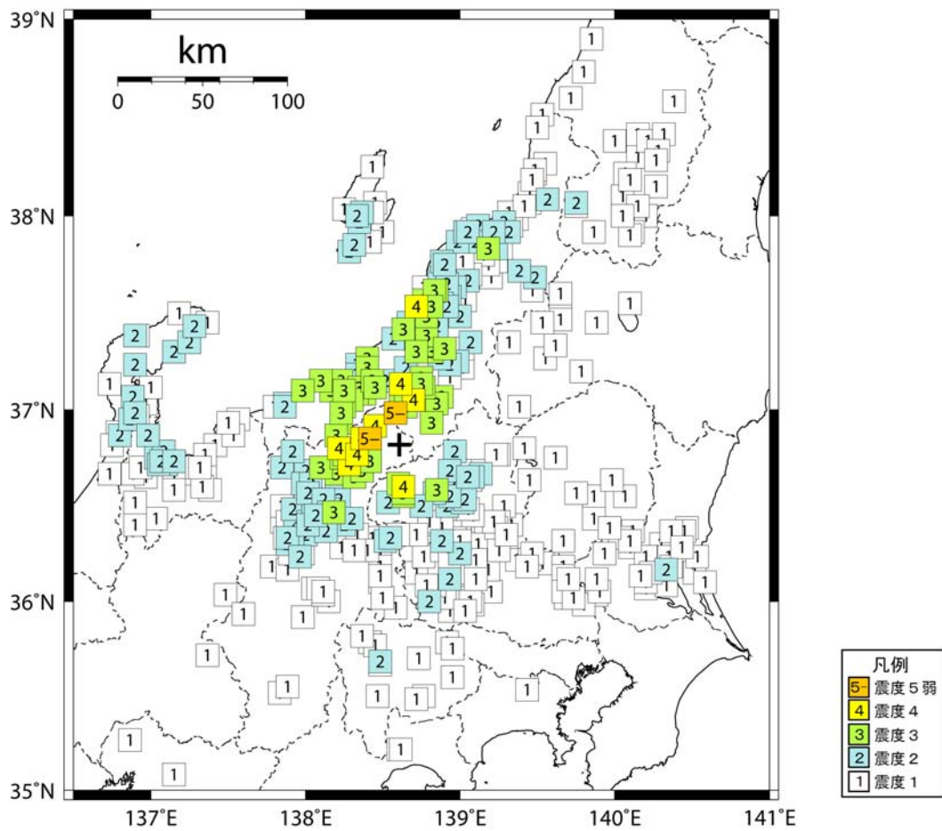
14 4 月 12 日 07 時 26 分 長野県・新潟県県境付近 (M5.6、ごく浅い、最大震度 5 弱)
