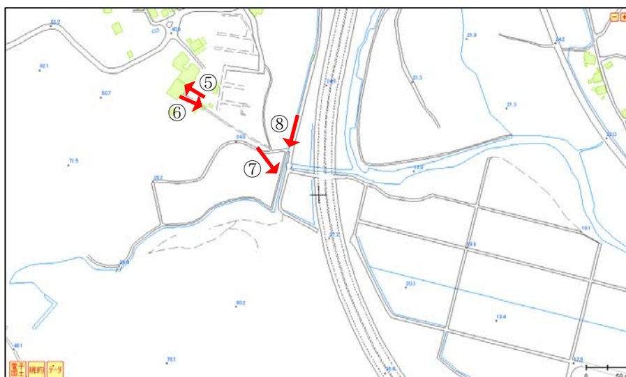
図 3-26 湯ノ岳断層付近調査地点（いわき市常磐藤原町）
