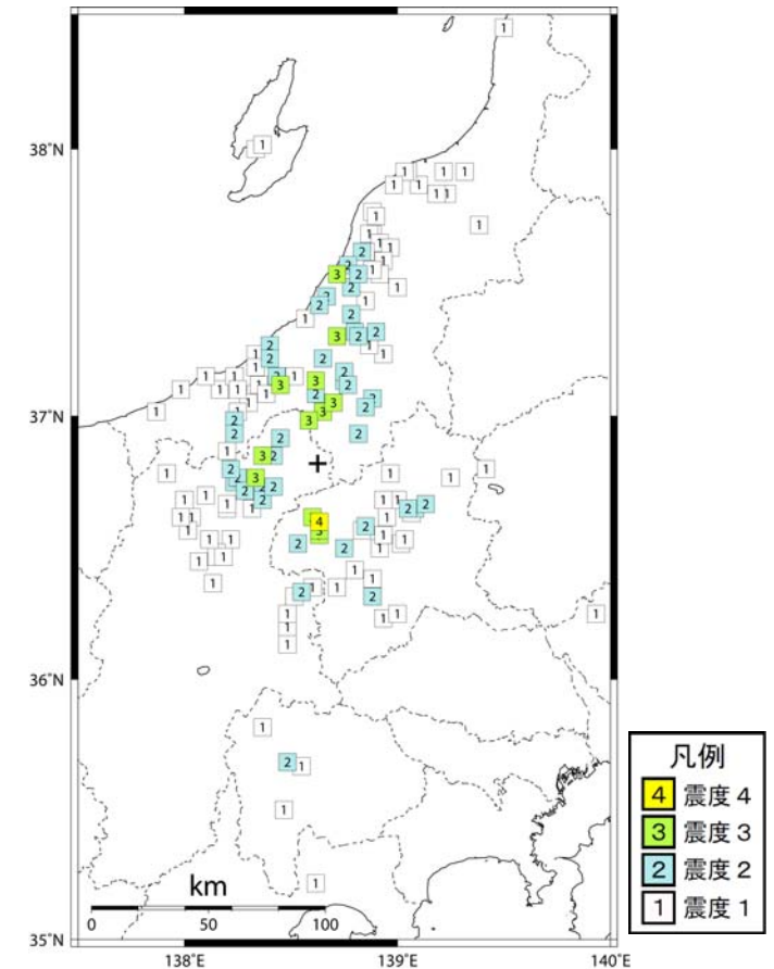
図 3-6 震度分布図（各図の左上の数字は表 1，図 2 の番号に対応する。+印は震央を示す）
