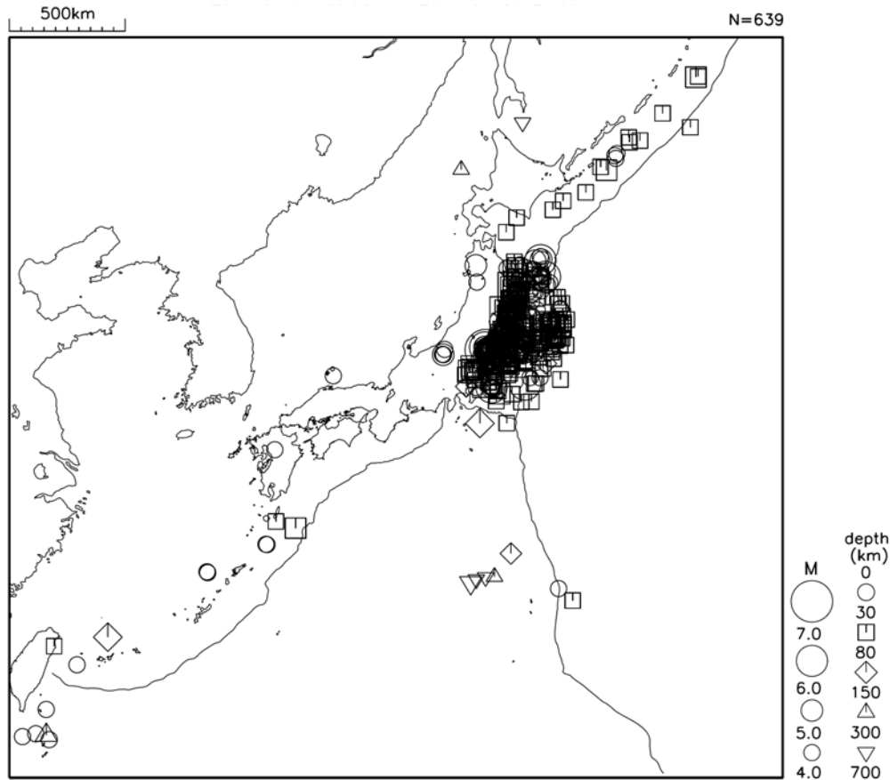
図 1 平成 23 年 4 月に日本及びその周辺で発生した M4.0 以上の地震の震央分布図 （「平成 23 年（2011 年）東北地方太平洋沖地震」の余震域で発生した地震について 処理の遅れのため掲載されていないものがある）
