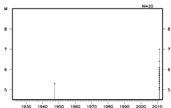
図 3-2-2 領域 b 内の M-T 図
