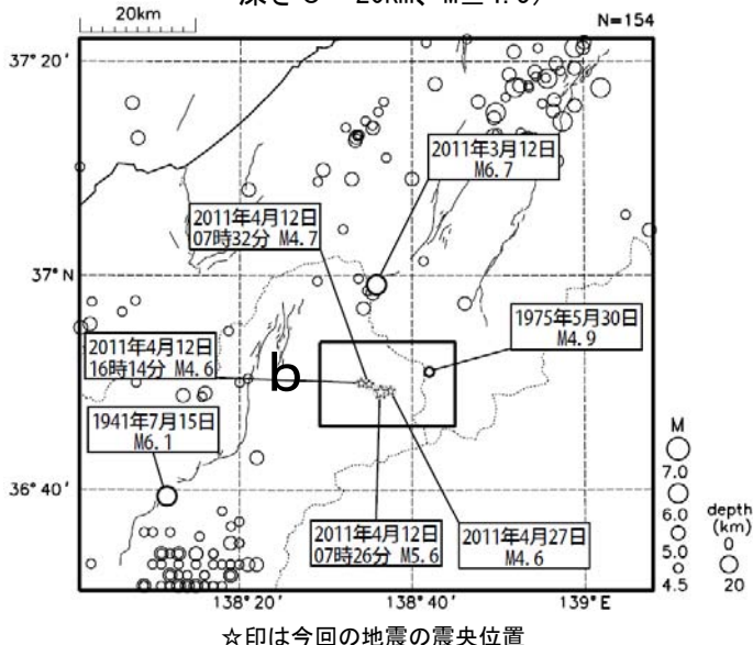
震央分布図（1923 年 8 月 1 日～2011 年 4 月 30 日、 深さ 0～20km、 M \geq 4.5 ）
