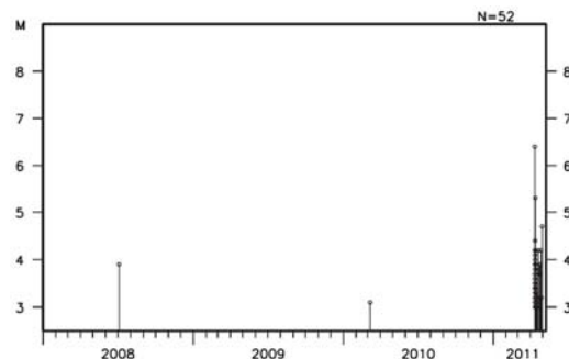
(2008年1月1日～4月30日、深さ0～100km、 M \geq 3.0 )
