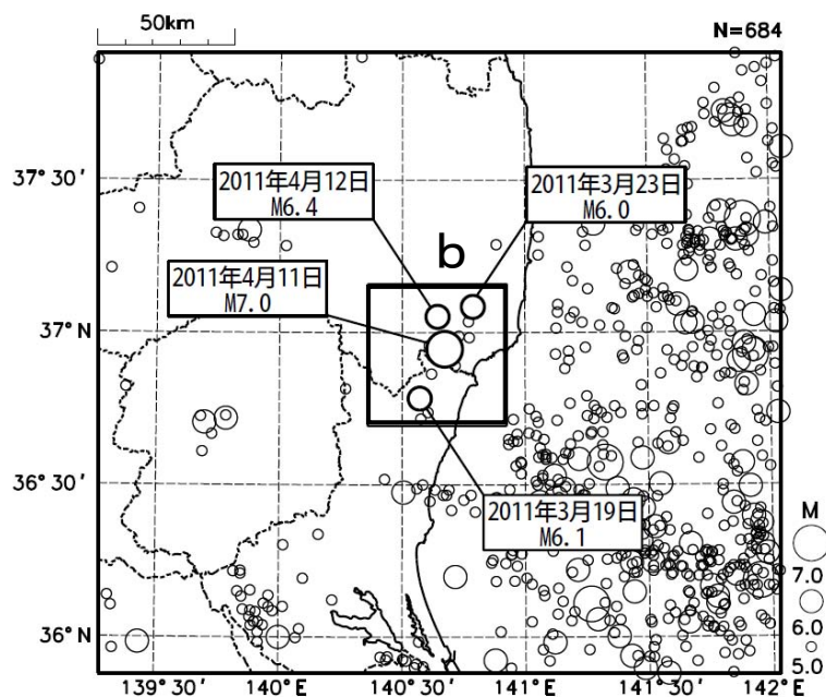
図 3-2-1 震央分布図 (1923 年 8 月 1 日～2011 年 4 月 30 日、 深さ 0～50km、 M \geq 5.0 )
