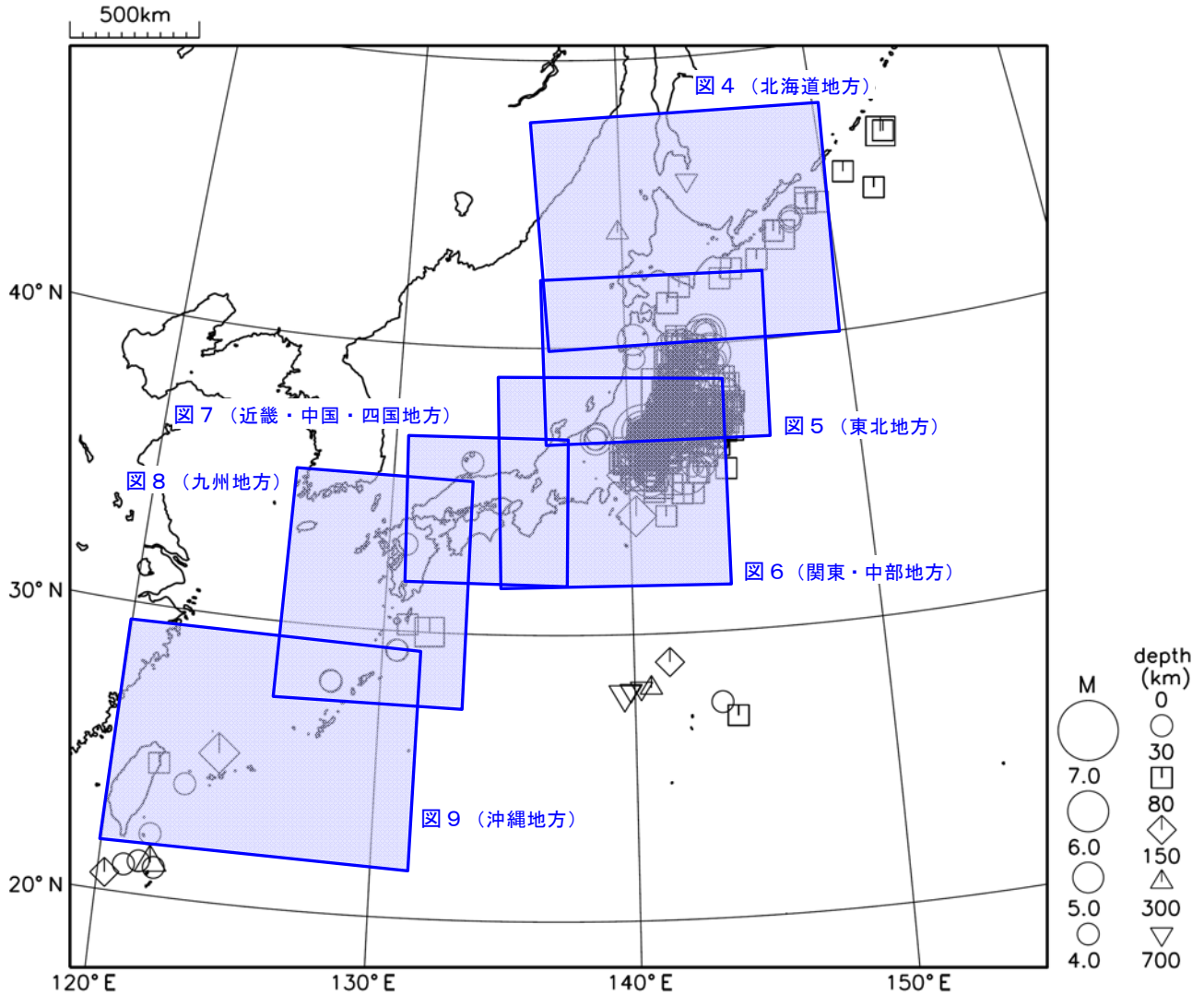
図 10 日本周辺で発生した主な地震の震央分布図（2011 年 4 月 1 日～4 月 30 日、 M \geq 4.0 ）
