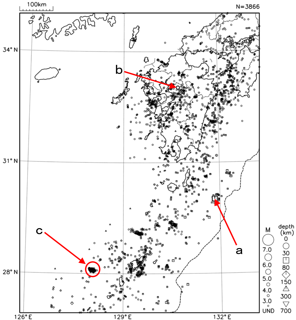
図 8 九州地方の震央分布図（2011 年 4 月 1 日～4 月 30 日）
