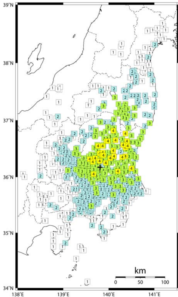
図 3－5 震度分布図（各図の左上の数字は表 1，図 2 の番号に対応する。＋印は震央を示す）
