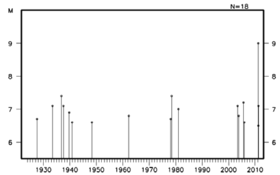
図 2-2-2 領域 c 内の M-T 図
