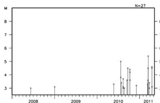
(2008年1月1日～4月30日、深さ0～100km、 M \geq 3.0 )
