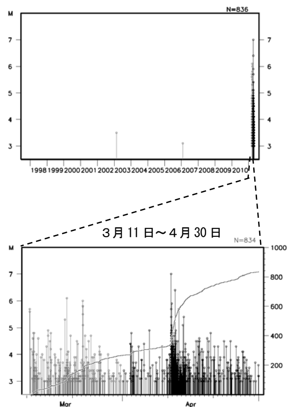
図 3-1-2 領域 a 内の M-T 図及び回数積算図
