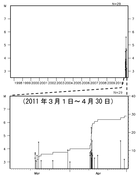
領域 a 内の M-T 図、回数積算図
