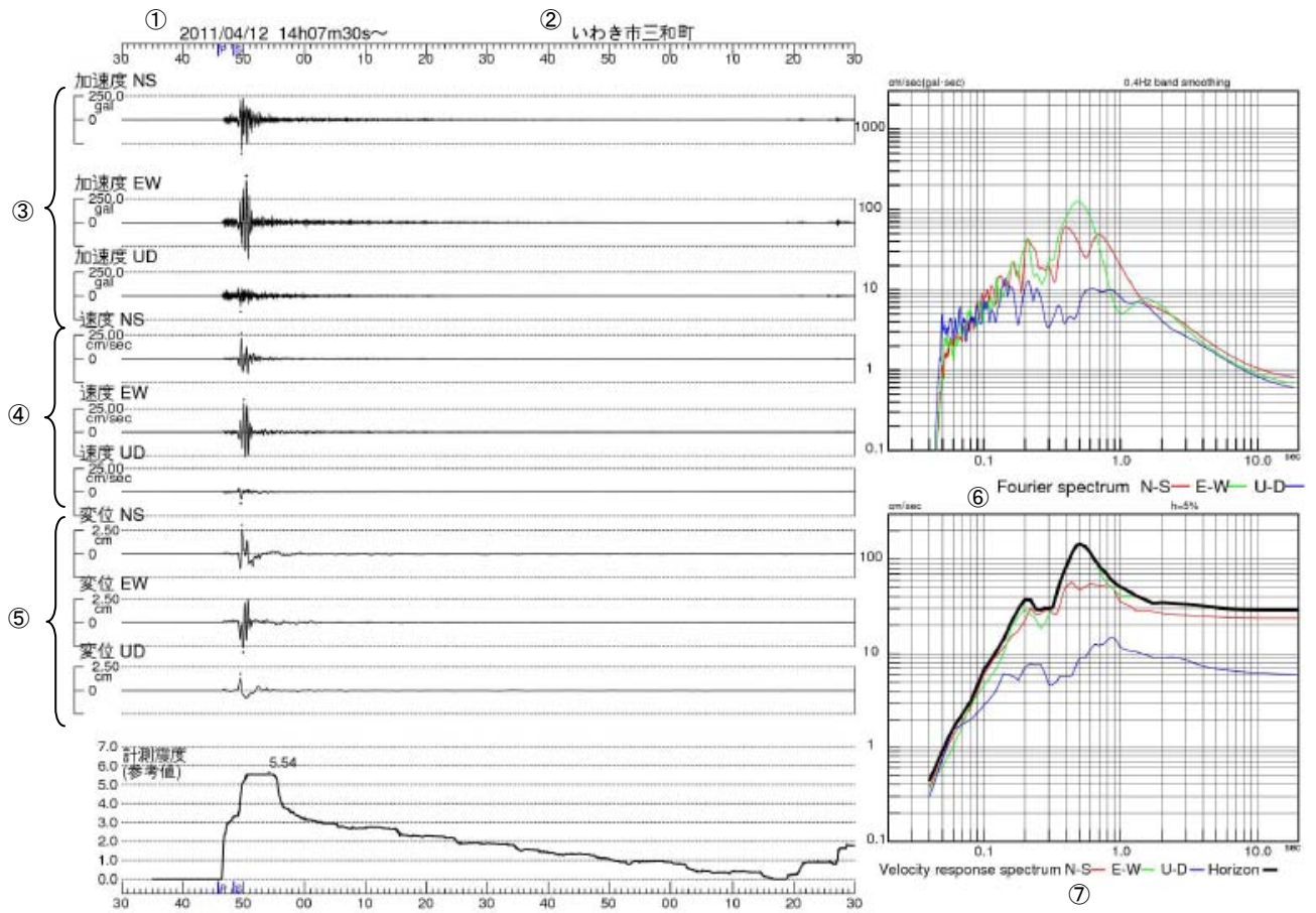
図 3-14 いわき市三和町で観測した波形、加速度フーリエスペクトル及び速度応答スペクトル
