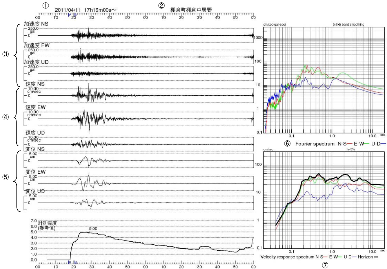
図 3-7 棚倉町棚倉中居野で観測した波形、加速度フーリエスペクトル及び速度応答スペクトル
