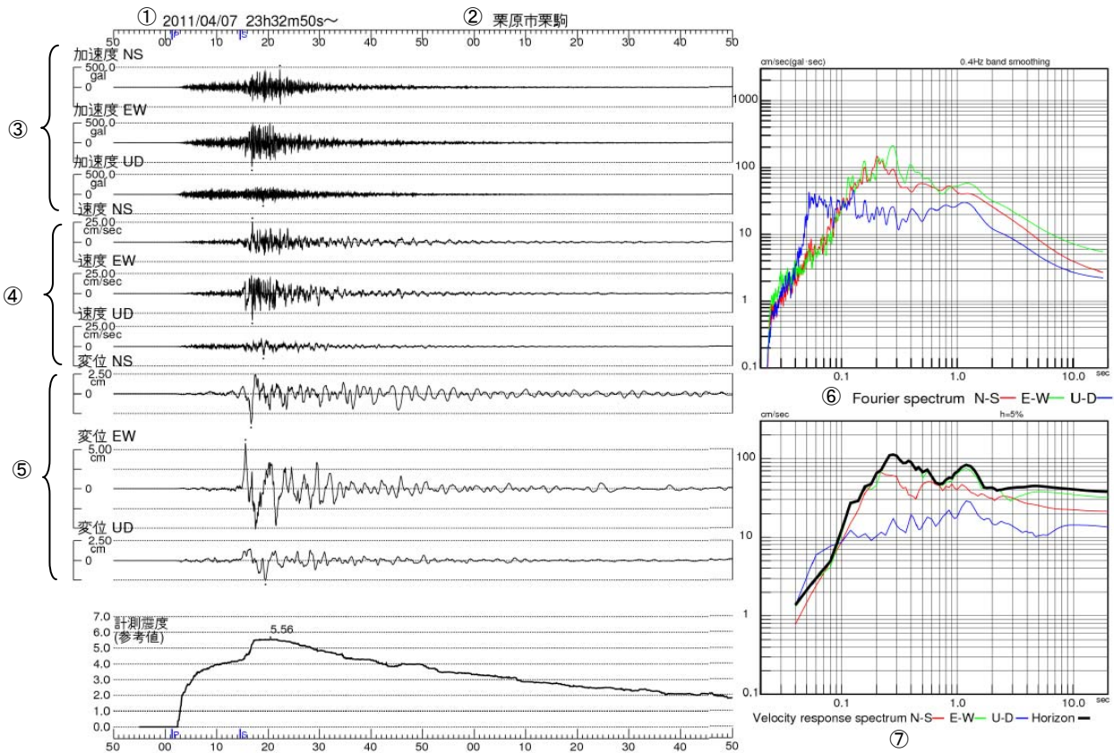
図 2-8 栗原市栗駒で観測した波形、加速度フーリエスペクトル及び速度応答スペクトル
