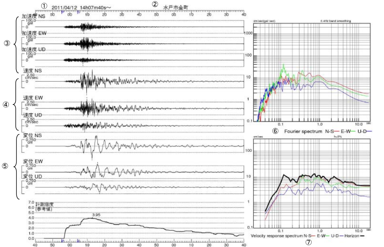
図 3-17 水戸市金町で観測した波形、加速度フーリエスペクトル及び速度応答スペクトル
