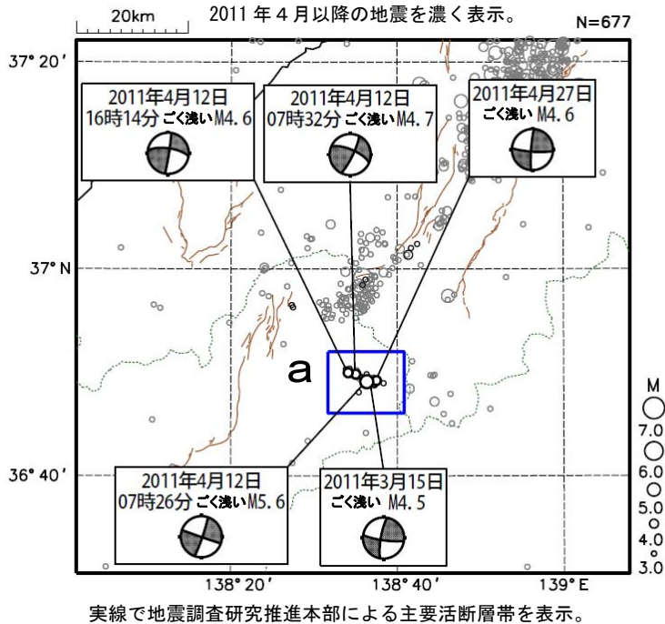
震央分布図（1997 年 10 月 1 日～2011 年 4 月 30 日、 深さ 0～20km、 M \geq 3.0 ）
