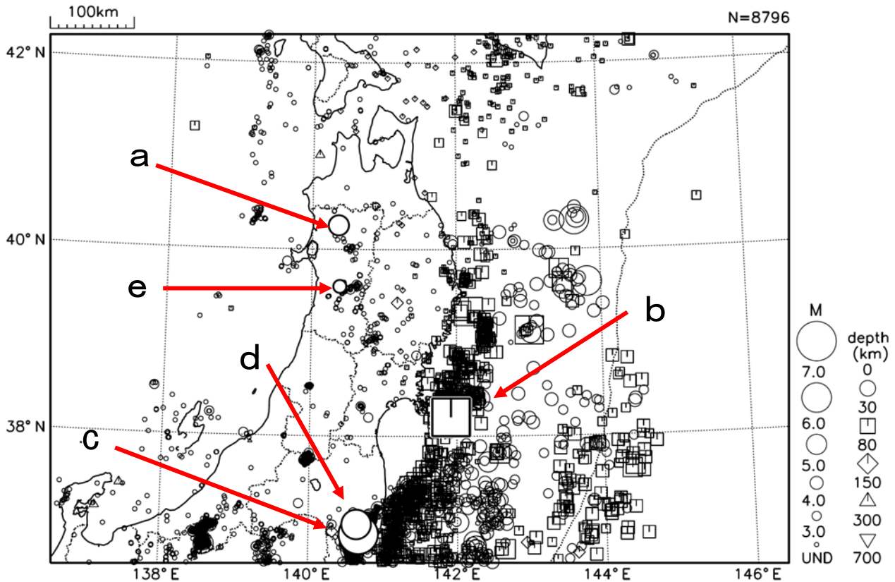
図5 東北地方の震央分布図（2011年4月1日～4月30日） （「平成23年（2011年）東北地方太平洋沖地震」の余震域で発生した地震について 処理の遅れのため掲載されていないものがある）
