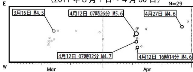
領域 a 内の時空間分布図（東西投影） （2011 年 3 月 1 日～4 月 30 日）
