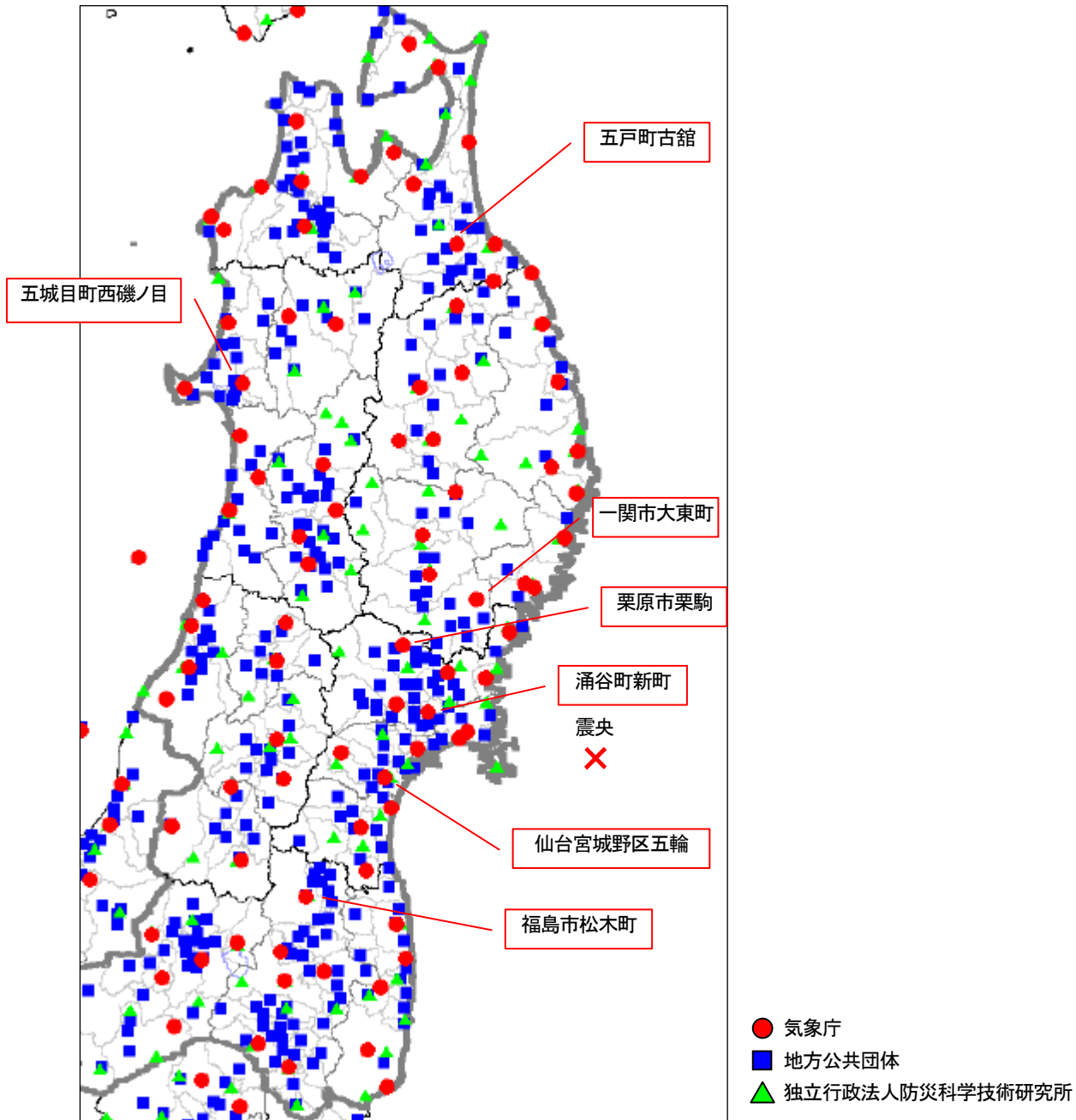
図 2-6 図 2-7～13 で波形等を示している観測点の位置
