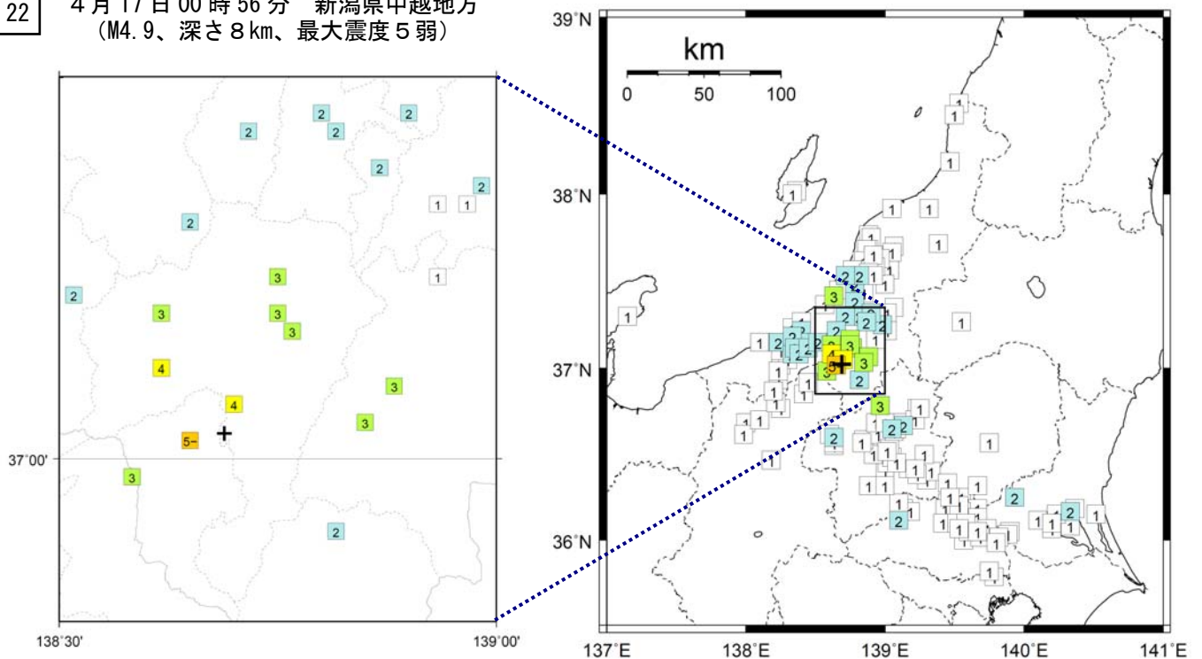
図 3-4 震度分布図（各図の左上の数字は表 1，図 2 の番号に対応する。+印は震央を示す）
