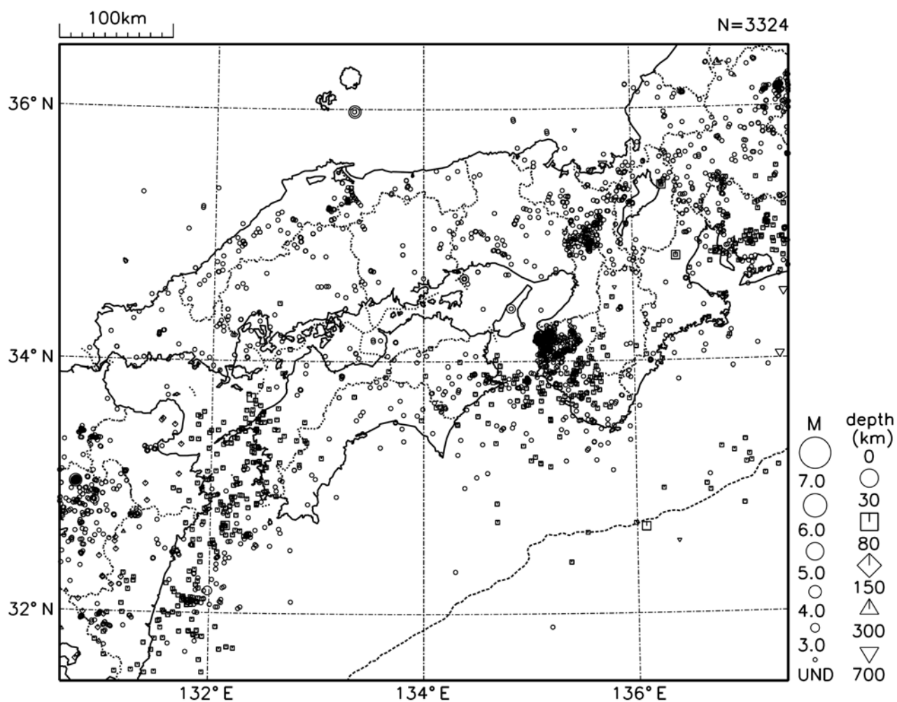
図 7 近畿・中国・四国地方の震央分布図（2011 年 4 月 1 日～4 月 30 日）
