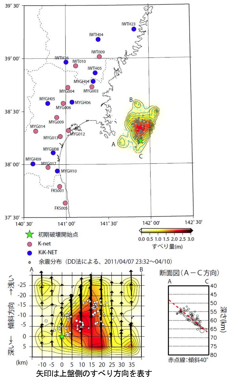
図 2-3 震源過程解析から推定された、断層面上のすべり量分布
