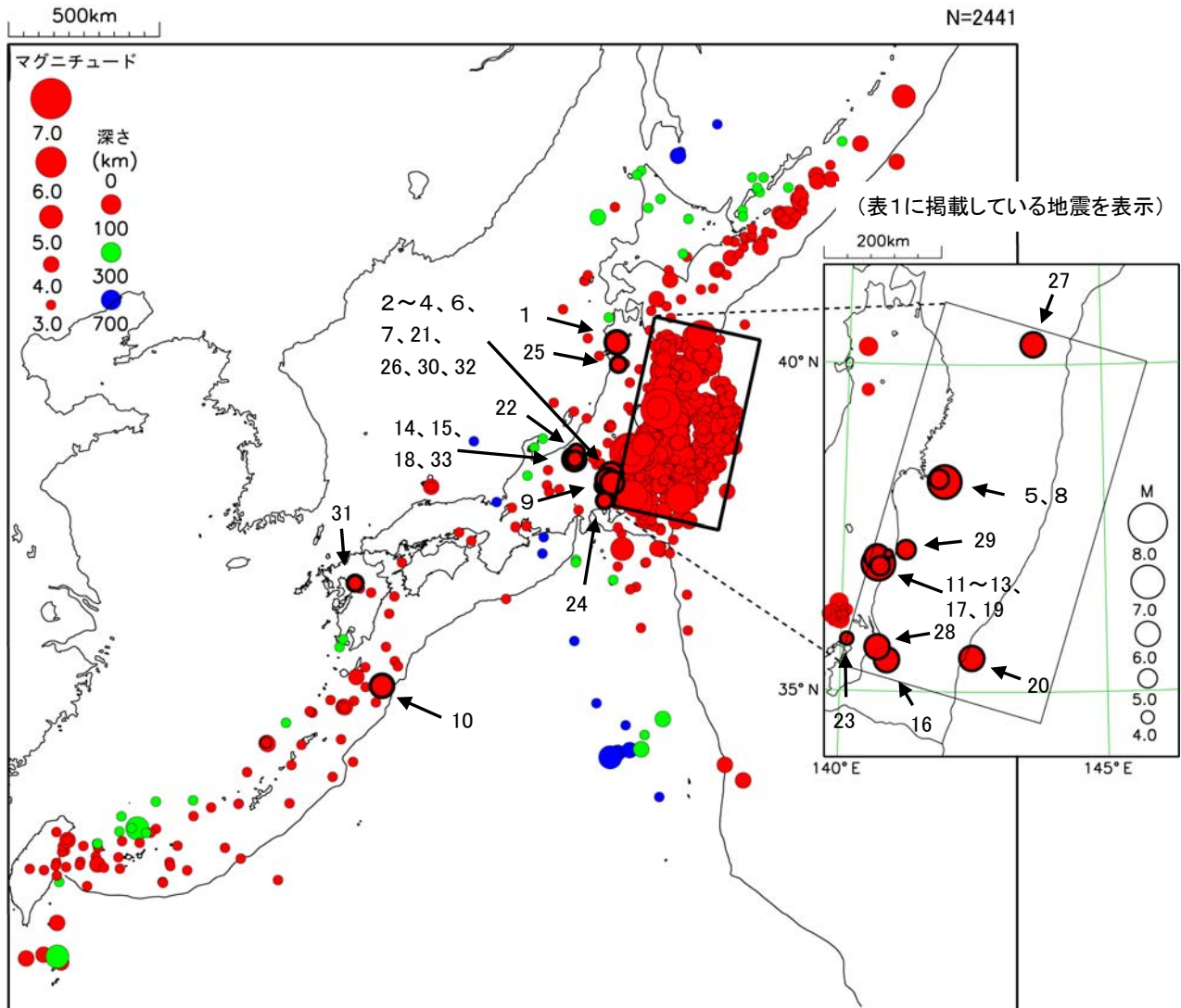
図 2 平成 23 年 4 月に日本及びその周辺で発生した M3.0 以上の地震の震央分布図
