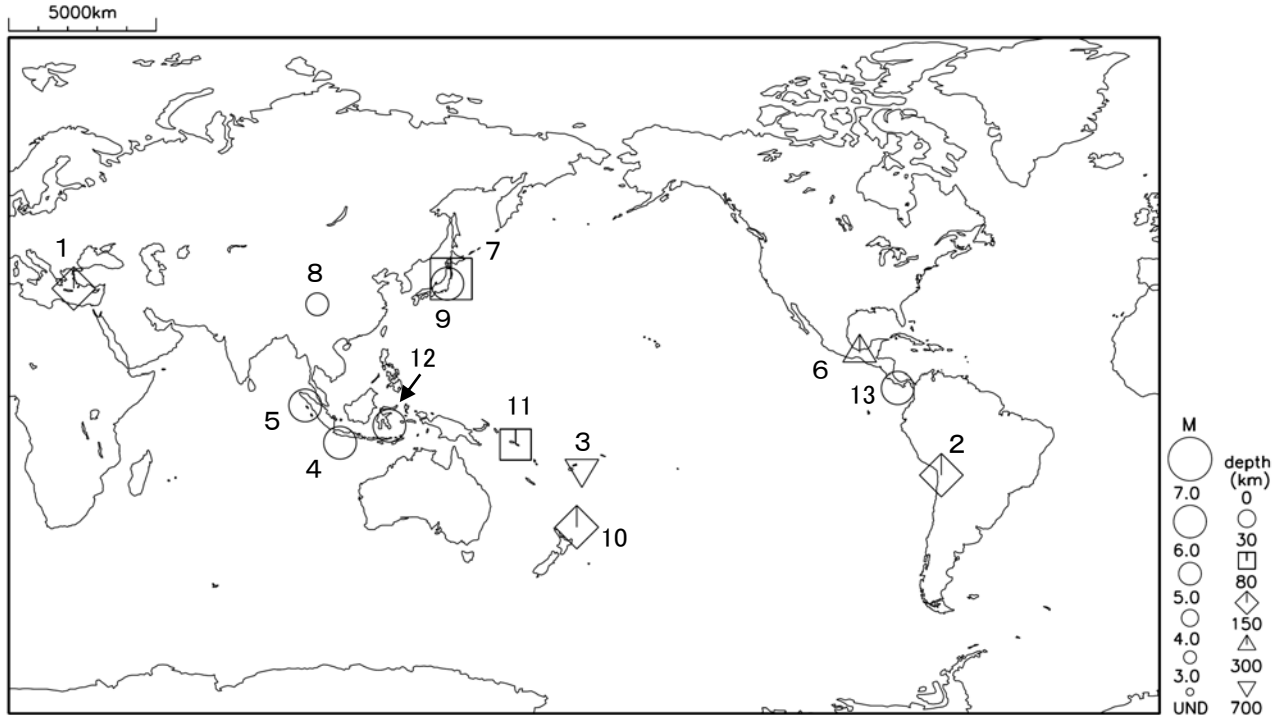
図 1 平成 23 年（2011 年）4 月に世界で発生した M6.0 以上または被害を伴った地震の震央分布
