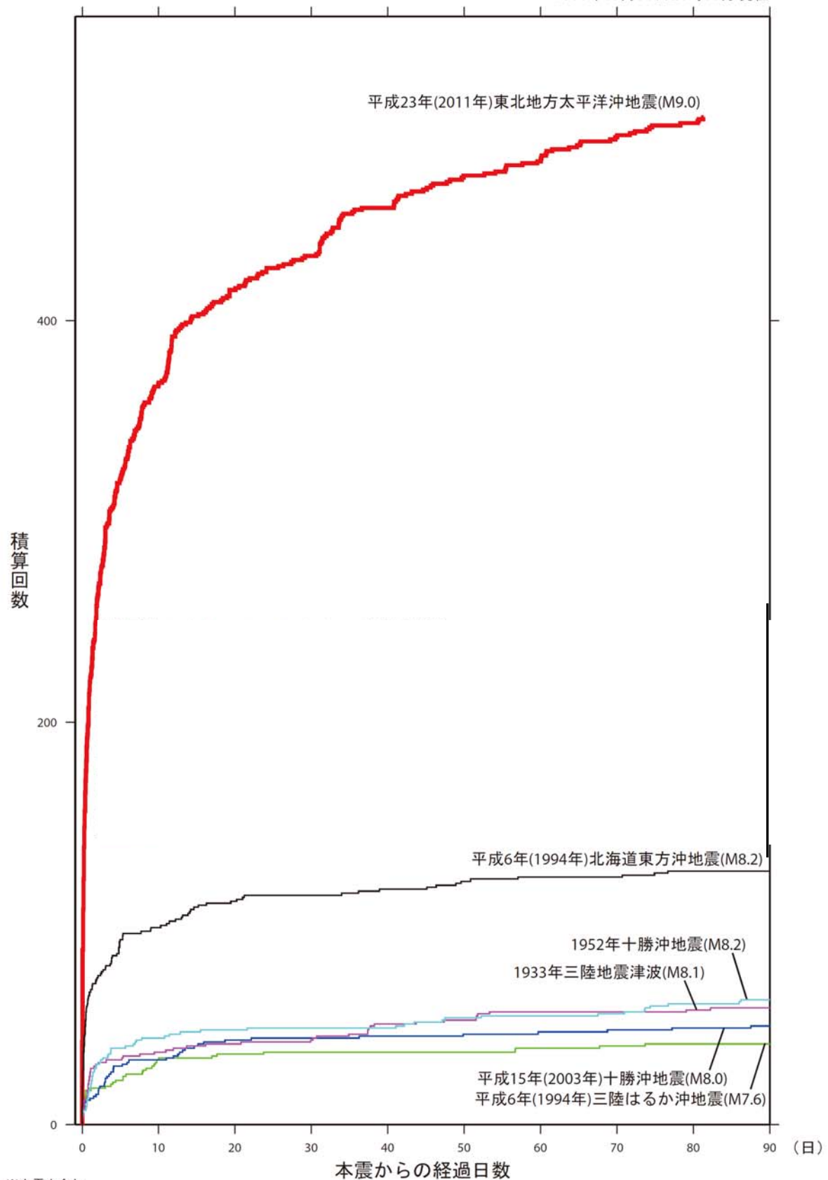
図1 海域で発生した主な地震の余震回数比較（※本震を含む：マグニチュード5.0以上）
