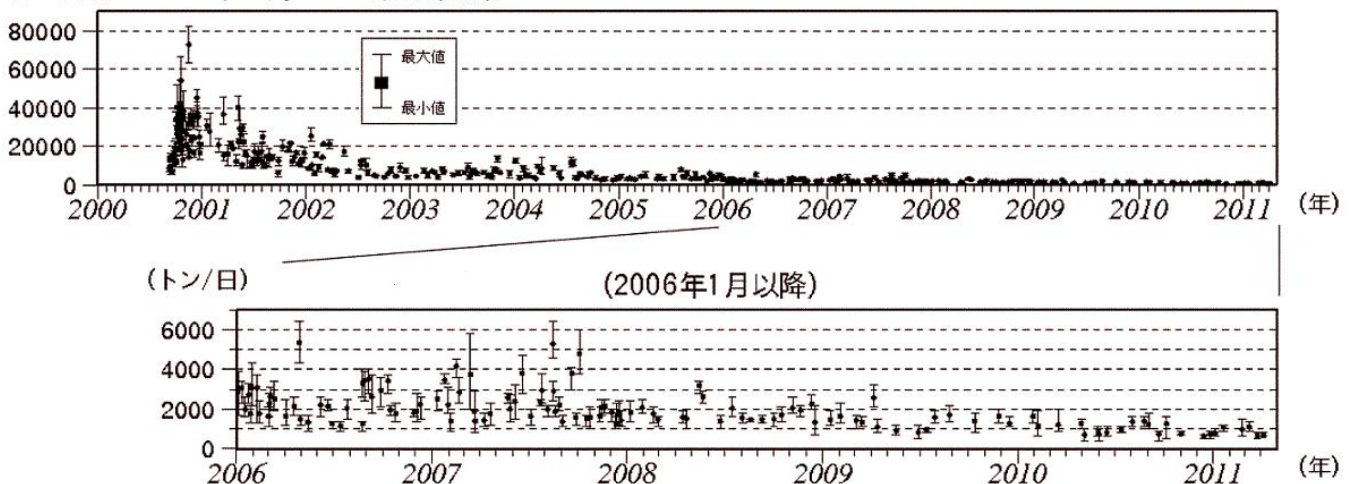
図 2 三宅島 二酸化硫黄の放出量 4) の推移（2000 年 8 月～2011 年 4 月）
