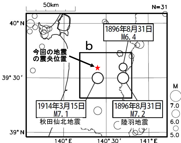
震央分布図 (1885 年 1 月 1 日～2011 年 4 月 30 日 深さ 0～50km M \geq 5.0 ) (1885 年 1 月 1 日～1923 年 7 月 31 日は宇津カタログによる)
