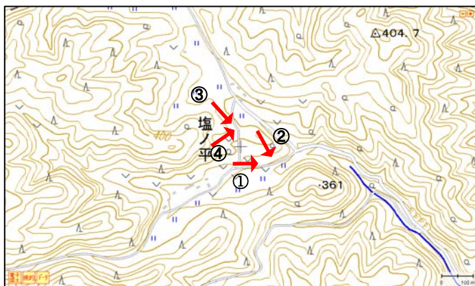
図 3-25 井戸沢断層付近調査地点 (いわき市田人町黒田塩ノ平)
