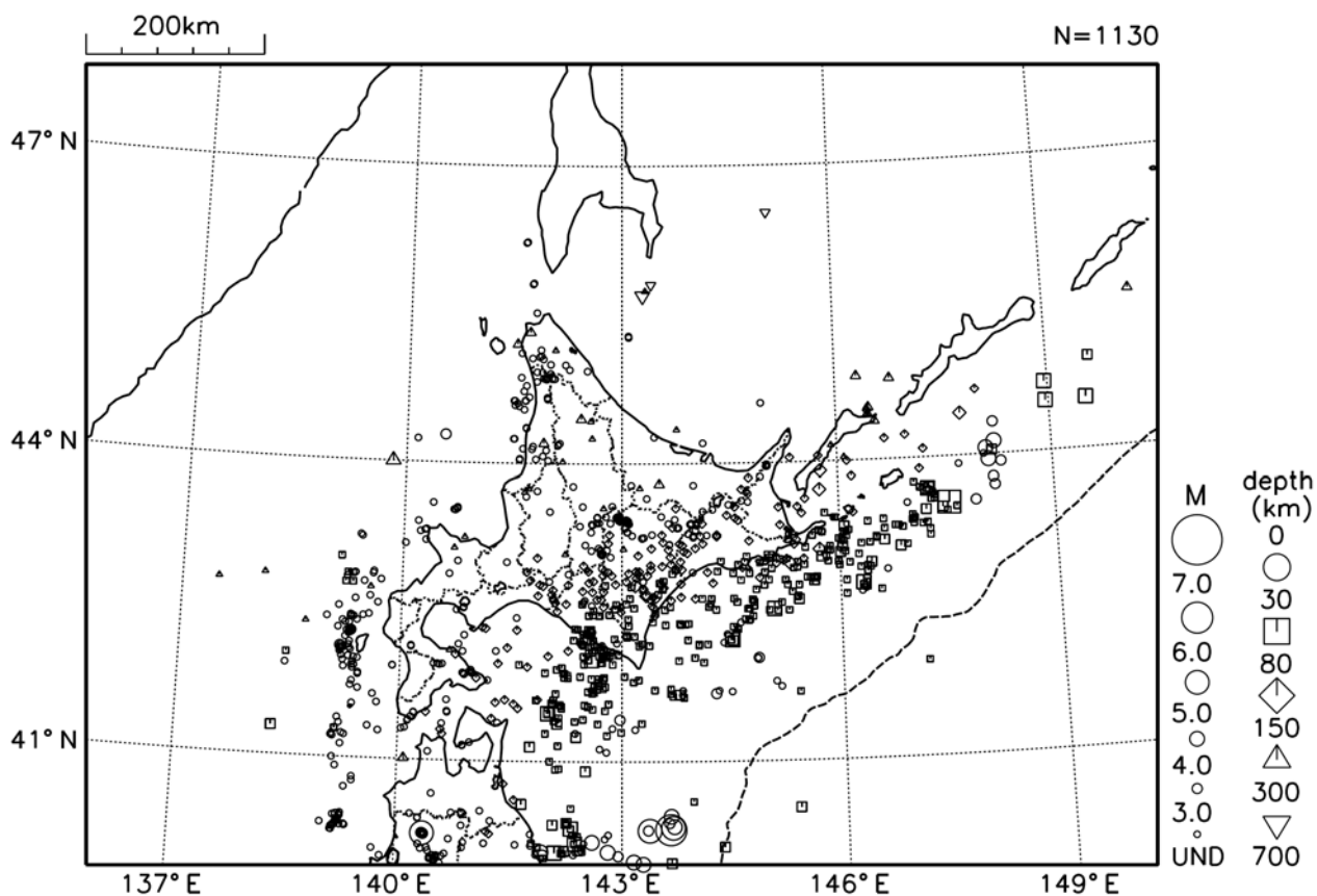
図4 北海道地方の震央分布図（2011年4月1日～4月30日）
