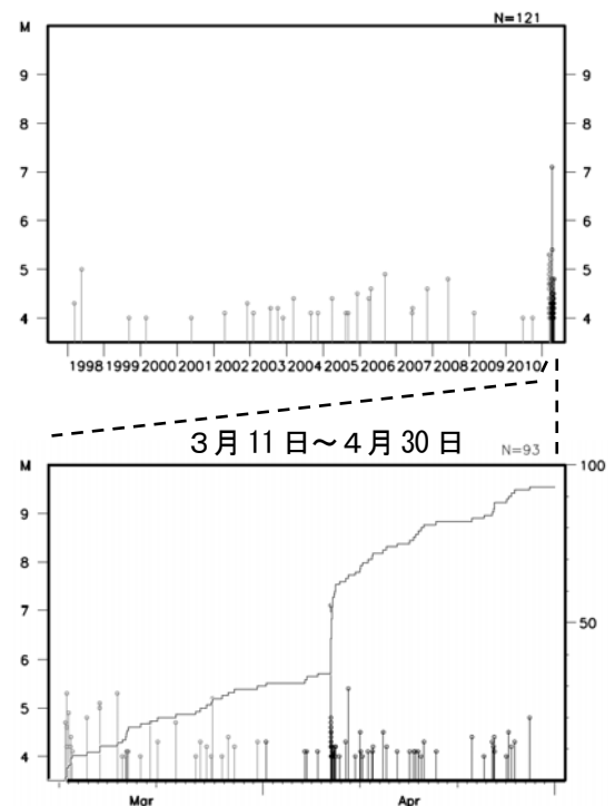
図 2-1-2 領域 b 内の M-T 図及び回数積算図
