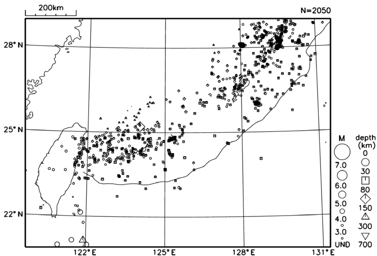
図9 沖縄地方の震央分布図（2011 年 4 月 1 日～ 4 月 30 日）
