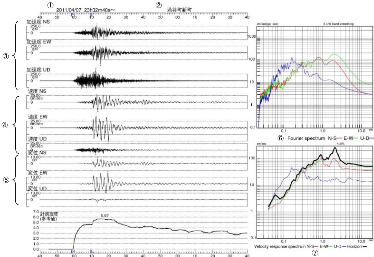
図 2-7 涌谷町新町で観測した波形、加速度フーリエスペクトル及び速度応答スペクトル
