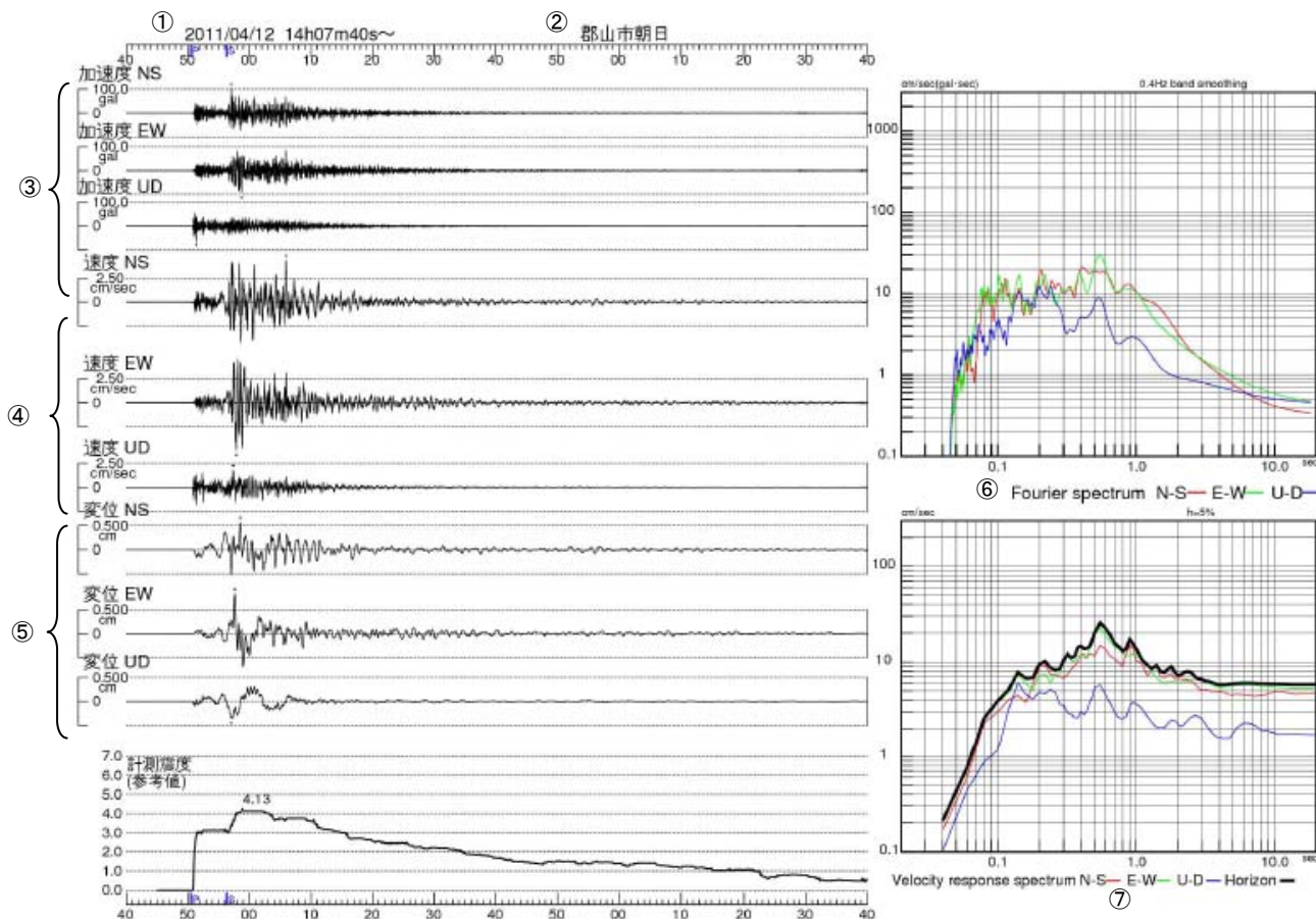
図 3-16 郡山市朝日で観測した波形、加速度フーリエスペクトル及び速度応答スペクトル
