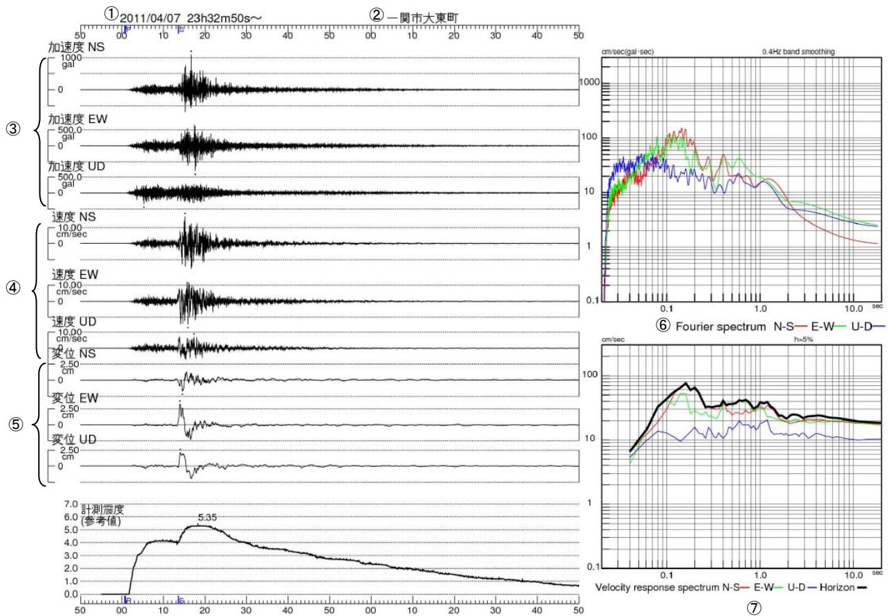
図 2-10 一関市大東町で観測した波形、加速度フーリエスペクトル及び速度応答スペクトル
