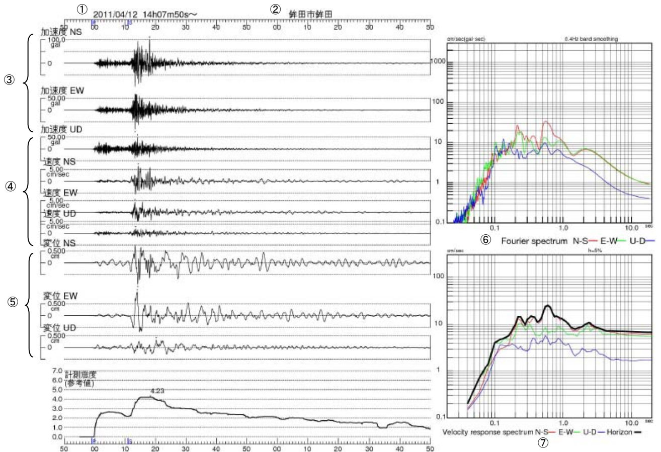
図 3-18 鉾田市鉾田で観測した波形、加速度フーリエスペクトル及び速度応答スペクトル
