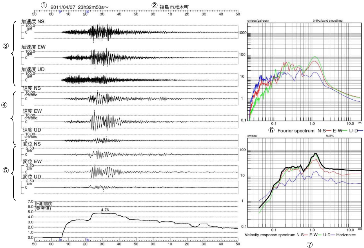
図 2-13 福島市松木町で観測した波形、加速度フーリエスペクトル及び速度応答スペクトル
