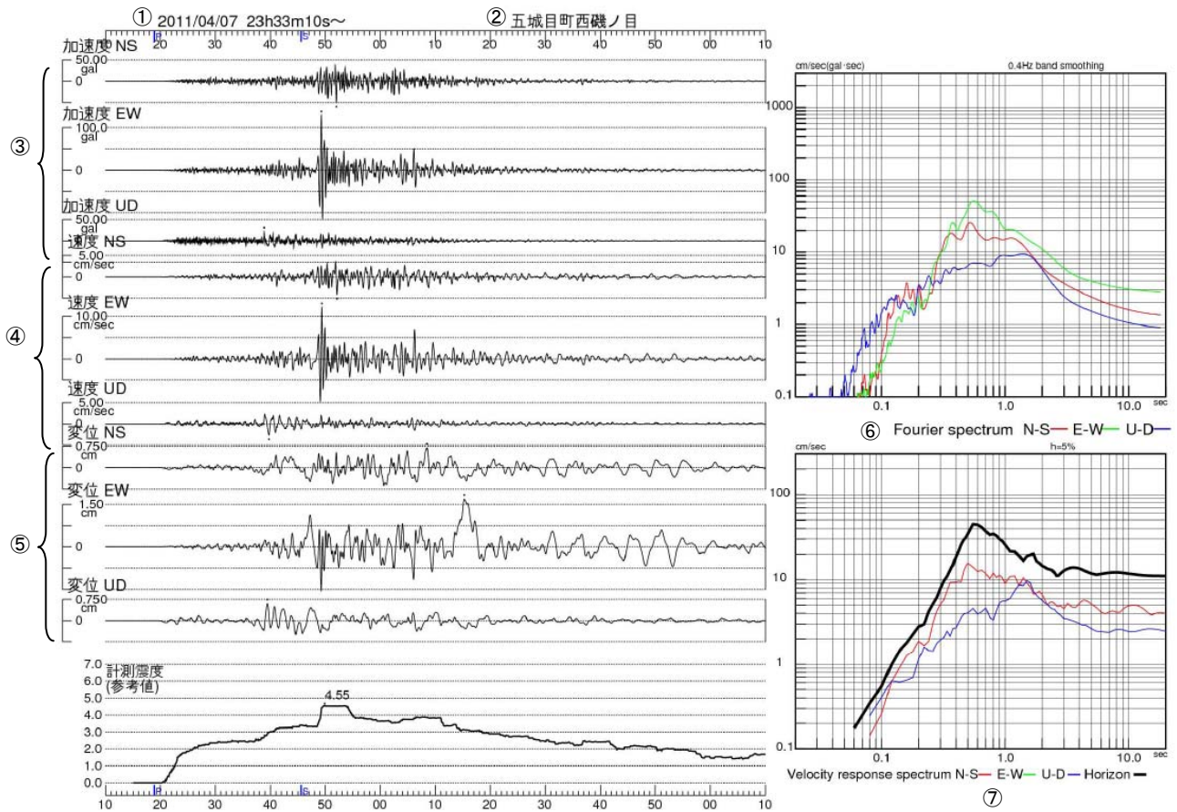
図 2-12 五城目町西磯ノ目で観測した波形、加速度フーリエスペクトル及び速度応答スペクトル
