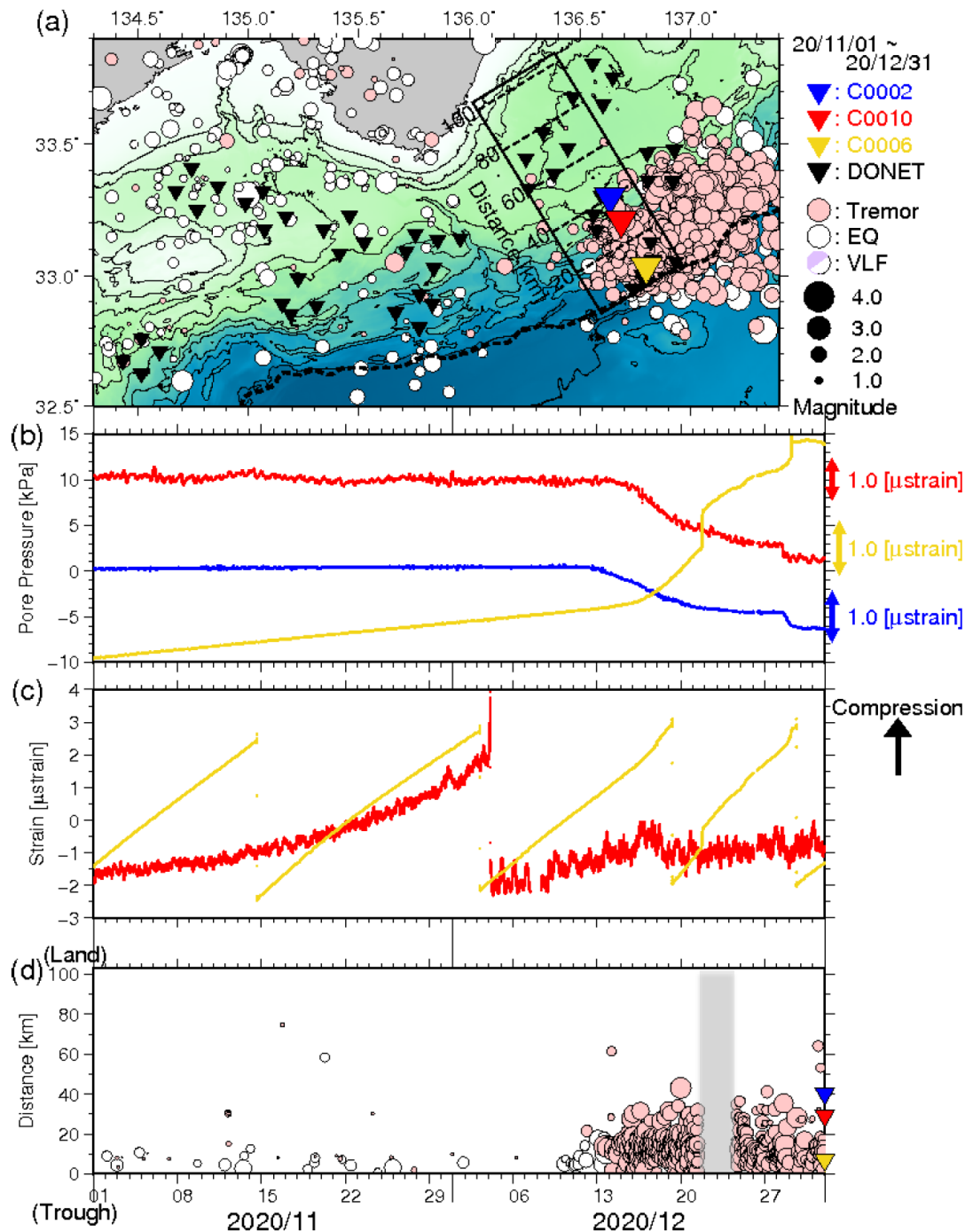
図3 直近2ヶ月間のSSE・低周波微動モニタリング（2020年11月1日～2020年12月31日）。
